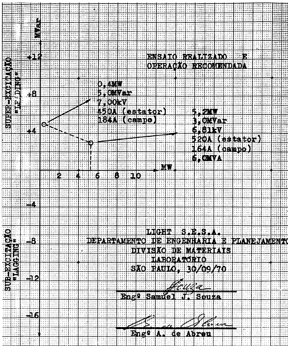
Figura A9 - Gráfico de operação da unidade nº 4 da UEP.
