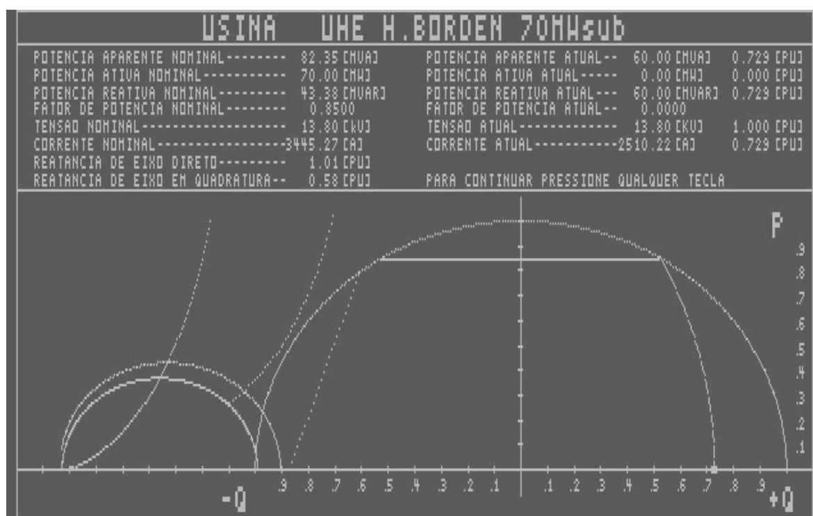
Figura B5 - Curva de capacidade das unidades de 70 MW de UHB.
