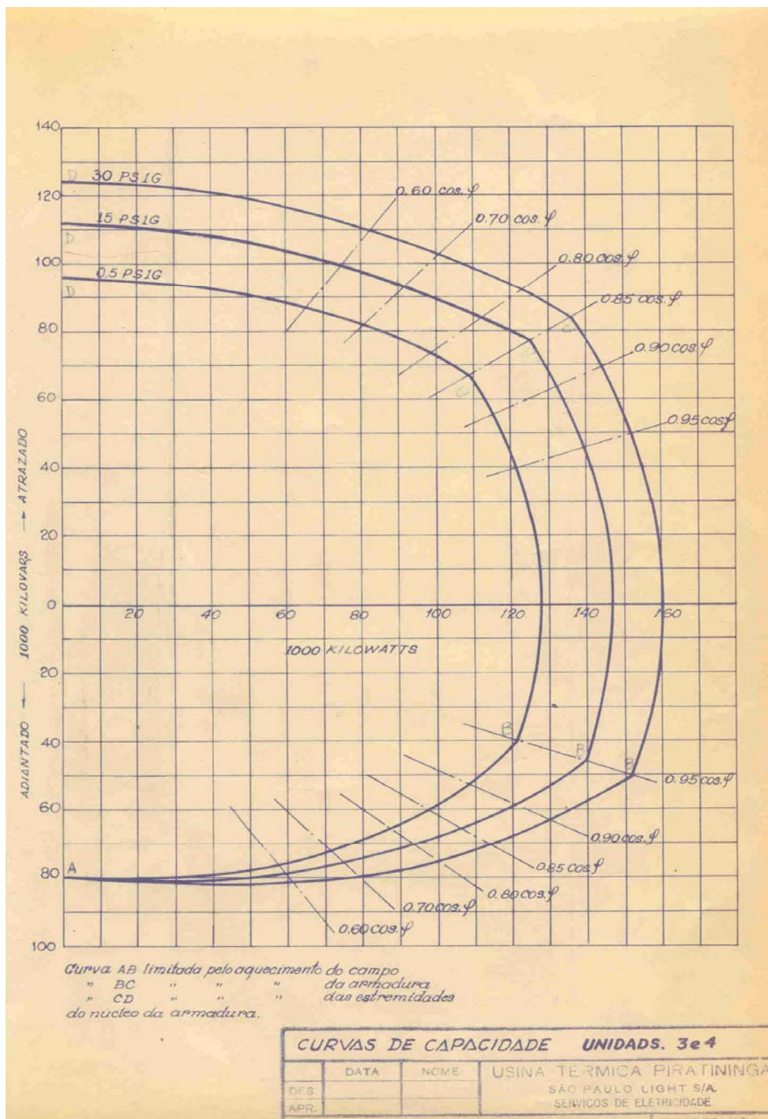
Figura C2 - Curva de capacidade das unidades nº 3 e 4 da Usina Termoelétrica Piratininga.
