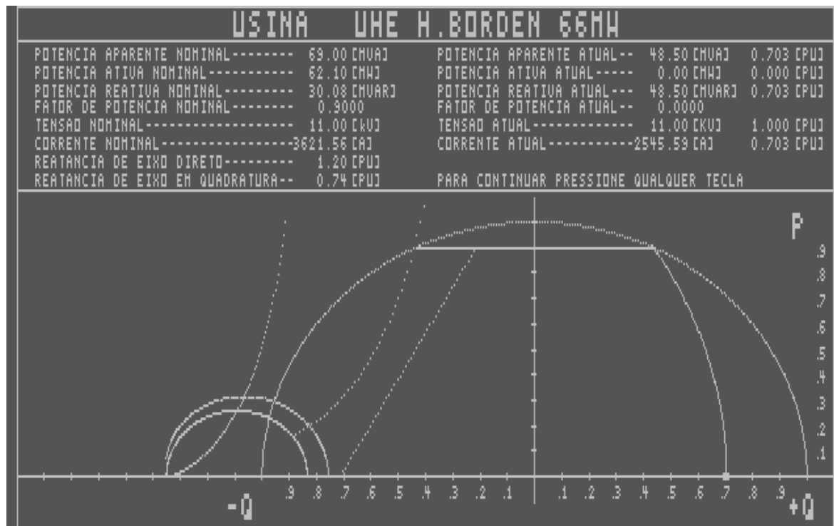
Figura B4 - Curva de capacidade das unidades de 66 MW de UHB
