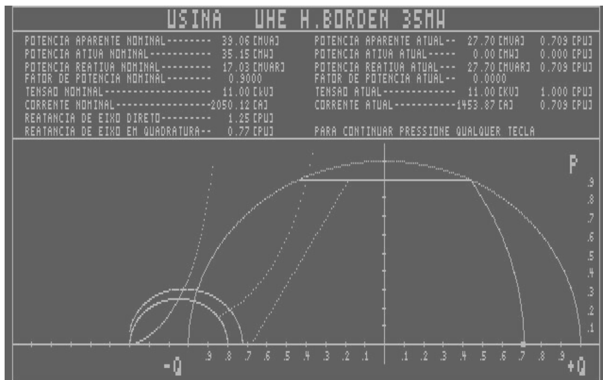
Figura B2 - Curva de capacidade das unidades de 35 MW de UHB.
