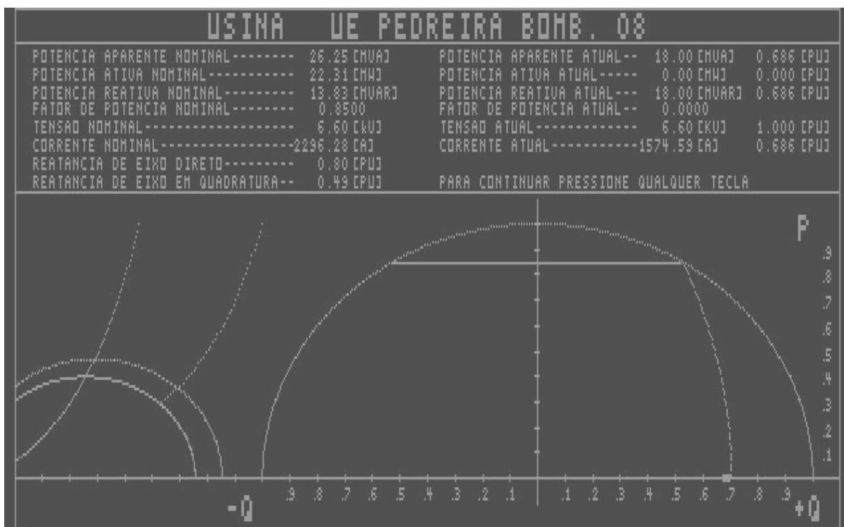
Figura A18 - Curva de capacidade da unidade nº 8 da UEP.
