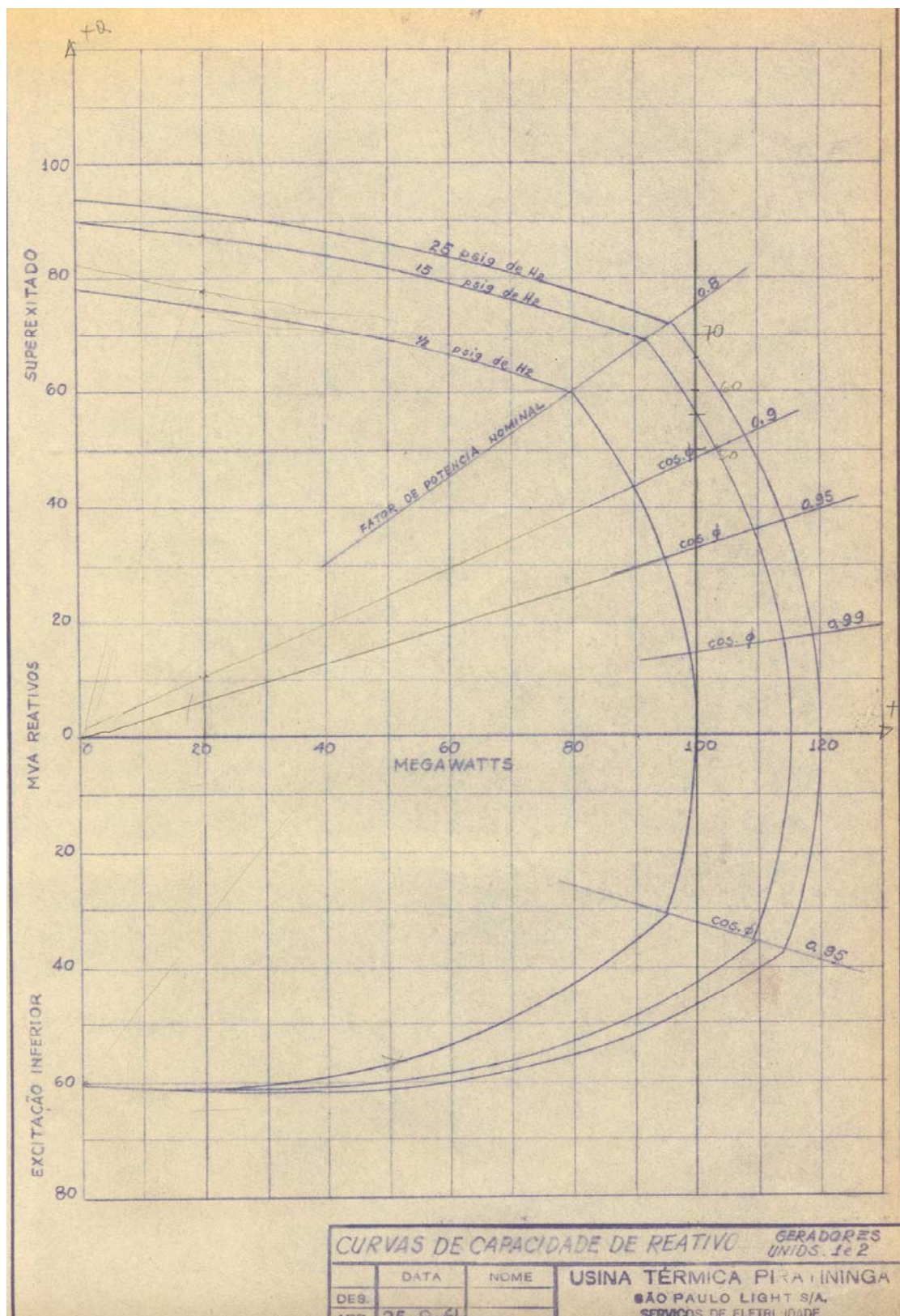
Figura C1 - Curva de capacidade das unidades n° 1 e 2 da Usina Termoeletrica Piratininga.
