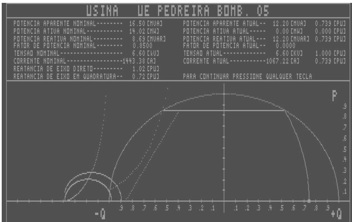
Figura A17 - Curva de capacidade da unidade nº 5 da UEP.
