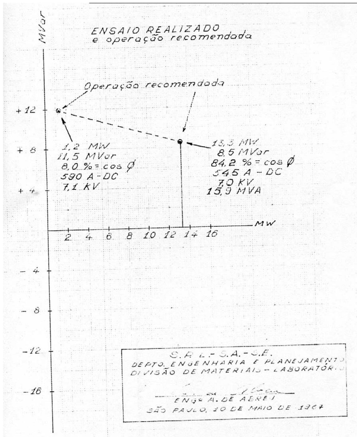
Figura A6 - Gráfico de operação da unidade nº 2 da UEP.
