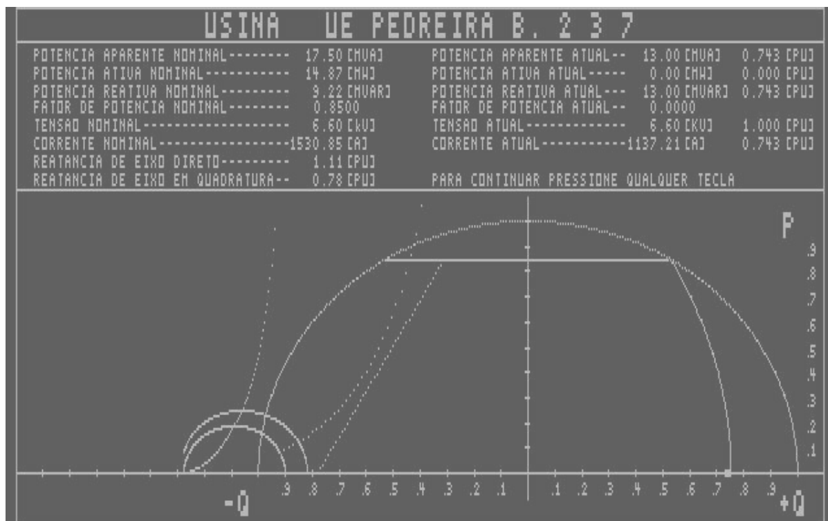
Figura A16 - Curva de capacidade das unidades 2, 3 e 7 da UEP.
