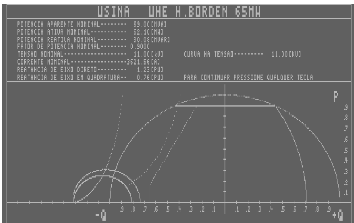
Figura B3 - Curva de capacidade das unidades de 65MW de UHB.
