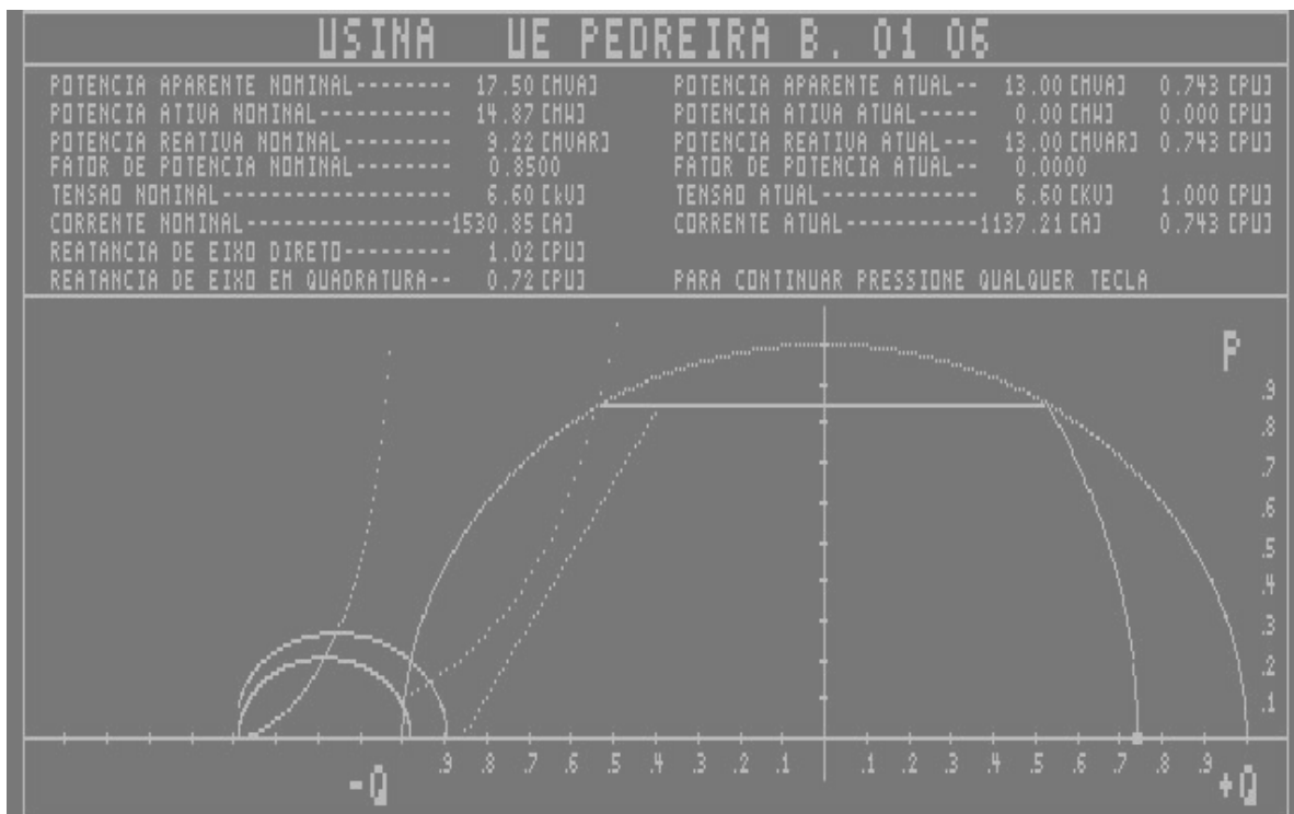
Figura A15 - Curva de capacidade das unidades nº 1 e 6 da UEP.
