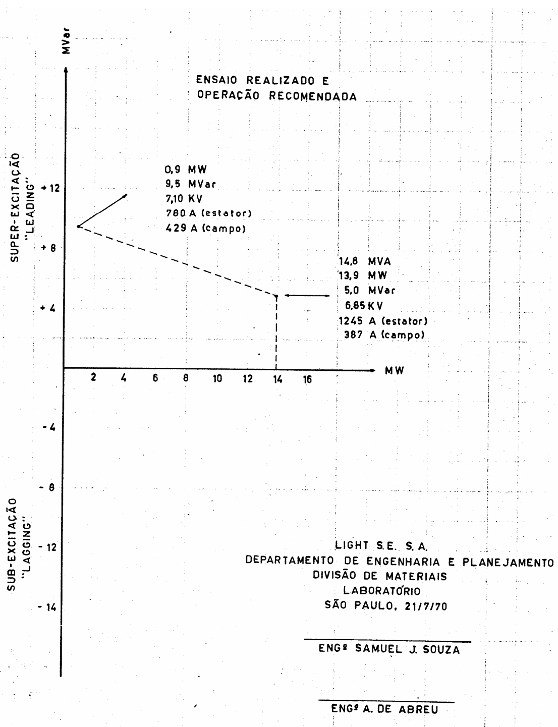
Figura A12 - Gráfico de operação da unidade nº 5 da UEP.
