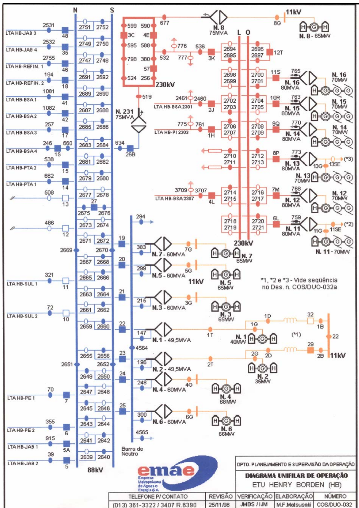
Figura B1 - Diagrama elétrico da ETU Henry Borden.
