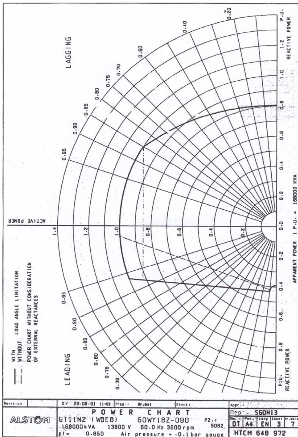
Figura D1 - Curva de capacidade das unidades geradoras da Usina Termoeletrica Nova Piratininga.
