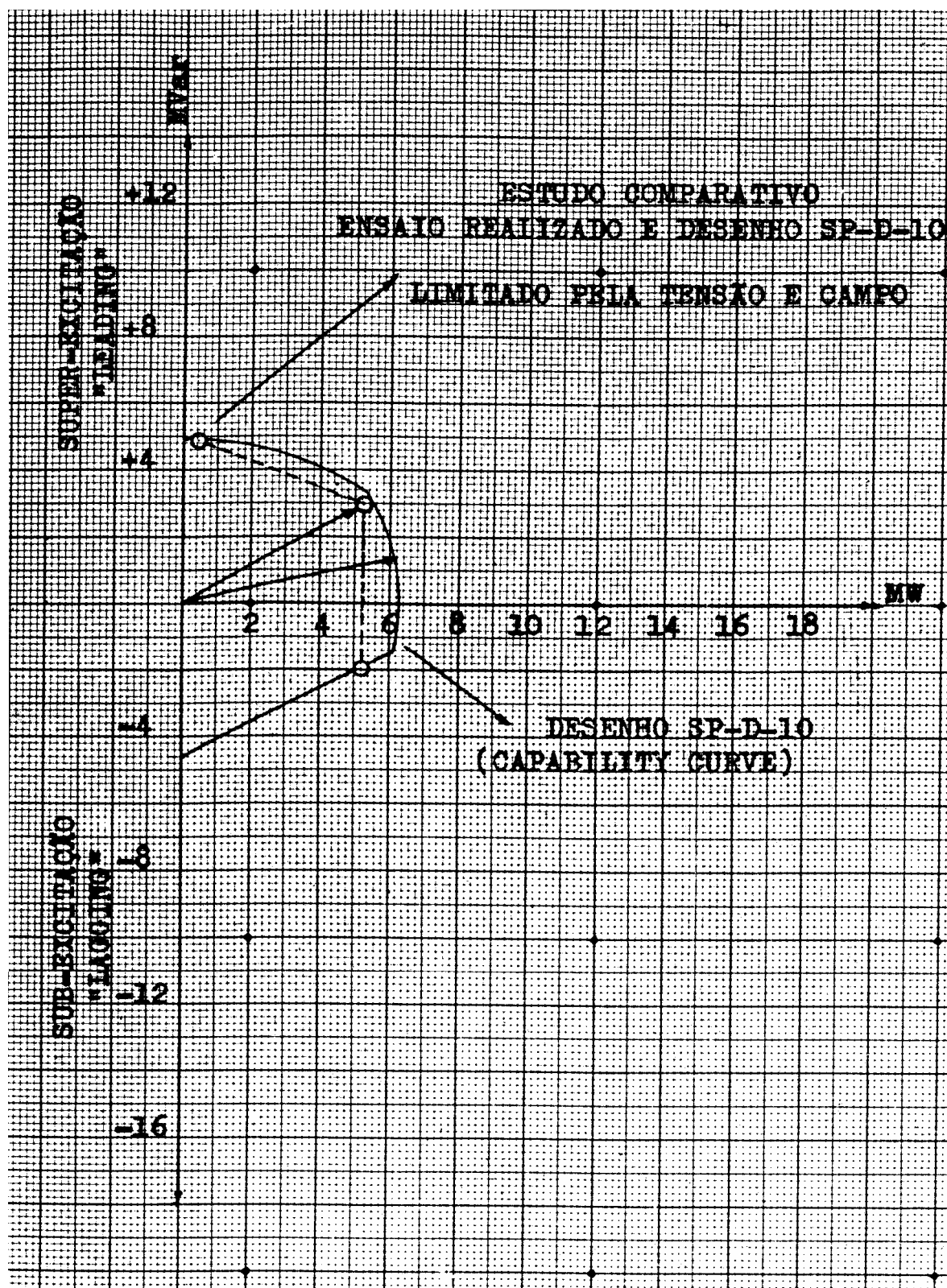
Figura A10 - Curva de operação da unidade nº 4 da UEP.
