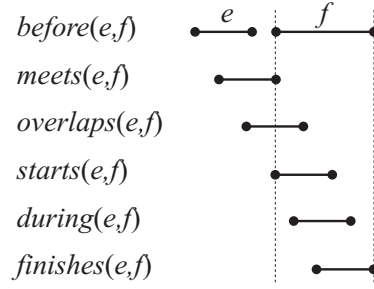
Figura 3.1: Possíveis relacionamentos entre dois intervalos
