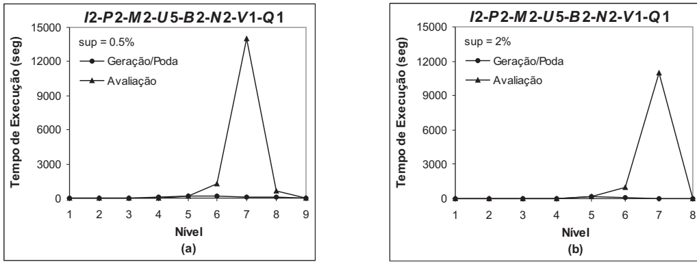
Figura 6.3: Tempo de execução de cada etapa em cada nível
