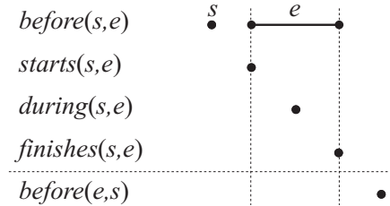
Figura 3.3: Possíveis relacionamentos entre um ponto e um intervalo (acima da linha pontilhada), e entre um intervalo e um ponto (abaixo da linha pontilhada)
