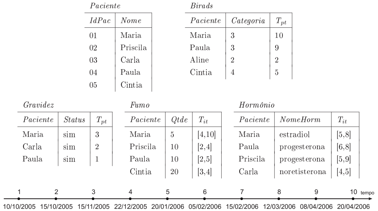
Figura 1.1: Exemplo de um banco de dados de uma clínica de mamografia
