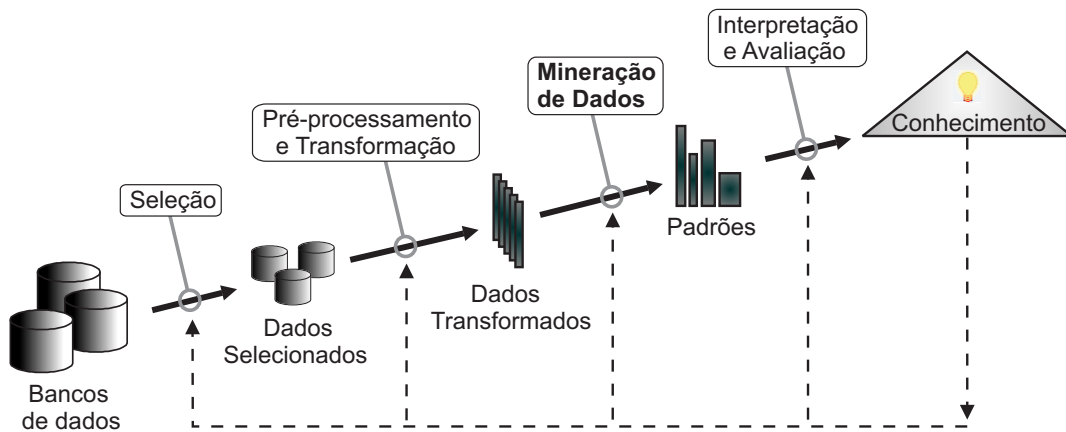
Figura 2.1: Passos do KDD ( adaptação de [1] )
