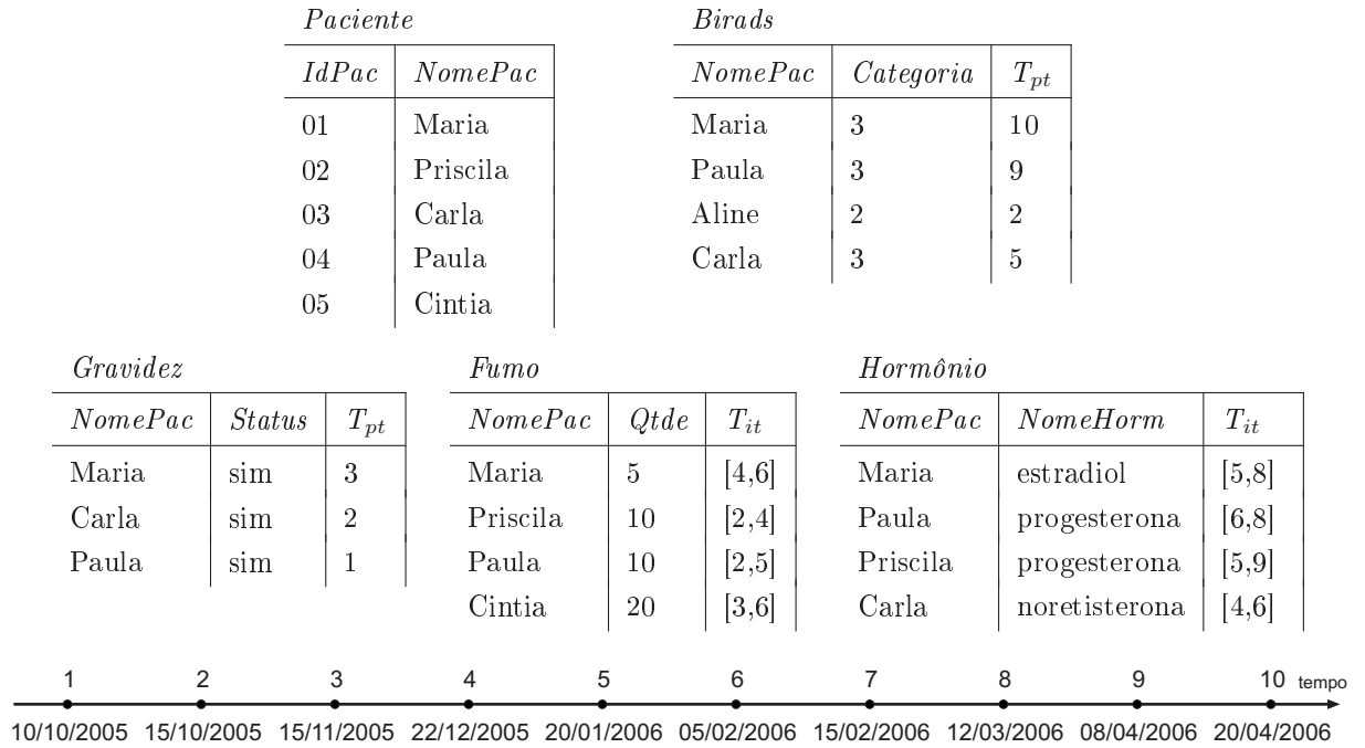
Figura 3.4: Exemplo de um banco de dados de pacientes e de um mapeamento em datas
