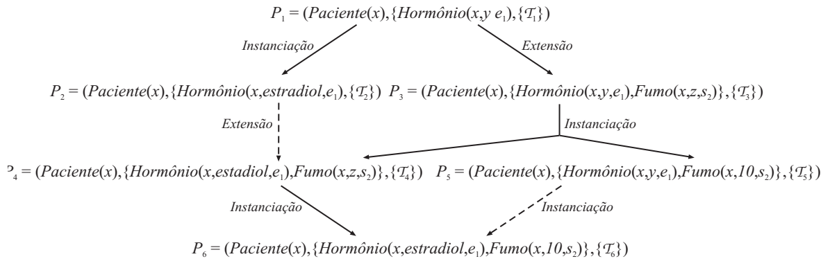
Figura 4.1: Exemplo de dois pth's P_4 e P_6 obtidos a partir de pth's não equivalentes
