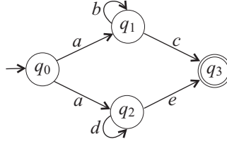
Figura 2.2: Autômato A_{\mathcal{R}} associado a uma expressão regular \mathcal{R}
