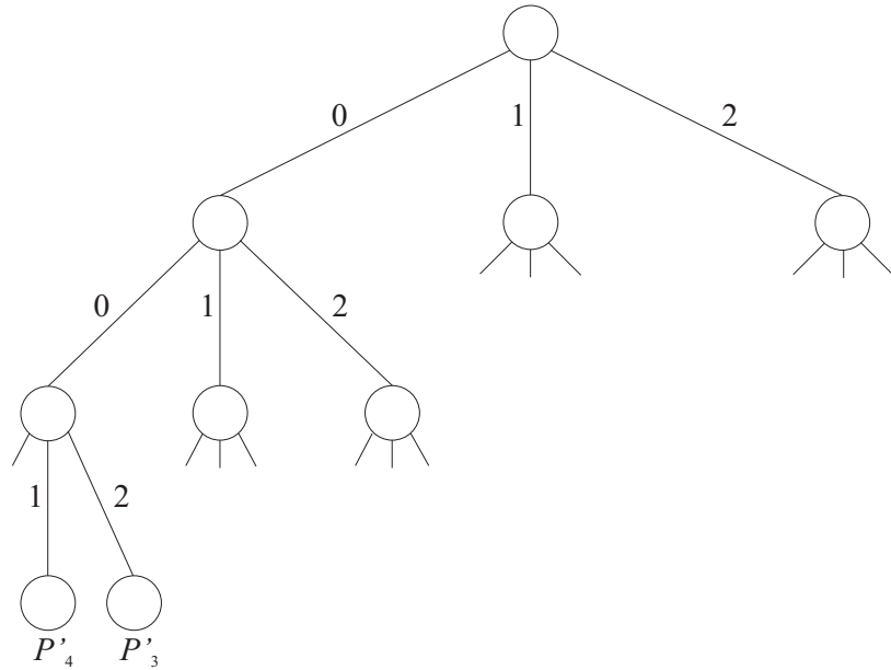
Figura 5.14: Árvore hash após a inserção dos pth's
