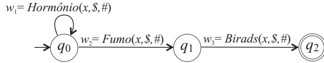
Figura 5.8: Autômato \mathcal{A}_R associado a expressão regular \mathcal{R}
