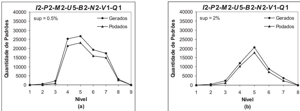
Figura 6.2: Relação entre a quantidade de pth's gerados e podados
