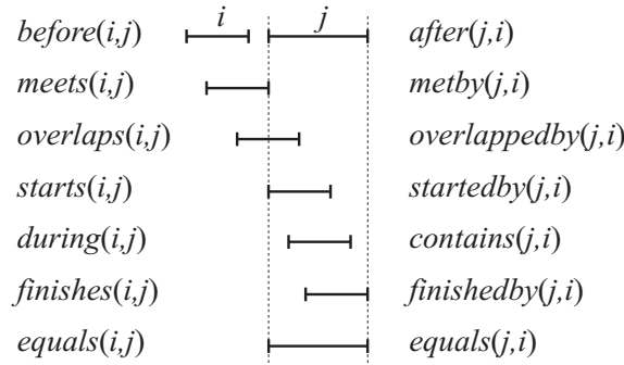
Figura 2.5: Possíveis relacionamentos entre dois intervalos ( adaptação de [2] )
