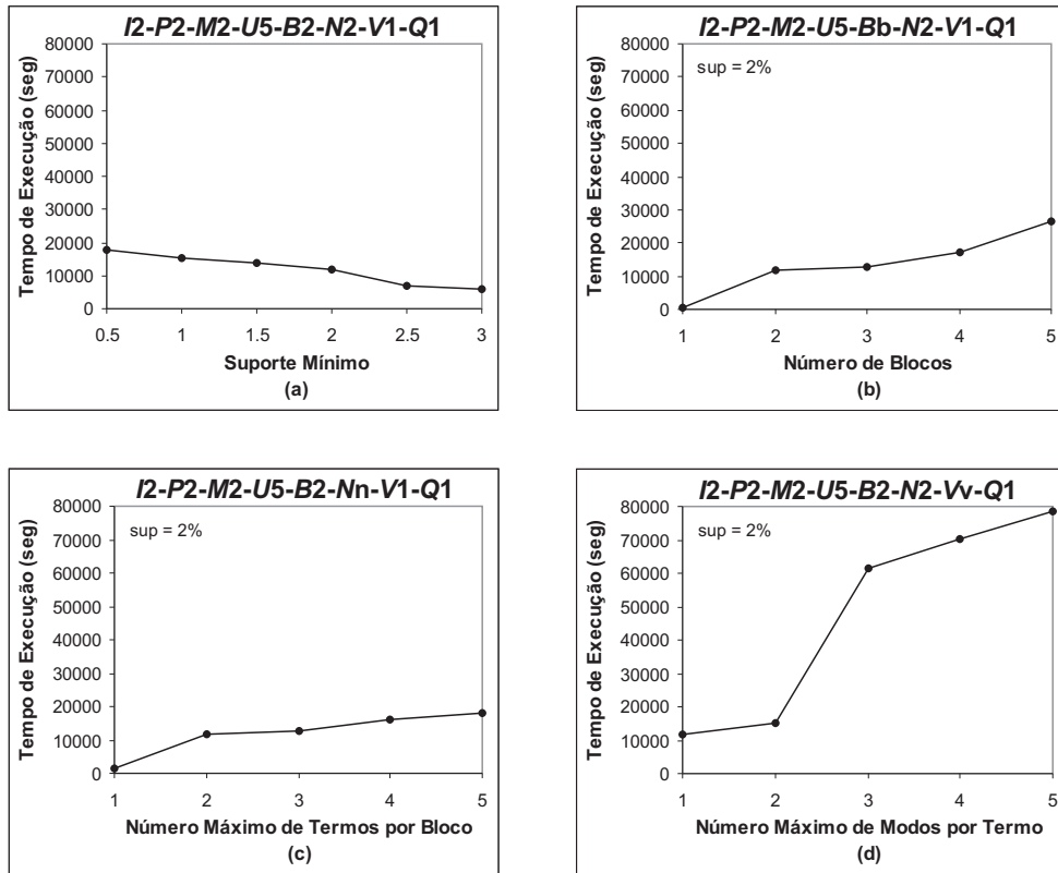
Figura 6.1: Análise de performance variando alguns parâmetros
