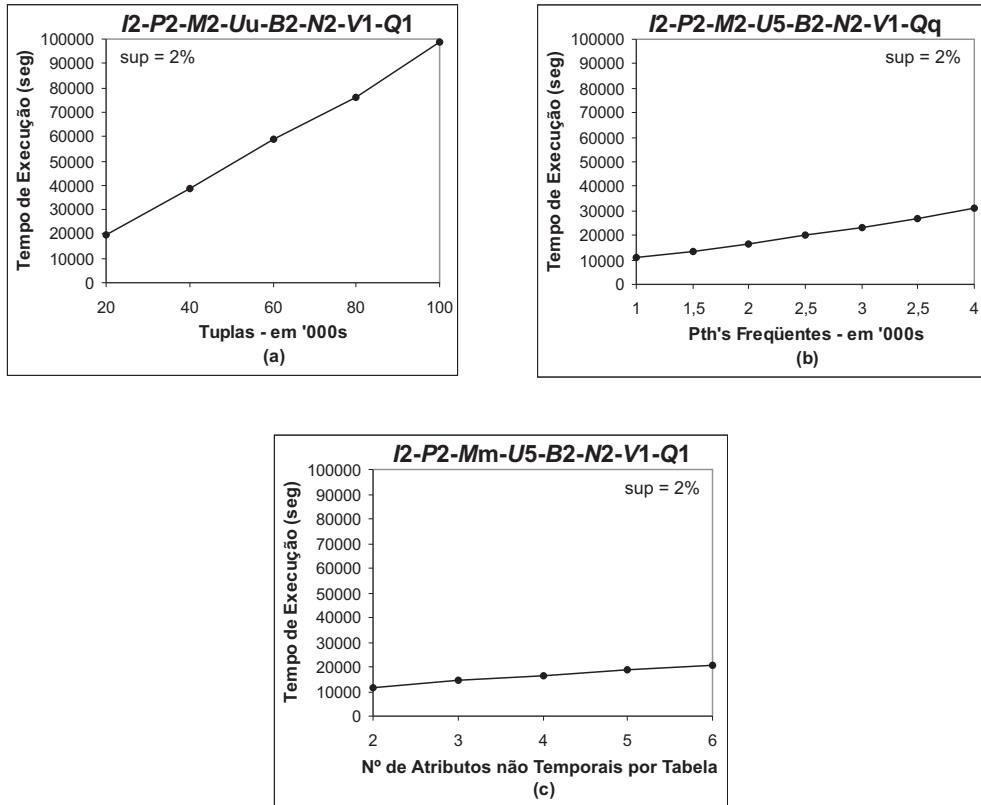
Figura 6.4: Análise de escalabilidade variando alguns parâmetros
