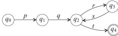
Figura 2.4: Autômato A_{\mathcal{R}} .
