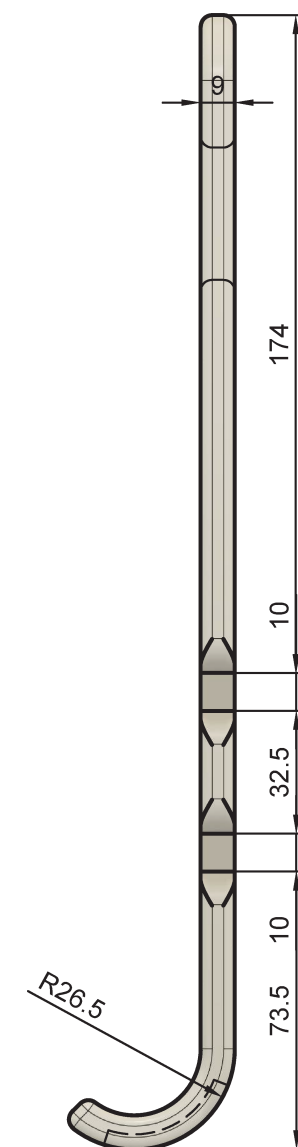
PEÇA 2 PLANO INCLINADO VISTA LATERAL ESC. 1/2
