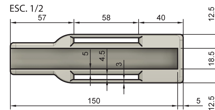
ACESSÓRIO PARA TRANSPORTE VISTA SUPERIOR ESC. 1/2
