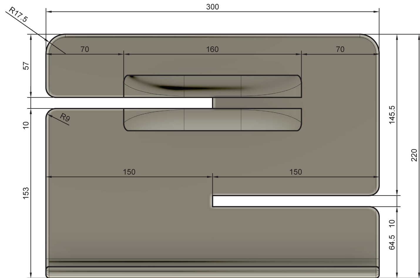
PEÇA 1 PLANO INCLINADO VISTA FRONTAL ESC. 1/2
