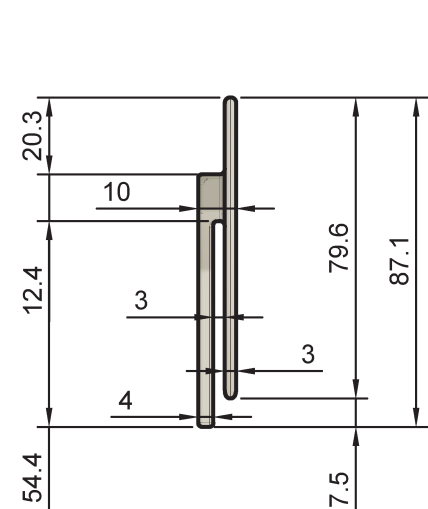
CLIPE PARA LIVRO VISTA LATERAL ESC. 1/2
