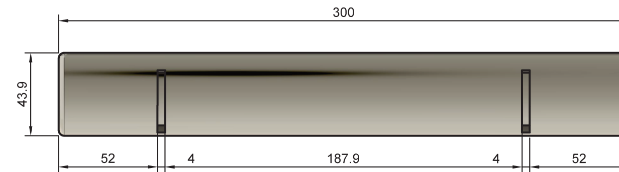
PEÇA 1 PLANO INCLINADO VISTA SUPERIOR ESC. 1/2
