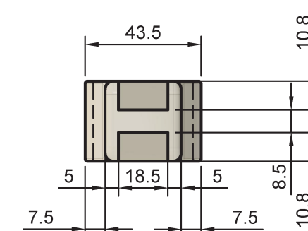
ACESSÓRIO PARA TRANSPORTE VISTA LATERAL ESC. 1/2
