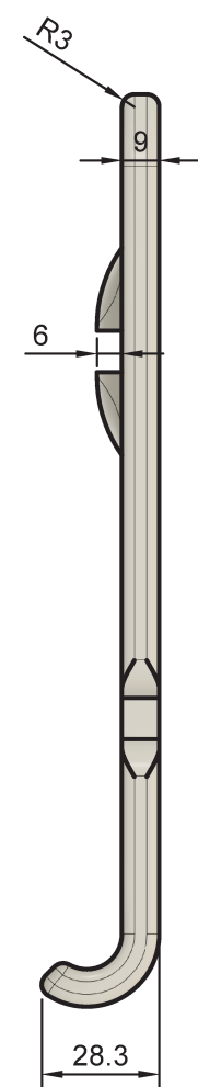
PEÇA 1 PLANO INCLINADO VISTA LATERAL ESC. 1/2
