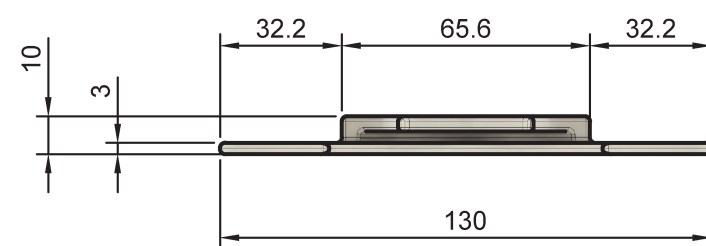
CLIPE PARA LIVRO VISTA POSTERIOR ESC. 1/2
