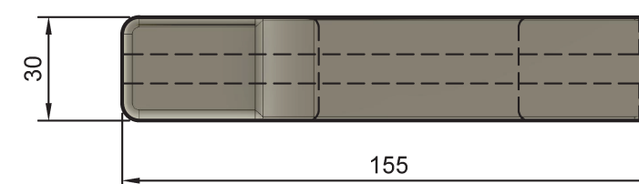
ACESSÓRIO PARA TRANSPORTE VISTA FRONTAL ESC. 1/2
