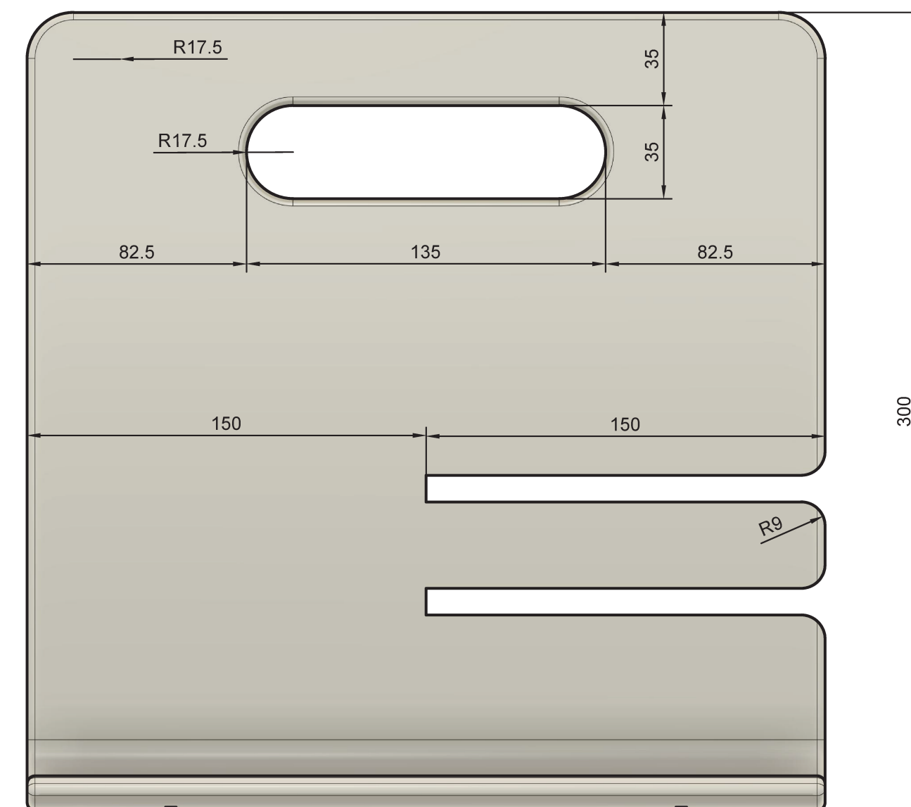
PEÇA 2 PLANO INCLINADO VISTA FRONTAL ESC. 1/2
