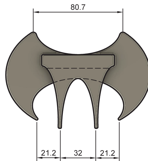
CLIPE PARA LIVRO VISTA POSTERIOR ESC. 1/2
