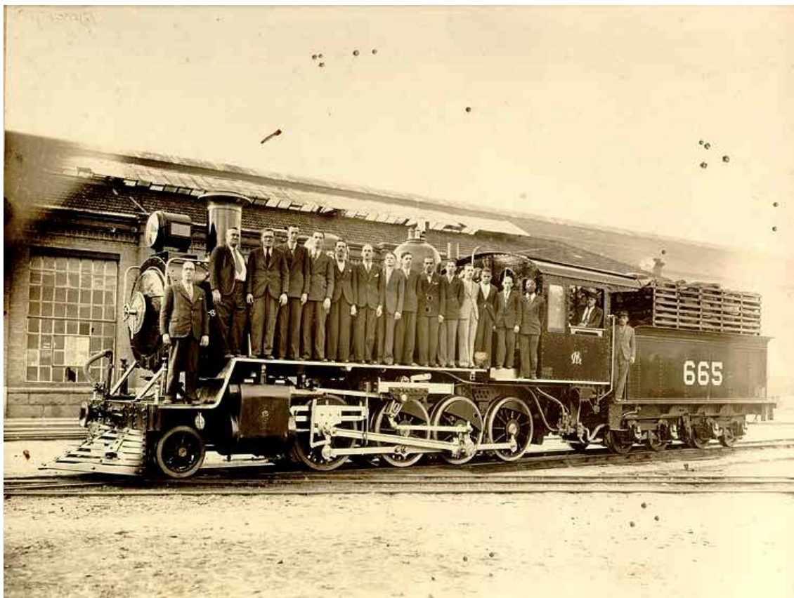
Entrega oficial da 665 tipo Consolidation, fabricada pela CM, com esforço de tração de 11.465 kg à 85% de pressão na caldeira. (Foto do acervo do Museu da CP - Jundiaí) Fonte: http://www.cmef.com.br/ acesso dia 10 de março de 2011 9 horas.
