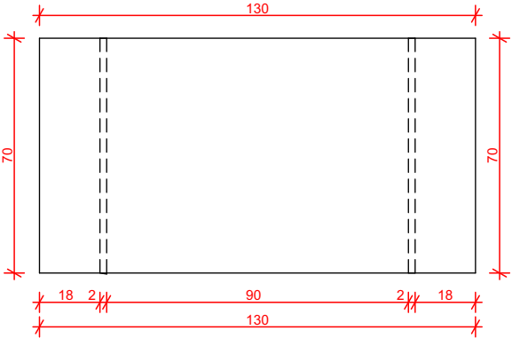
3. Peça 01 Escala: 1:20
