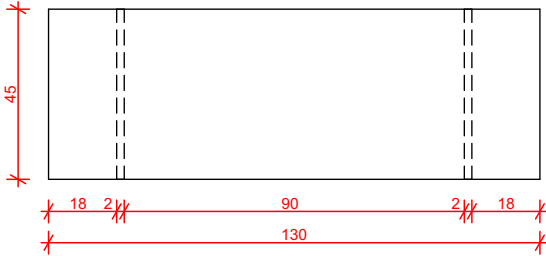
5. Peça 03 Escala: 1:20
