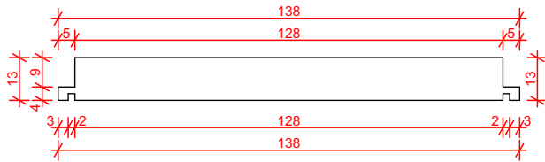
2. Trava 02 Escala: 1:20
