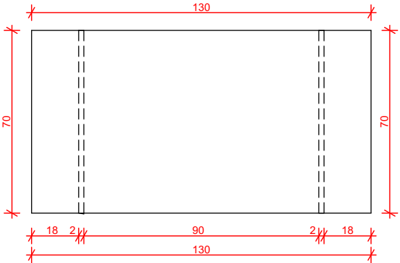
5. Peça 04 Escala: 1:20
