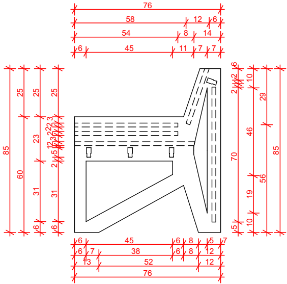
4. Peça 02 Escala: 1:20
