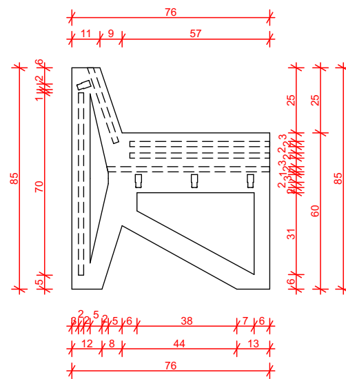
3. Peça 01 Escala: 1:20
