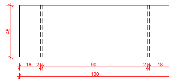
5. Peça 03 Escala: 1:20
