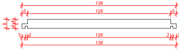
1. Trava 01 Escala: 1:20
