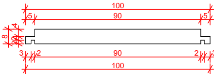
5. Trava 5 Escala: 1:20
