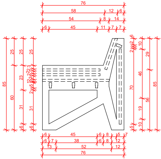
4. Peça 02 Escala: 1:20
