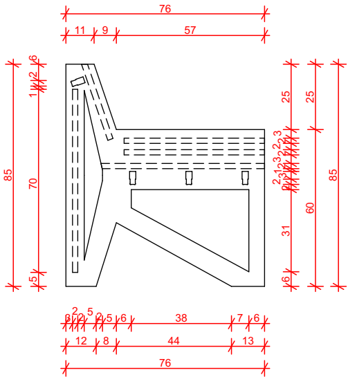
3. Peça 01 Escala: 1:20
