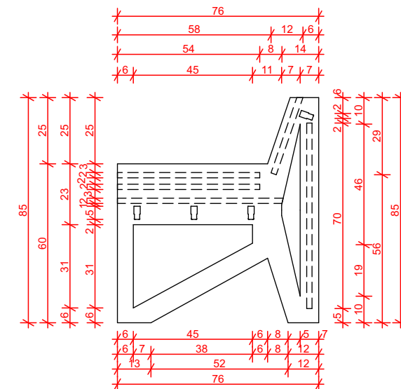
4. Peça 02 Escala: 1:20
