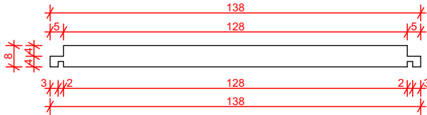
Trava 01 Escala: 1:20
