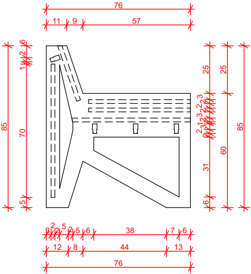
3. Peça 01 Escala: 1:20
