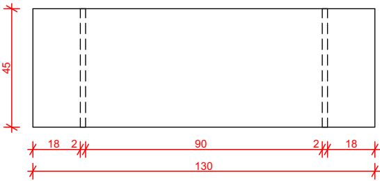
5. Peça 03 Escala: 1:20
