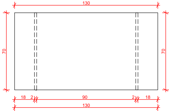
6. Peça 04 Escala: 1:20
