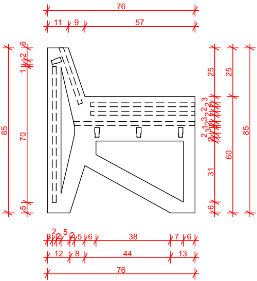
3. Peça 01 Escala: 1:20
