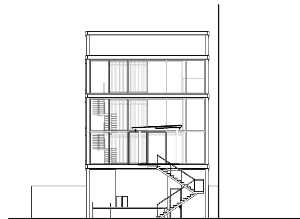
FACHADA PRINCIPAL ANEXO
