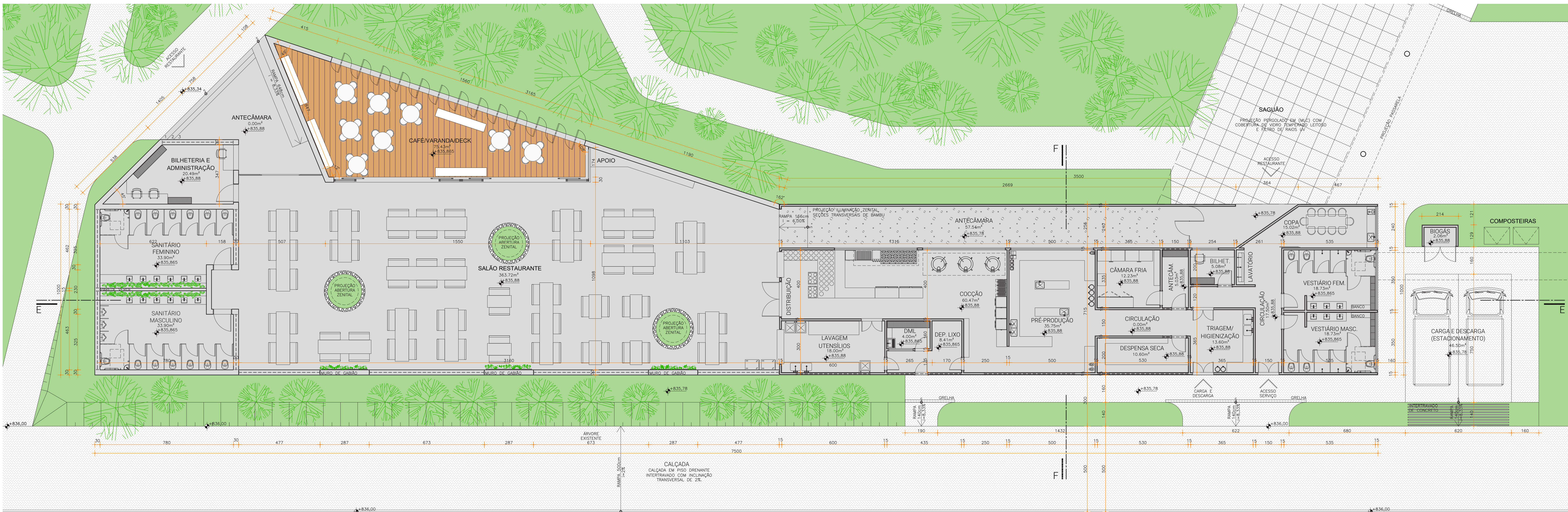
PLANTA TÉRREO 1:100
