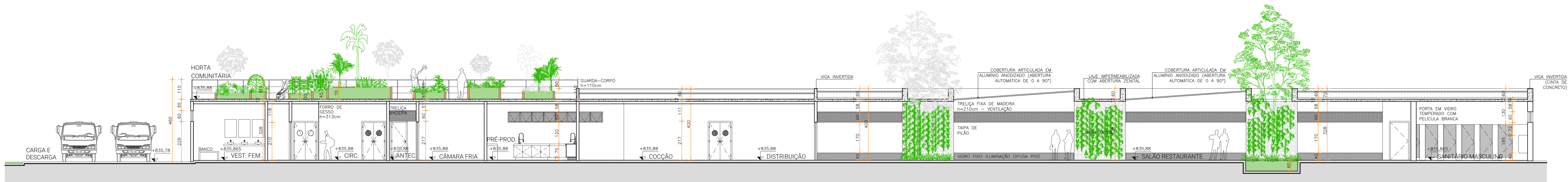
CORTE EE 1:100
