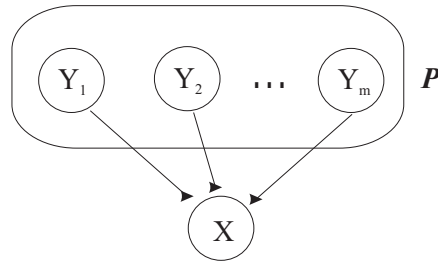
Fig. 5.1: Nós pais de um nó em uma rede bayesiana
