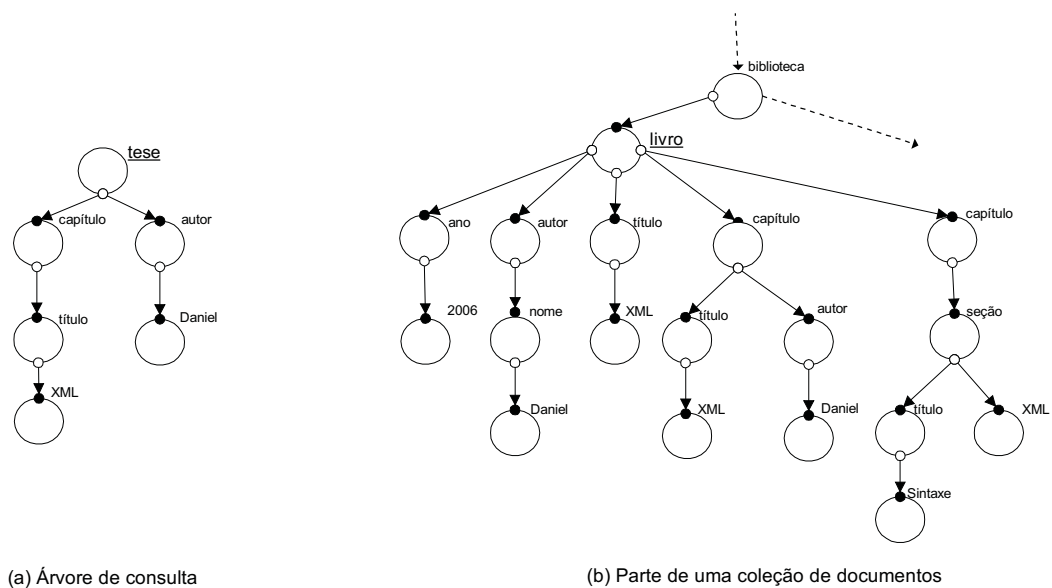
Fig. 5.12: Árvores de consulta e dados
