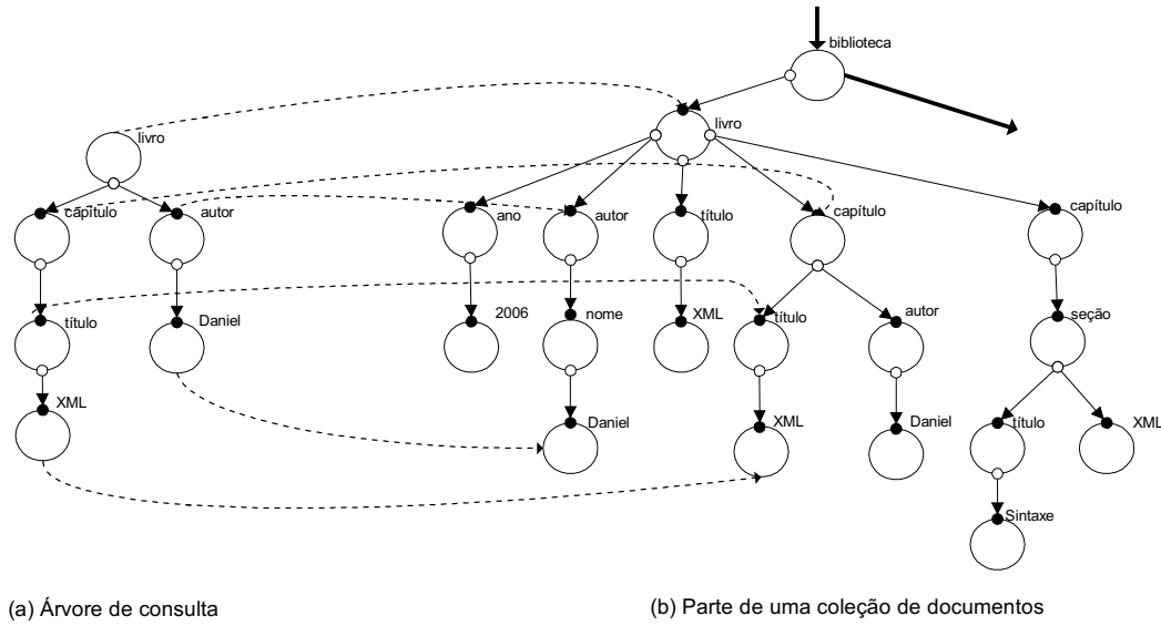
Fig. 5.9: Correlação entre uma árvore de consulta e uma árvore de dados
