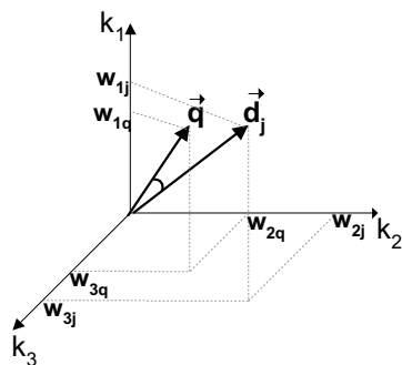
Fig. 4.1: Exemplo dos vetores documento e consulta no espaço vetorial tridimensional ( t = 3 )
