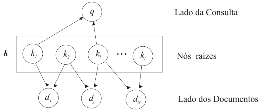
Fig. 5.3: Rede bayesiana para uma consulta q composta pelos termos k_1 e k_i
