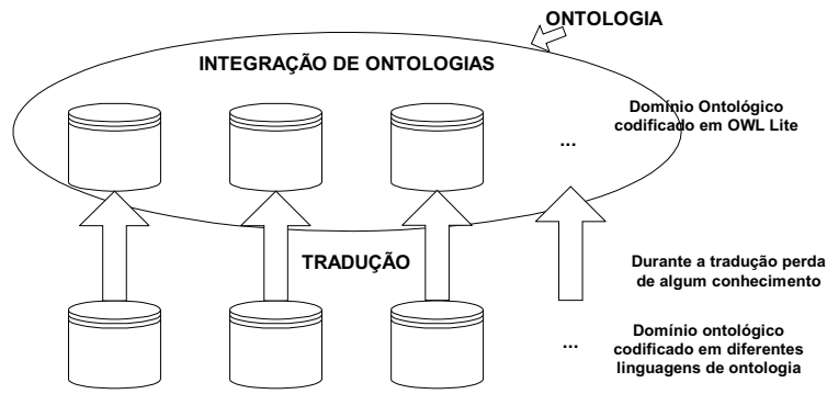
Fig. 5.7: Tradução e integração de ontologias
