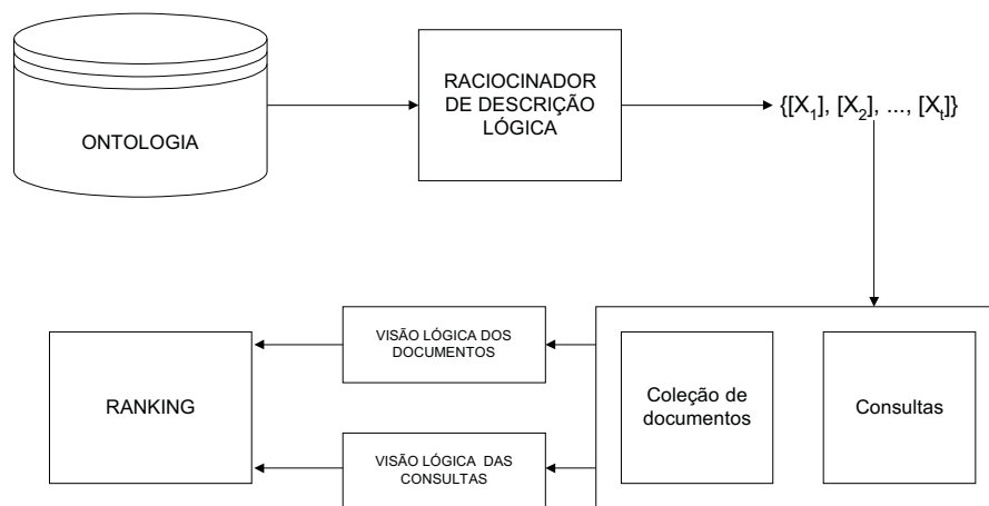
Fig. 5.6: Principais partes do modelo de RI baseado em Ontologia para a Web semântica.
