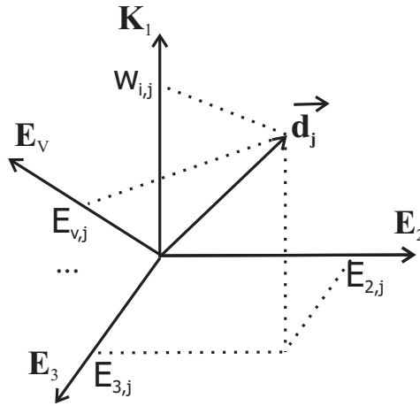
Fig. 5.5: Modelo genérico vetorial para combinação de múltiplas fontes de evidências
