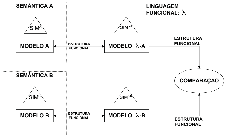
Fig. 3.1: Esquema geral para comparação de equivalência entre modelos de RI
