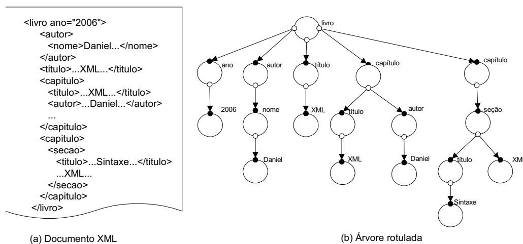
Fig. 5.8: Mapeamento de um documento XML para um árvore rotulada
