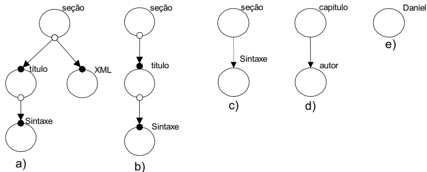
Fig. 5.10: Exemplos de termos complexos
