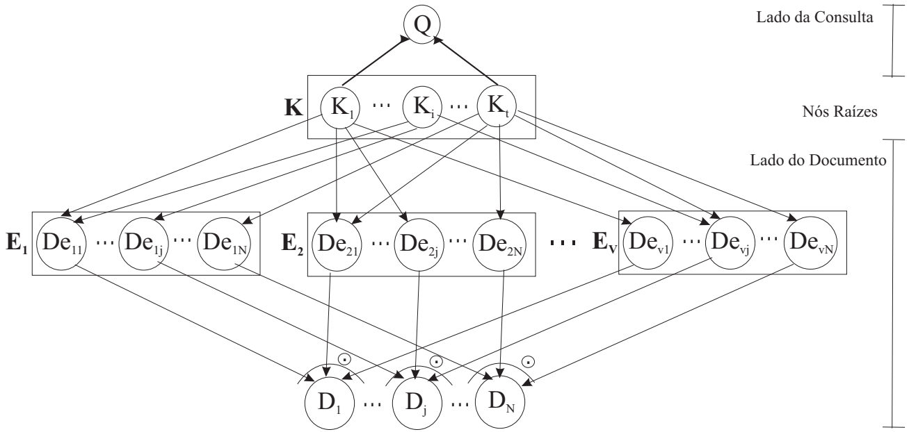
Fig. 5.4: Modelo de rede de crença para combinar múltiplas fontes de evidências
