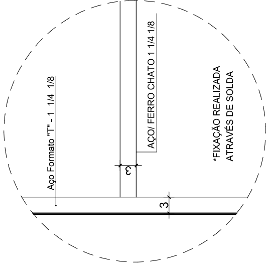
ENCAIXE DETALHE 02 ESC. 1:05
