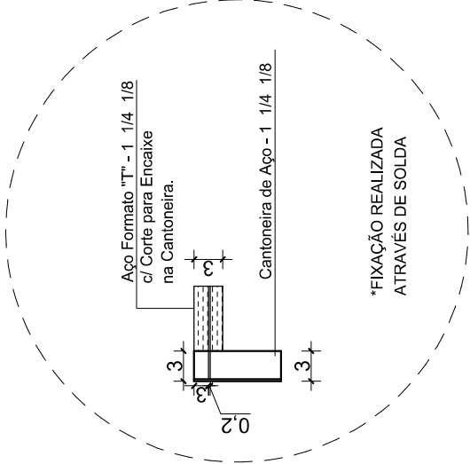
ENCAIXE DETALHE 01 ESC. 1:05
