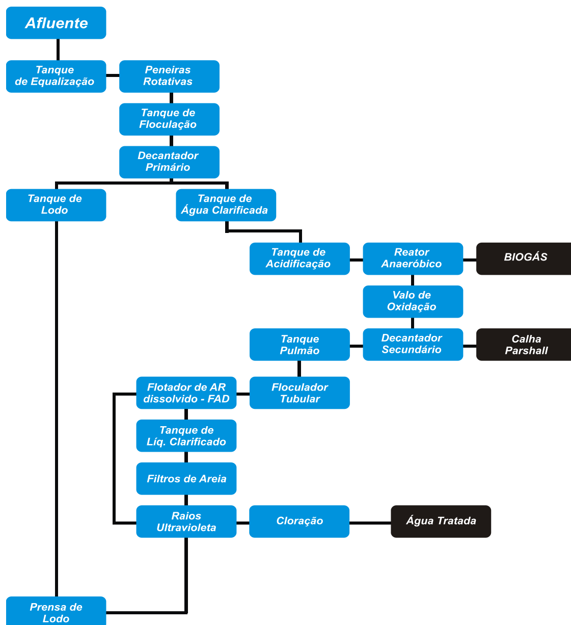
Figura 67 - Etapas da ETE da Souza Cruz, 2008. Adaptado de Souza (2005). Organização: Clóvis Cruvinel, 2009.
