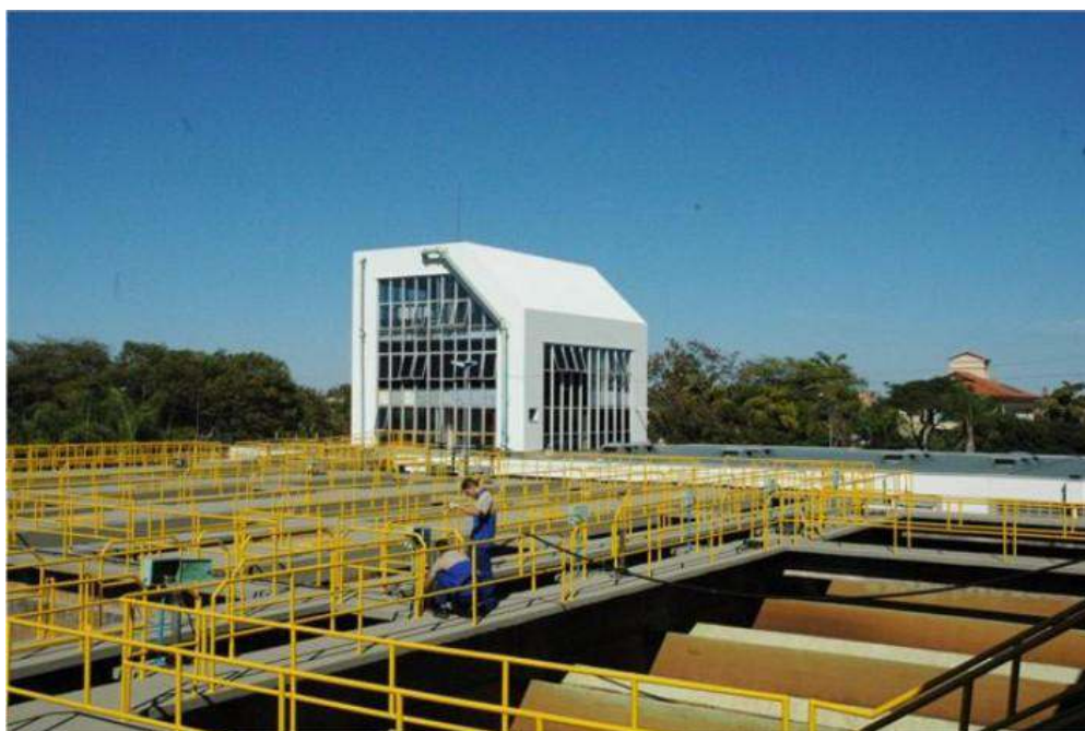
FIGURA 8 - Uberlândia: vista parcial da ETA Bom Jardim. Foto: DMAE, 2008.
