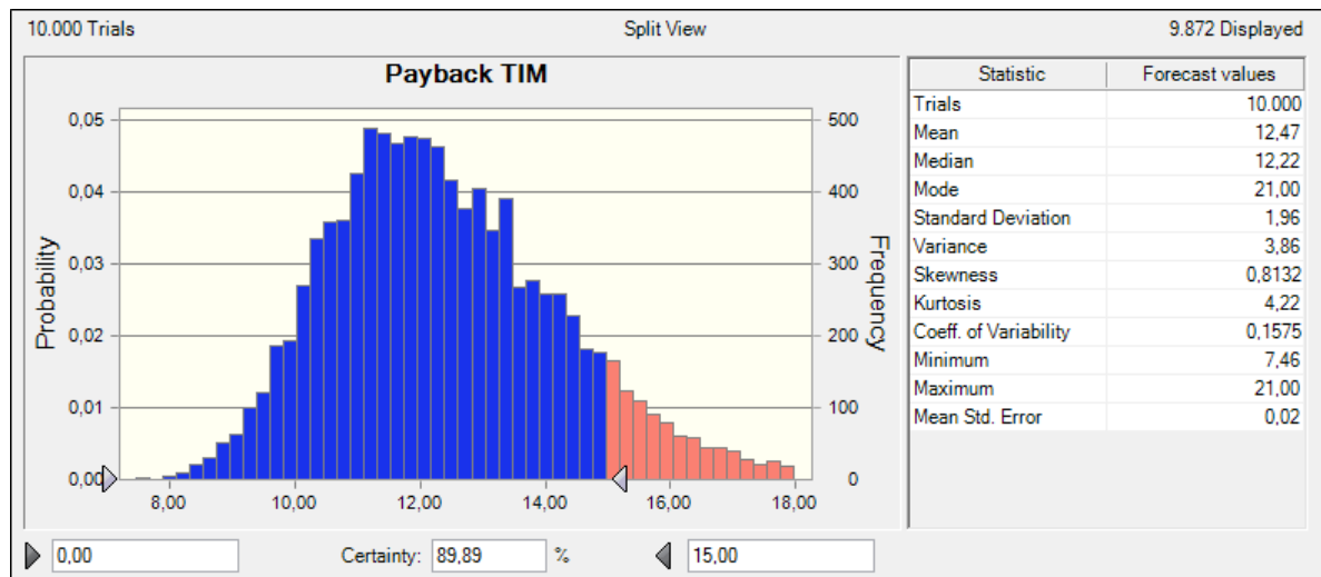
Figura 23: Distribuição de probabilidade do período de payback para a empresa TIM
