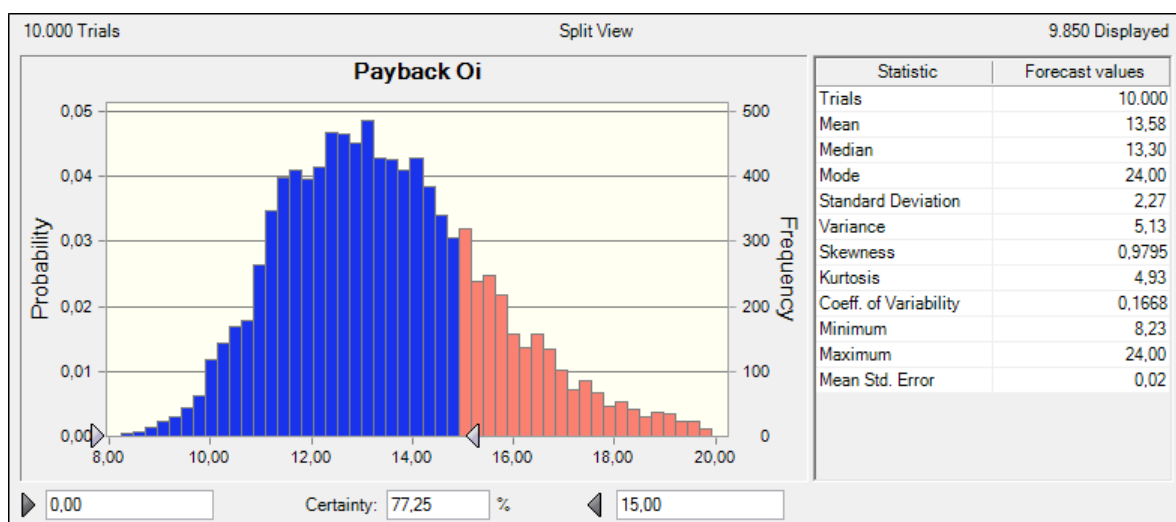
Figura 29: Distribuição de probabilidade do período de payback para a empresa Oi
