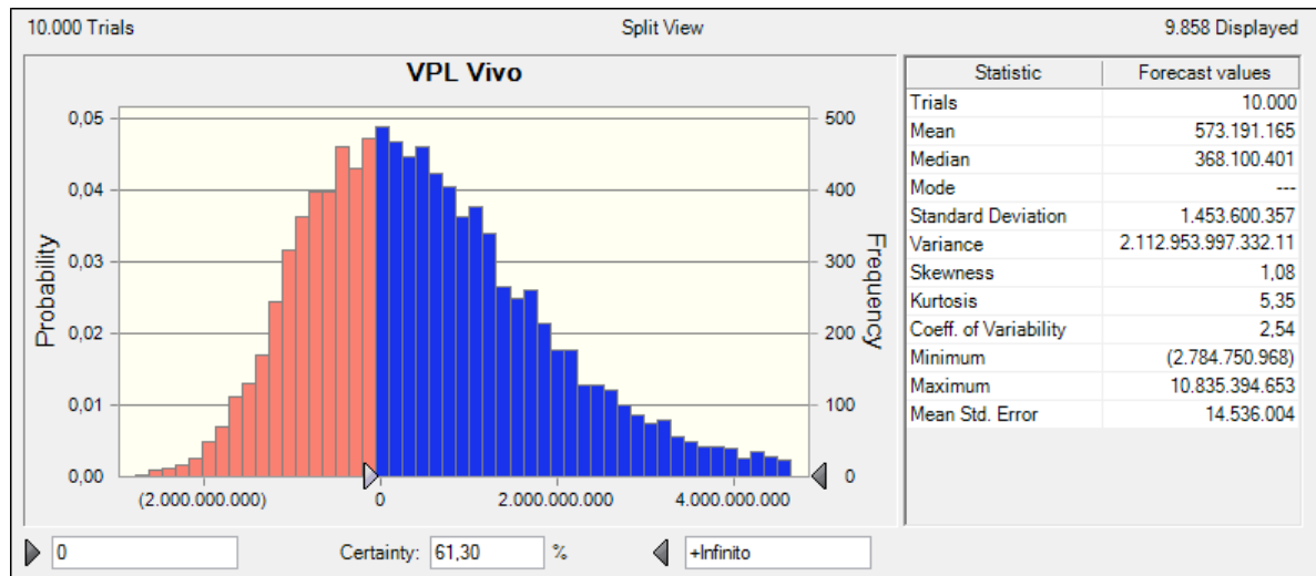
Figura 15: Distribuição de probabilidade do VPL para a empresa Vivo
