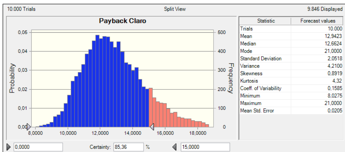
Figura 11: Distribuição de probabilidade do período de payback para a empresa Claro
