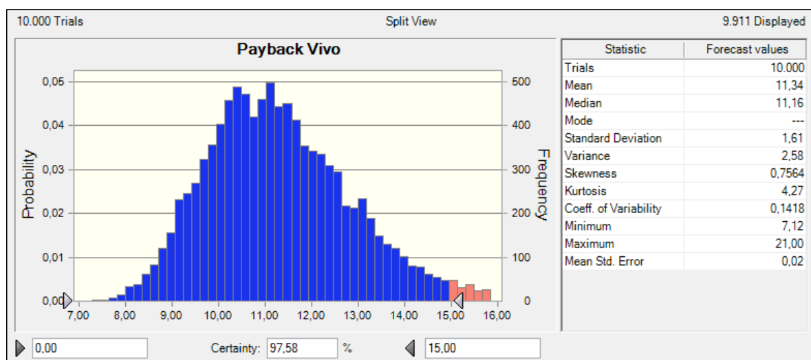
Figura 17: Distribuição de probabilidade do período de payback para a empresa Vivo
