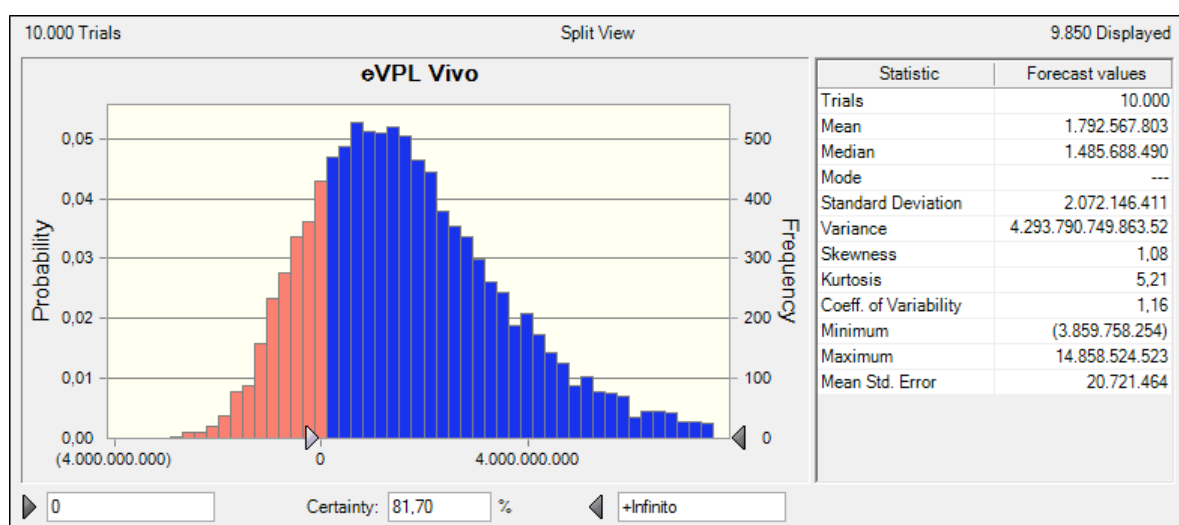
Figura 18: Distribuição de probabilidade do eVPL para a empresa Vivo
