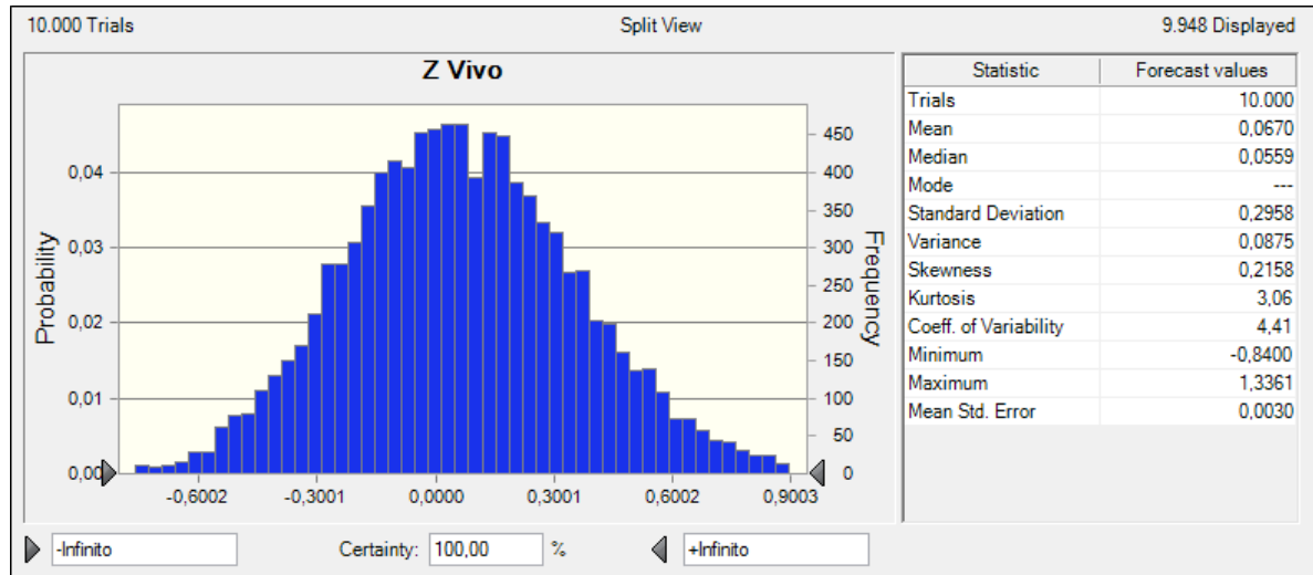
Figura 14: Distribuição de probabilidade da variável Z para a empresa Vivo
