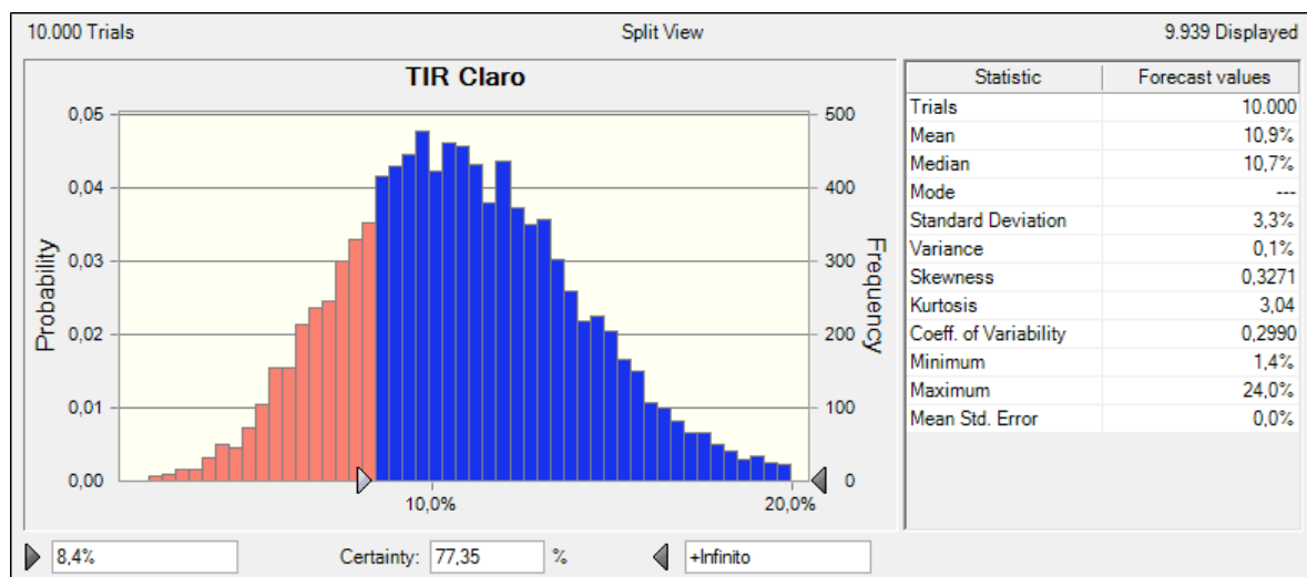
Figura 10: Distribuição de probabilidade da TIR para a empresa Claro
