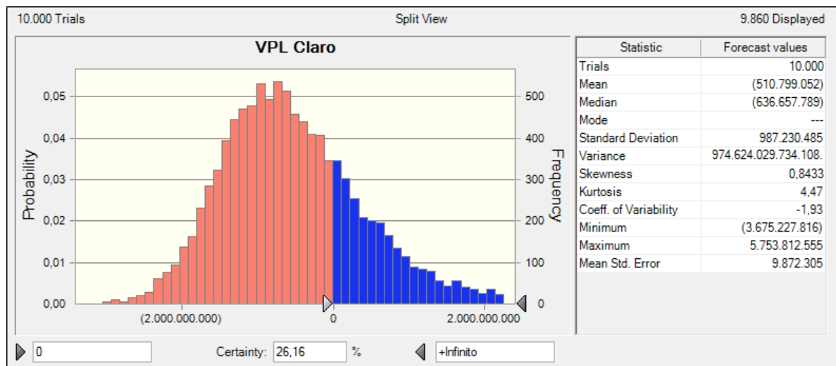
Figura 9: Distribuição de probabilidade do VPL para a empresa Claro
