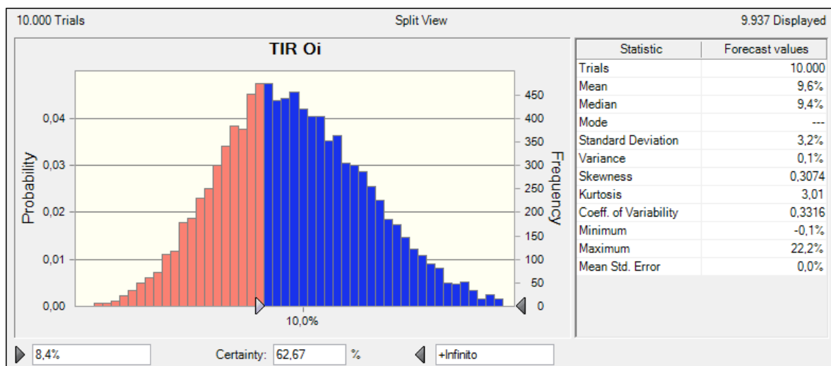
Figura 28: Distribuição de probabilidade da TIR para a empresa Oi
