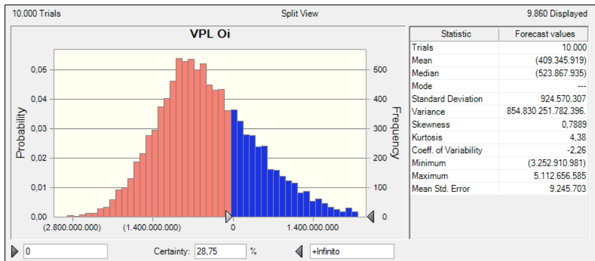
Figura 27: Distribuição de probabilidade do VPL para a empresa Oi
