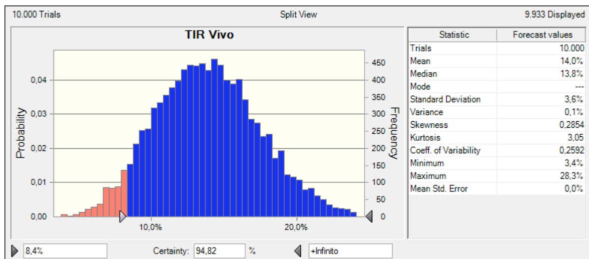
Figura 16: Distribuição de probabilidade da TIR para a empresa Vivo
