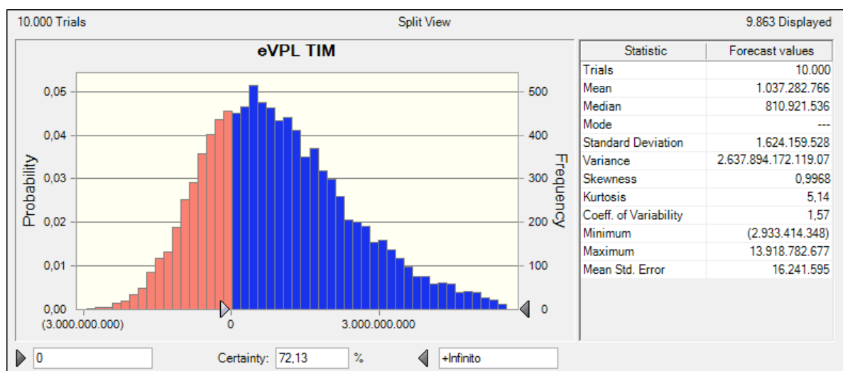
Figura 24: Distribuição de probabilidade do eVPL para a empresa TIM
