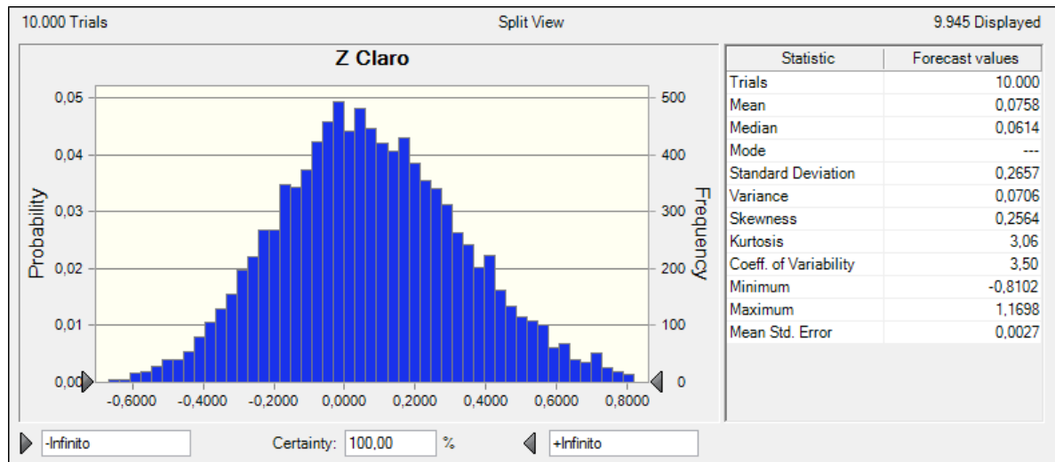
Figura 8: Distribuição de probabilidade da variável Z para a empresa Claro
