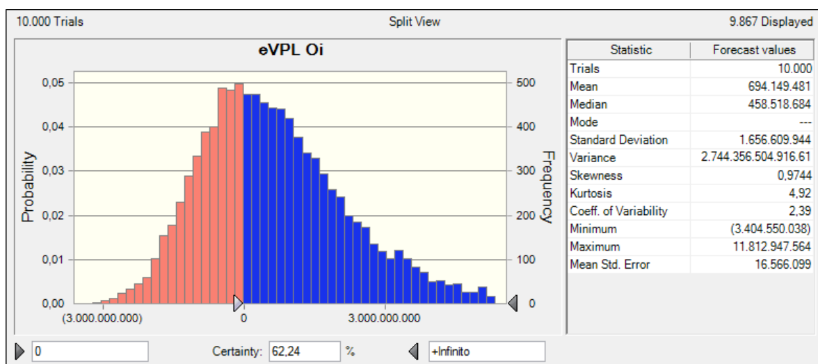
Figura 30: Distribuição de probabilidade do eVPL para a empresa Oi
