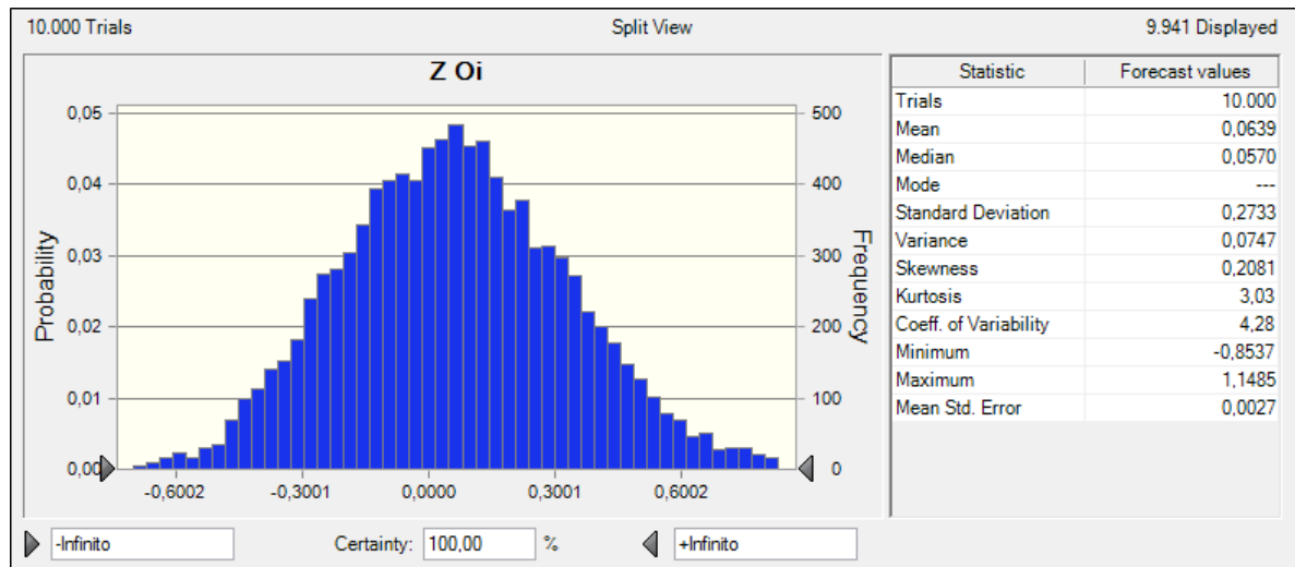
Figura 26: Distribuição de probabilidade da variável Z para a empresa Oi
