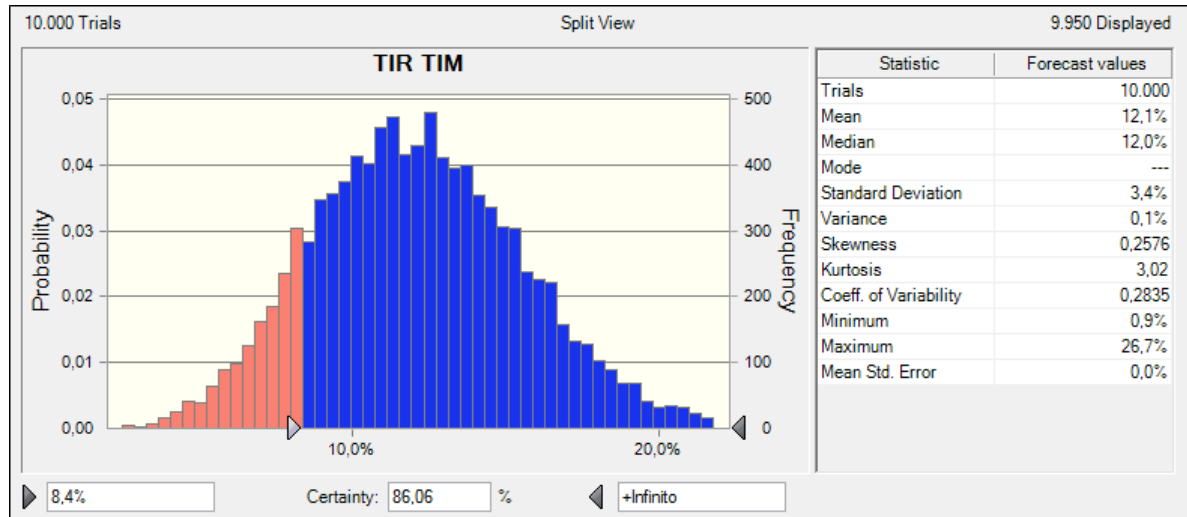
Figura 22: Distribuição de probabilidade da TIR para a empresa TIM
