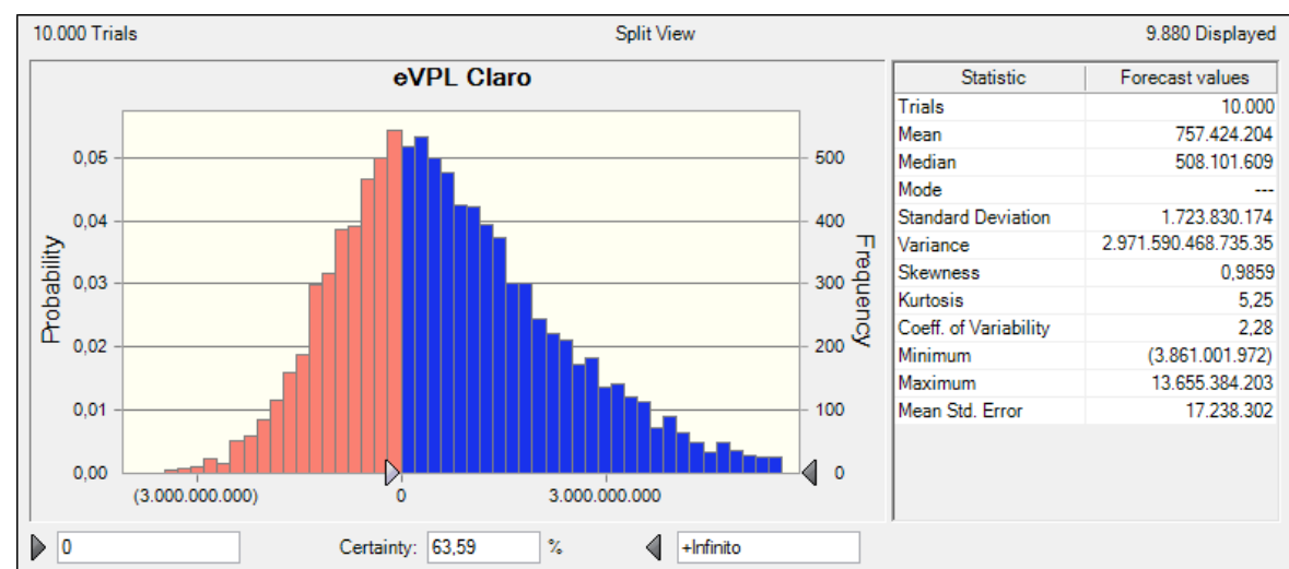
Figura 12: Distribuição de probabilidade do eVPL para a empresa Claro
