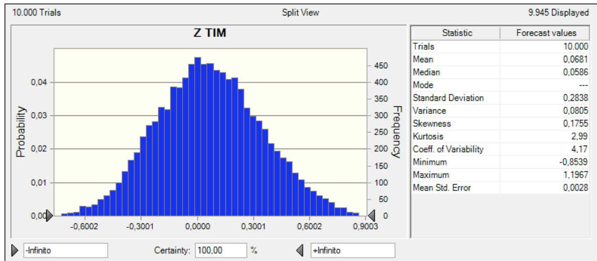
Figura 20: Distribuição de probabilidade da variável Z para a empresa TIM
