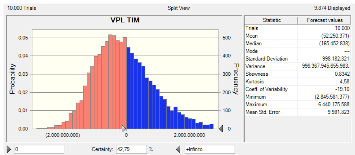
Figura 21: Distribuição de probabilidade do VPL para a empresa TIM
