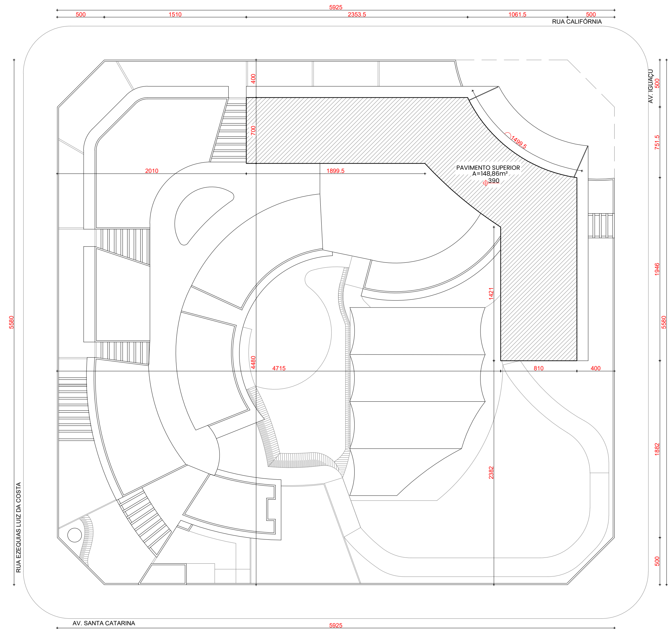
LOCAÇÃO- PAVIMENTO SUPERIOR ESCALA 1:250
