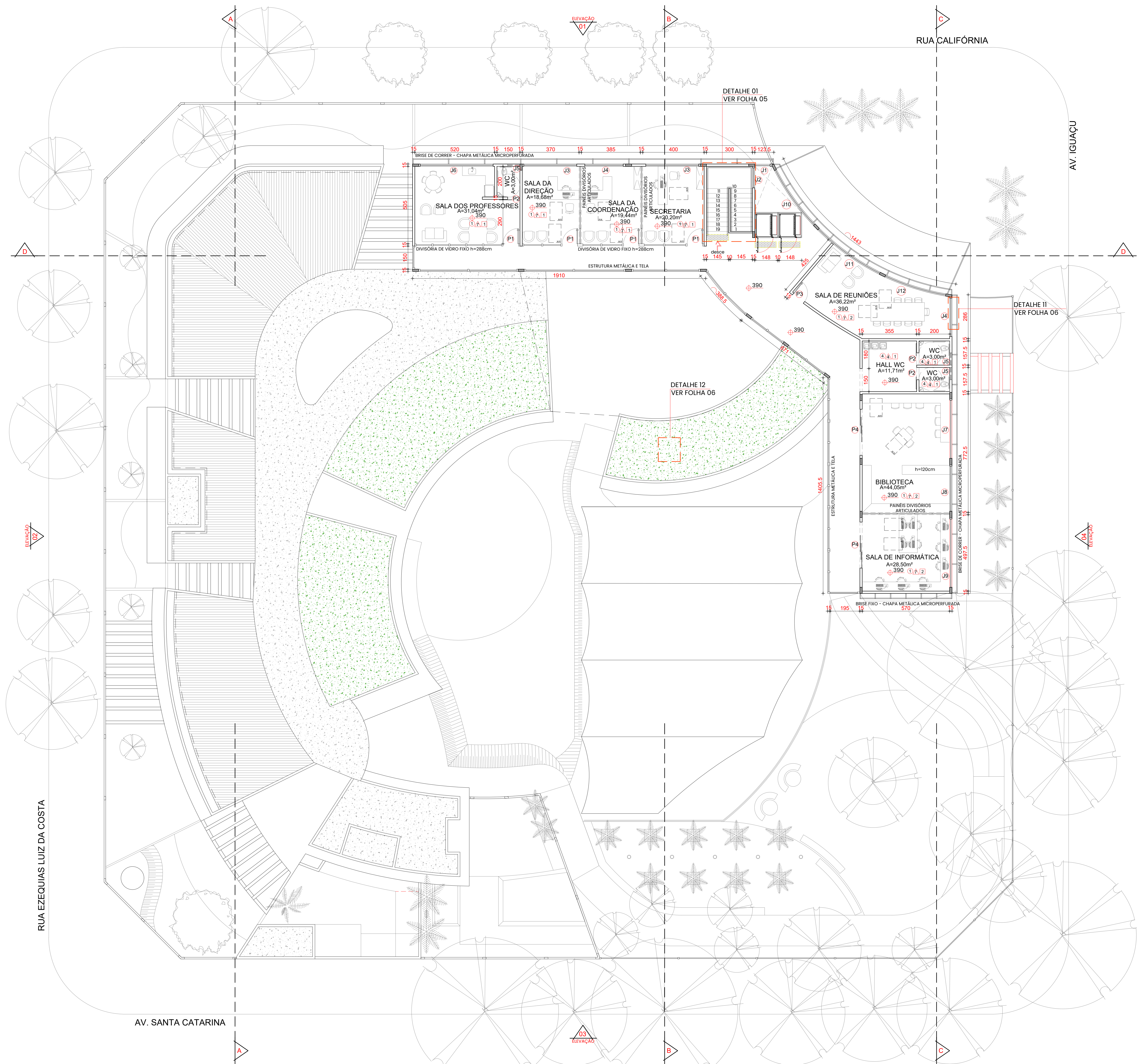
PLANTA - PAVIMENTO SUPERIOR ESCALA 1:100
