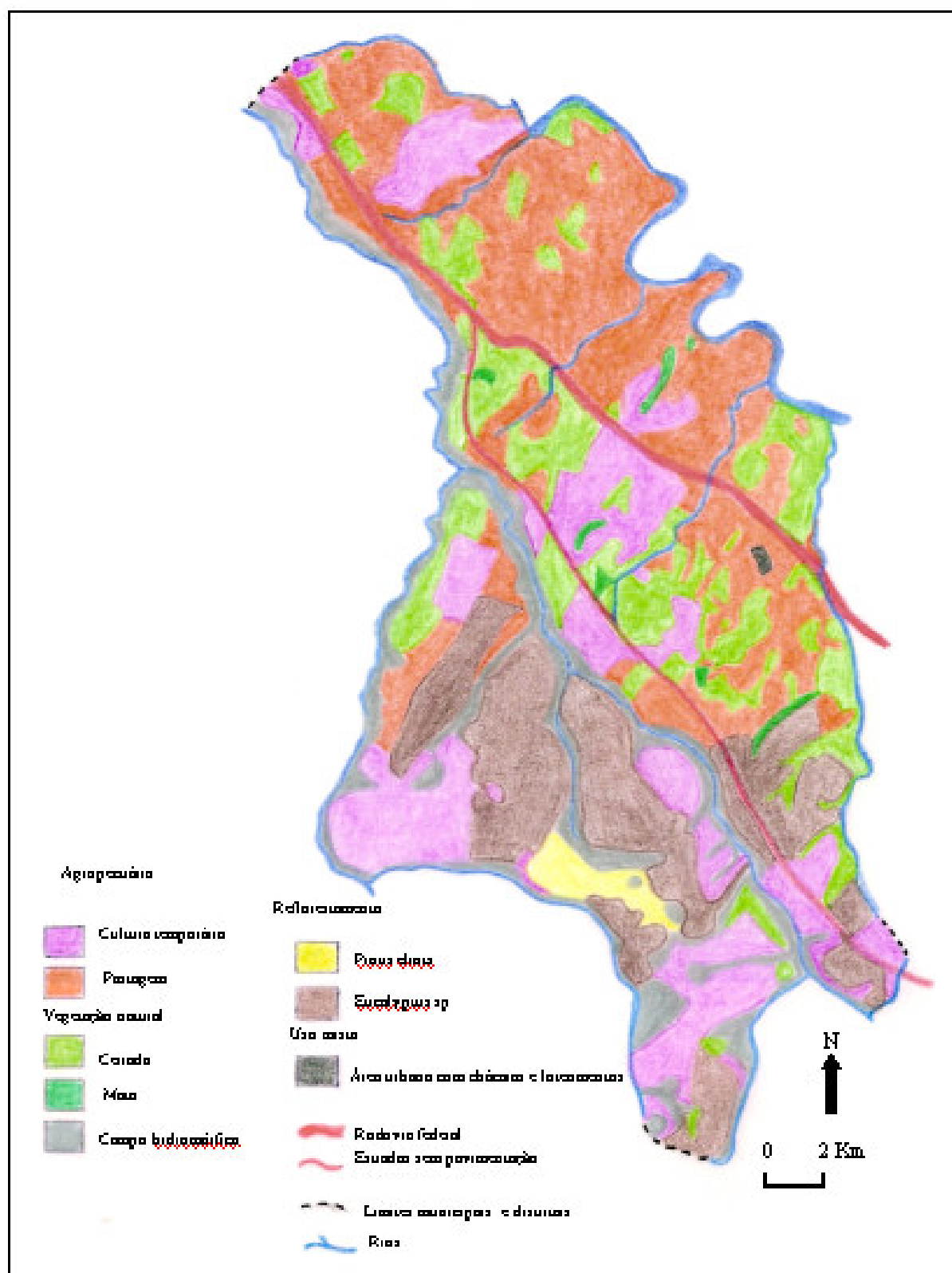
Figura 32 – Distrito de Tapuirama: uso do solo – 1988
