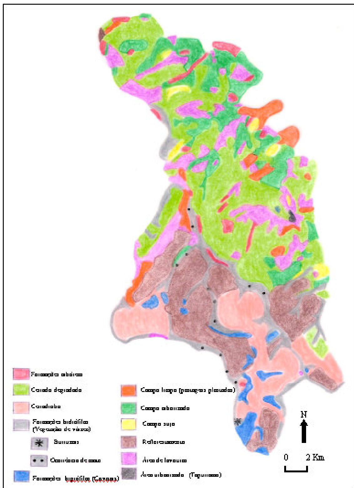
Figura 31 – Distrito de Tapuirmama: uso do solo – 1979
