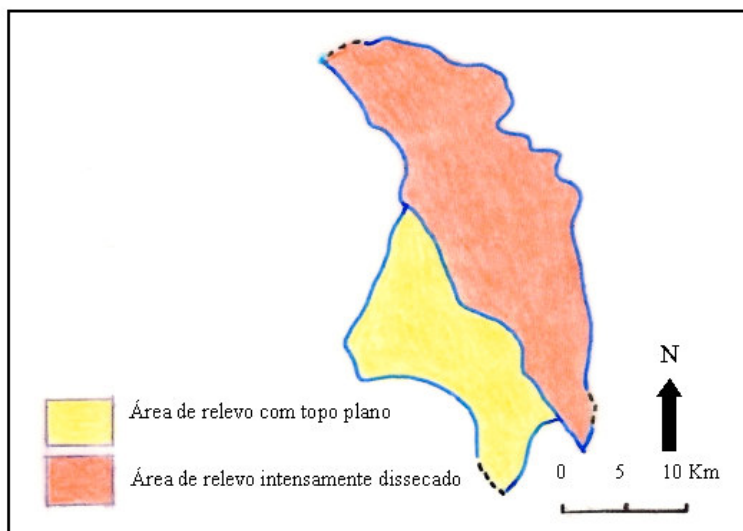
Figura 30 - Distrito de Tapuira: unidades geomorfológicas – 1997
