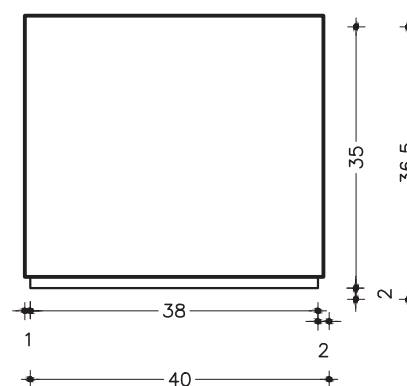
CRIADO COM RODÍZIO VISTA SUPERIOR ESC. 1:10
