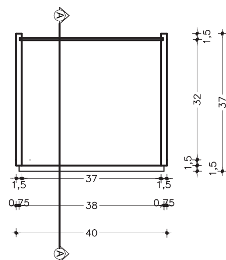
CRIADO COM RODÍZIO PLANTA ESC. 1:10
