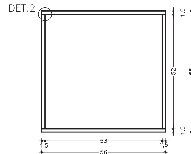
MALEIRO COM 1 PORTA VISTA FRONTAL S/ PORTA ESC. 1:10
