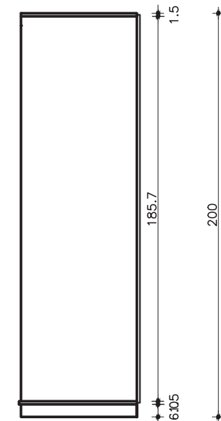
GUARDA-ROUPA COM 2 PORTAS VISTA LATERAL ESC. 1:25
