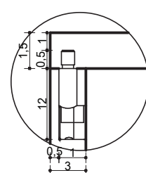
DETALHE 2 ENCAIXE MINIFIX ESC. 1:5
