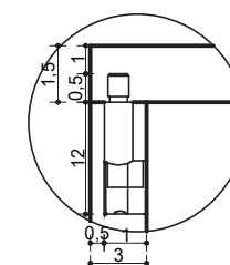
DETALHE 2 ENCAIXE MINIFIX ESC. 1:5
