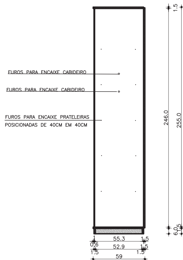
GUARDA ROUPA COM DE 2 PORTAS CORTE AA ESC. 1:25
