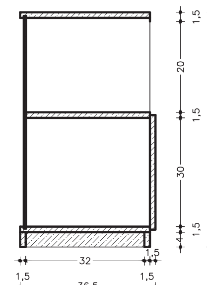
CRIADO COM RODAPÉ CORTE AA ESC. 1:10
