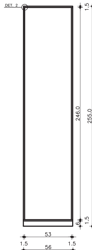
GUARDA-ROUPA COM 1 PORTA VISTA FRONTAL S/ PORTAS ESC. 1:25
