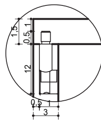
DETALHE 2 ENCAIXE MINIFIX FSC. 1:5
