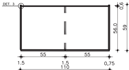
GUARDA ROUPA COM DE 2 PORTAS PLANTA ESC. 1:25
