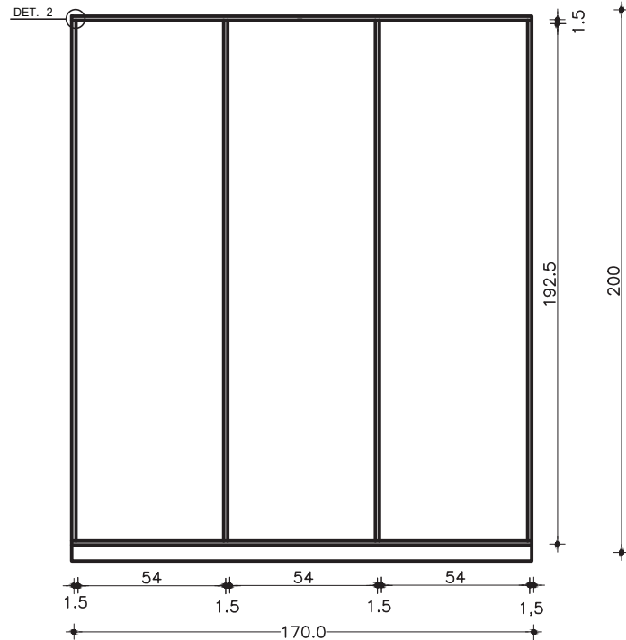
GUARDA-ROUPA COM 3 PORTAS VISTA FRONTAL S/ PORTAS ESC. 1:25
