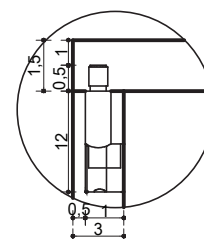
DETALHE 2 ENCAIXE MINIFIX FSC. 1:5
