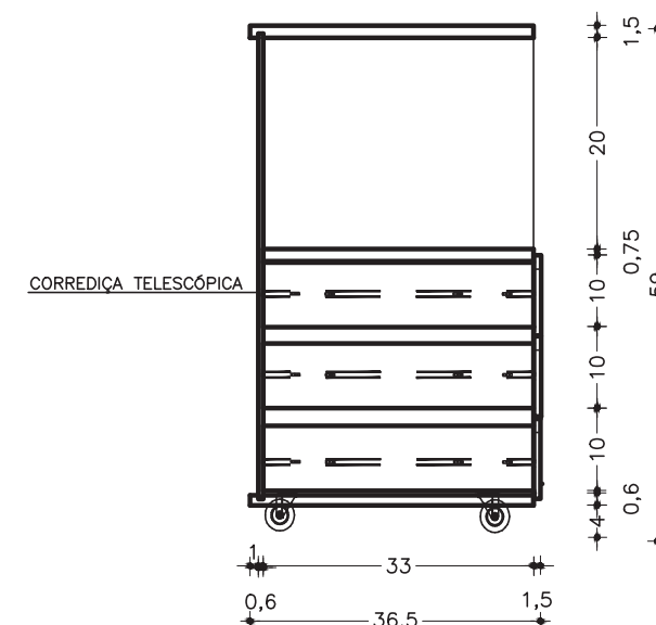
CRIADO COM RODAPÉ CORTE AA ESC. 1:10
