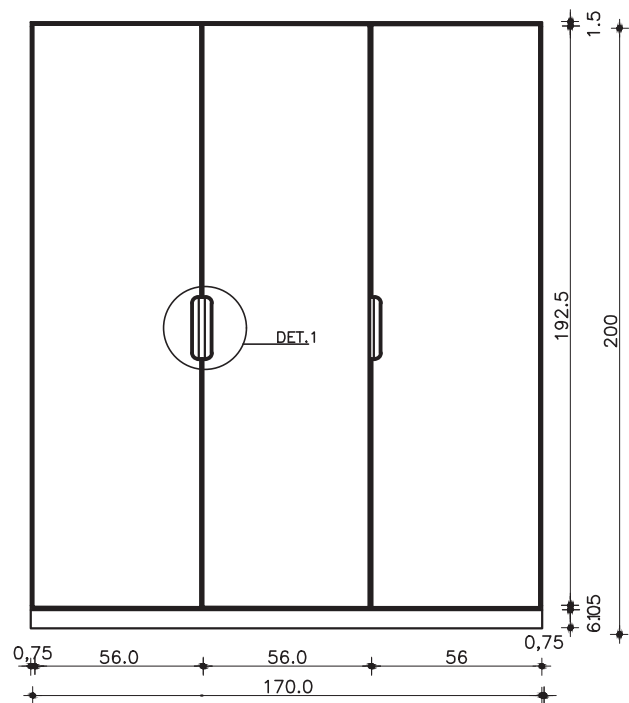
GUARDA-ROUPA COM 3 PORTAS VISTA FRONTAL C/ PORTAS ESC. 1:25
