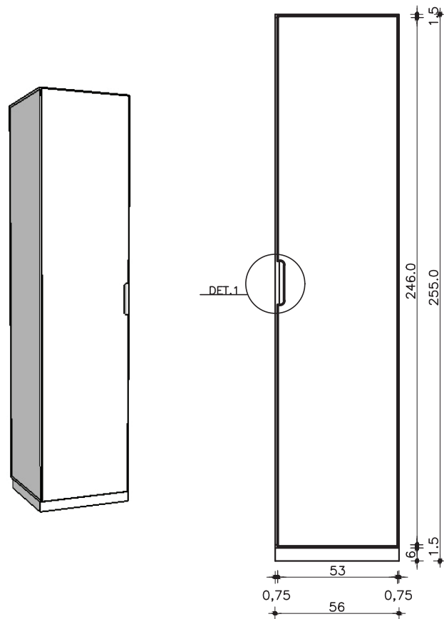
GUARDA-ROUPA COM 1 PORTA PERSPECTIVA ESC. 1:25
