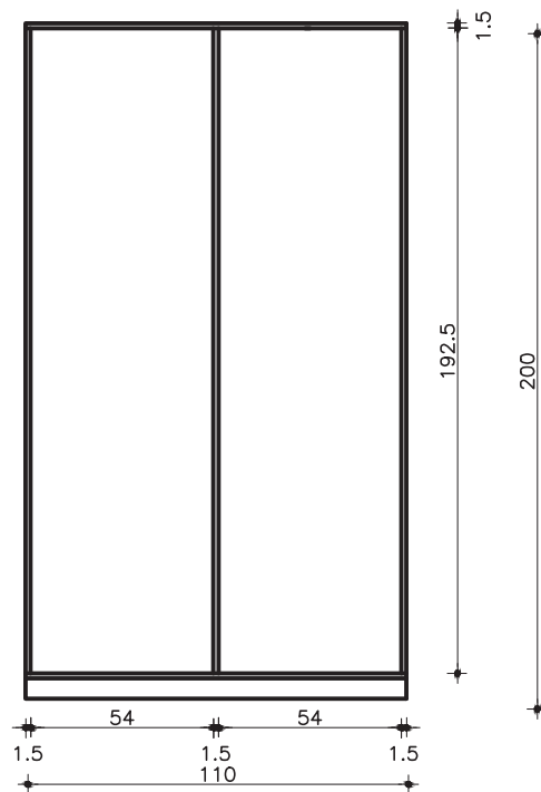
GUARDA-ROUPA COM 2 PORTAS VISTA FRONTAL S/ PORTAS ESC. 1:25
