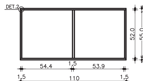
GUARDA-ROUPA COM 2 PORTAS VISTA FRONTAL S/ PORTAS ESC. 1:25
