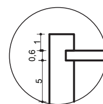
DETALHE 3 ENCAIXE CHAPA FUNDO ESC. 1:5
