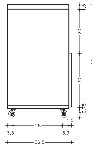
CRIADO COM RODÍZIO VISTA LATERAL ESC. 1:10
