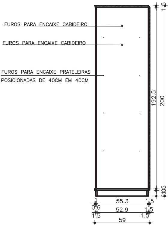
GUARDA ROUPA COM DE 1 PORTA CORTE AA ESC. 1:25
