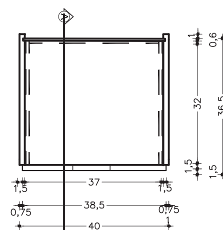
CRIADO COM RODÍZIO PLANTA ESC. 1:10
