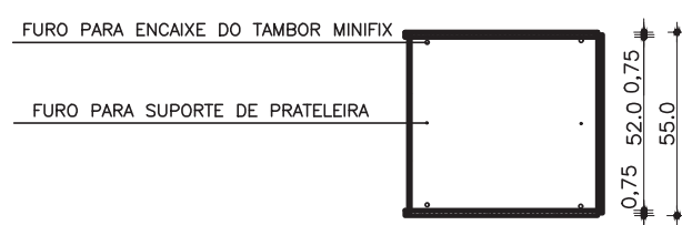
GUARDA-ROUPA COM 2 PORTAS CORTE AA ESC. 1:25
