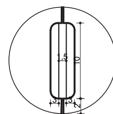
DETALHE 1 PUXADOR FSC. 1:5
