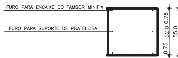
GUARDA-ROUPA COM 3 PORTAS CORTE AA ESC. 1:25
