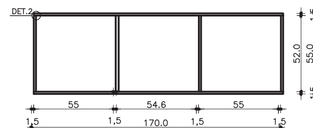
GUARDA-ROUPA COM 3 PORTAS VISTA FRONTAL S/ PORTAS ESC. 1:25
