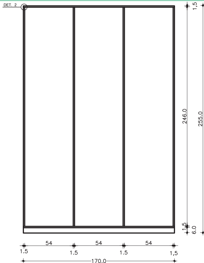
GUARDA-ROUPA COM 3 PORTAS VISTA FRONTAL S/ PORTAS ESC. 1:25
