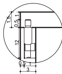
DETALHE 2 ENCAIXE MINIFIX
