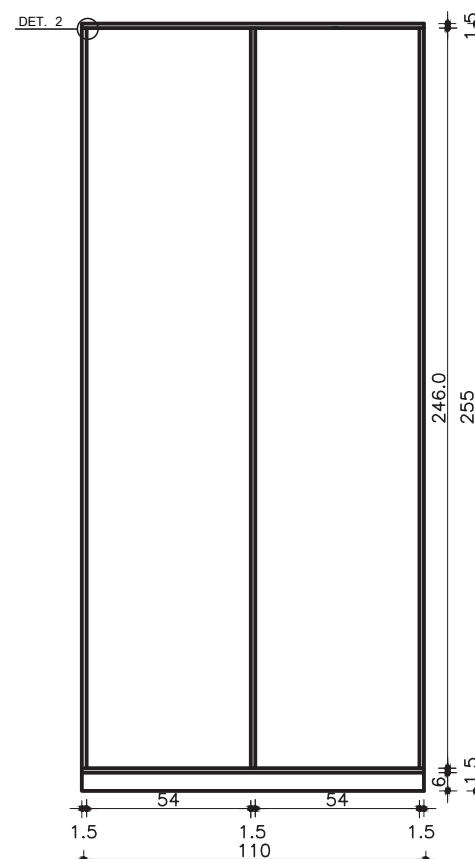
GUARDA-ROUPA COM 2 PORTAS VISTA FRONTAL S/ PORTAS ESC. 1:25
