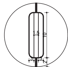
DETALHE 1 PUXADOR ESC. 1:5
