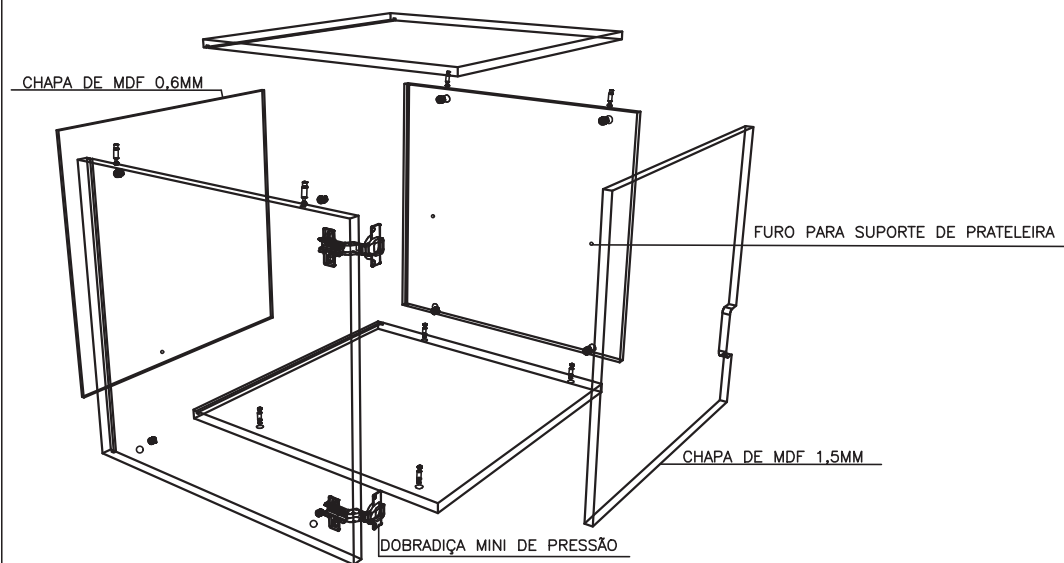
MALEIRO COM 1 PORTA PERSPECTIVA EXPLODIDA ESC. 1:10
