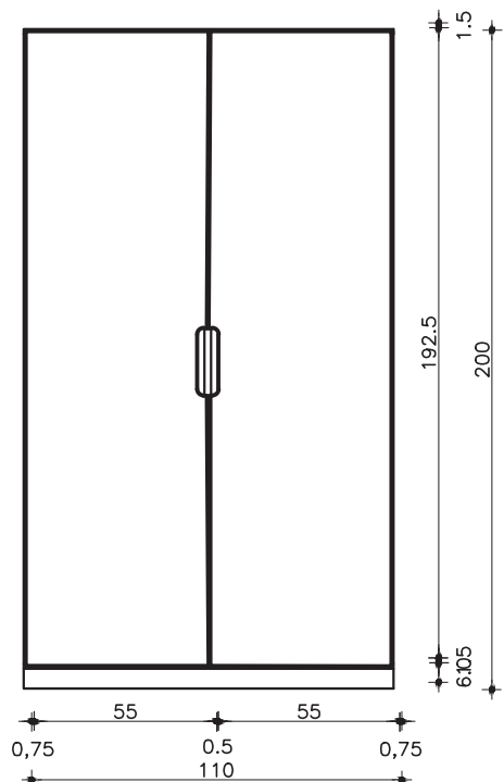
GUARDA-ROUPA COM 2 PORTAS VISTA FRONTAL C/ PORTAS ESC. 1:25
