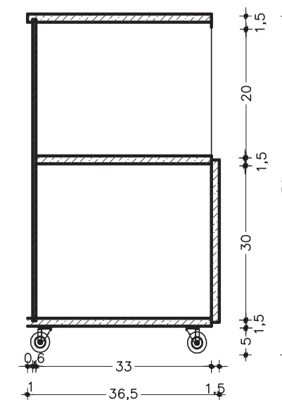
CRIADO COM RODÍZIO CORTE AA ESC. 1:10
