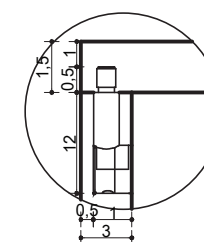
DETALHE 2 ENCAIXE MINIFIX ESC. 1:5
