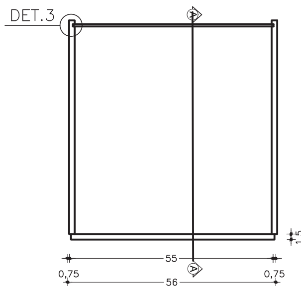
MALEIRO COM 1 PORTA PLANTA ESC. 1:10
