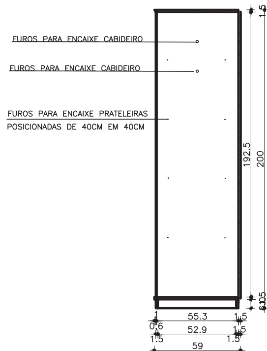
GUARDA ROUPA COM DE 3 PORTAS CORTE AA ESC. 1:25
