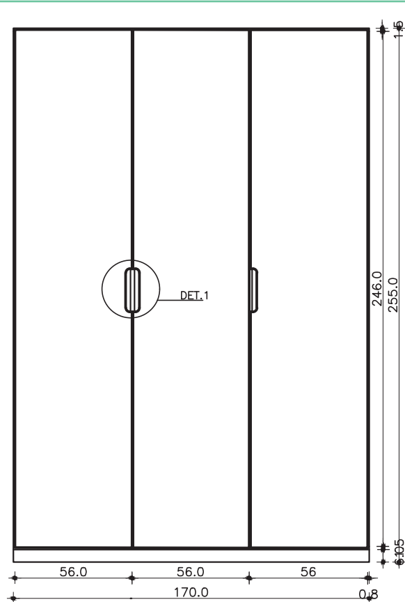
GUARDA-ROUPA COM 3 PORTAS VISTA FRONTAL C/ PORTAS ESC. 1:25
