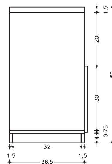
CRIADO COM RODAPÉ VISTA LATERAL ESC. 1:10
