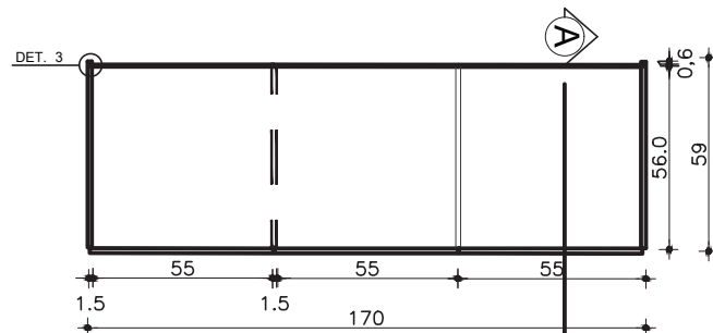
GUARDA ROUPA COM DE 3 PORTAS PLANTA ESC. 1:25
