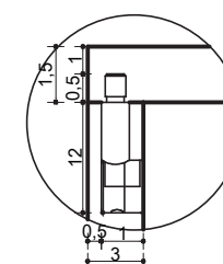
DETALHE 2 ENCAIXE MINIFIX
