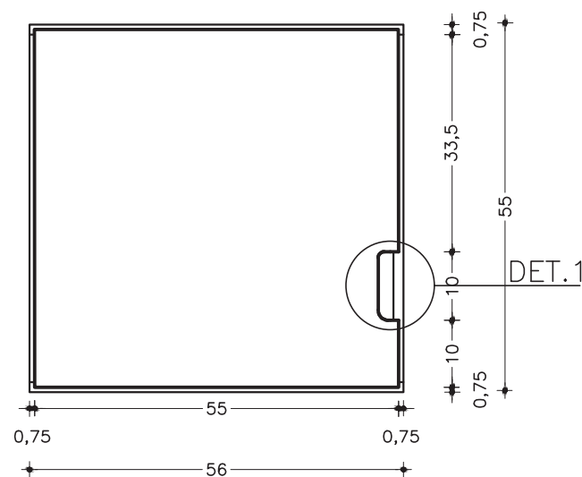
MALEIRO COM 1 PORTA VISTA FRONTAL C/ PORTA ESC. 1:10
