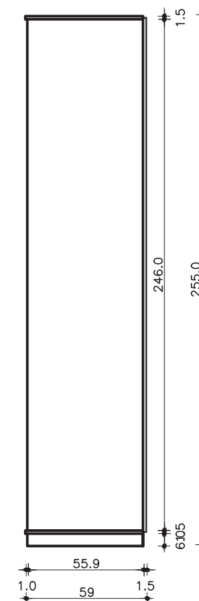
GUARDA-ROUPA COM 1 PORTA VISTA LATERAL ESC. 1:25
