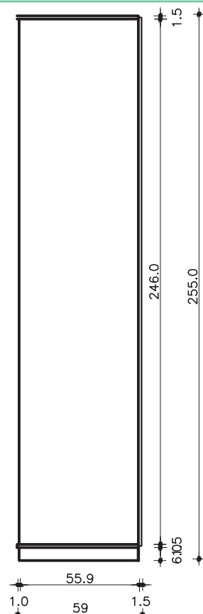
GUARDA-ROUPA COM 3 PORTAS VISTA LATERAL ESC. 1:25
