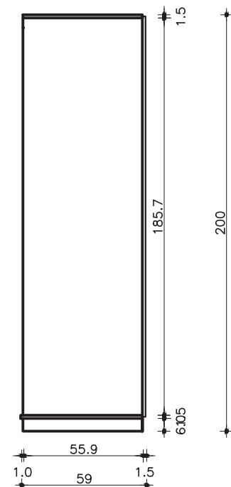
GUARDA-ROUPA COM 3 PORTAS VISTA LATERAL ESC. 1:25
