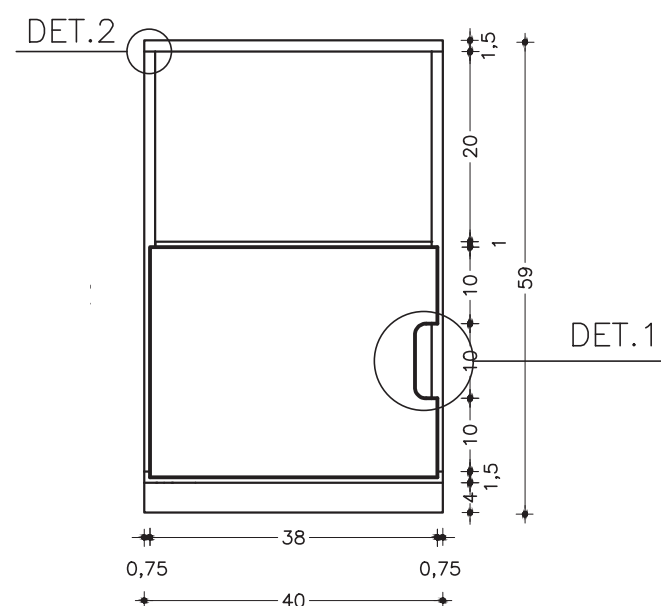
CRIADO COM RODAPÉ VISTA FRONTAL ESC. 1:10
