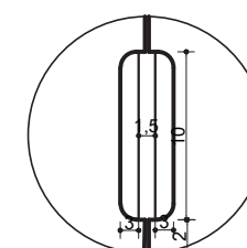
DETALHE 4 PUXADOR
