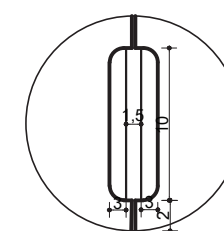
DETALHE 4 PUXADOR ESC. 1:5
