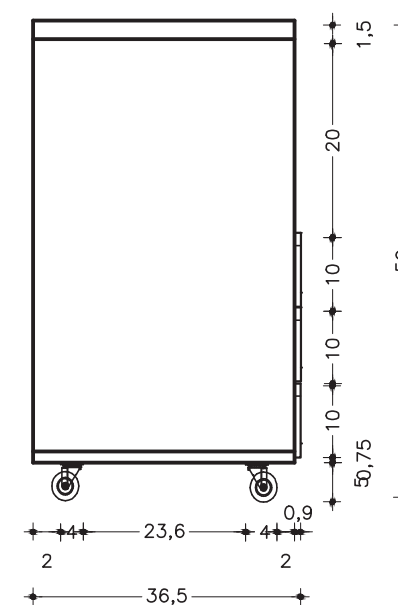
CRIADO COM RODÍZIO VISTA LATERAL ESC. 1:10
