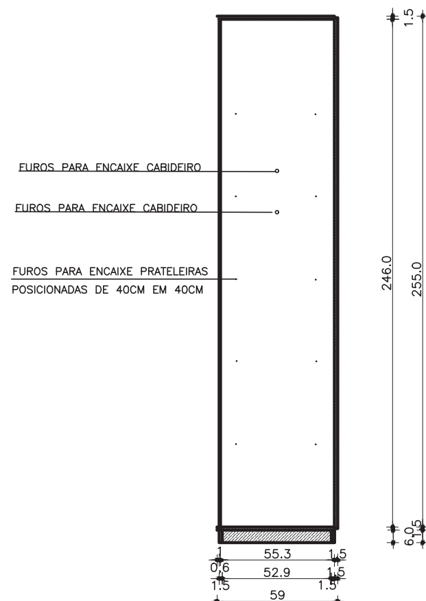
GUARDA ROUPA COM DE 1 PORTA CORTE AA ESC. 1:25
