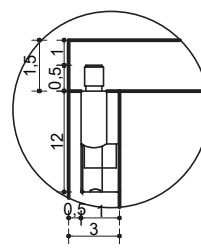
DETALHE 2 ENCAIXE MINIFIX ESC. 1:5
