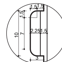
DETALHE 1 PUXADOR ESC. 1:5
