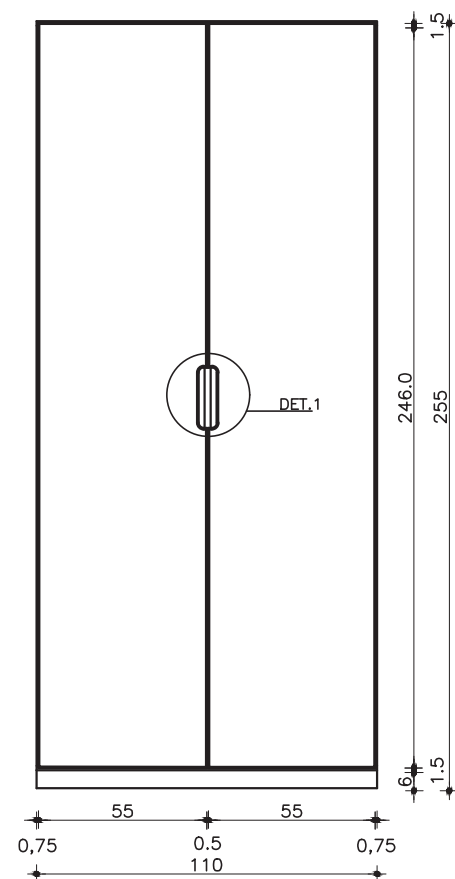
GUARDA-ROUPA COM 2 PORTAS VISTA FRONTAL C/ PORTAS ESC. 1:25
