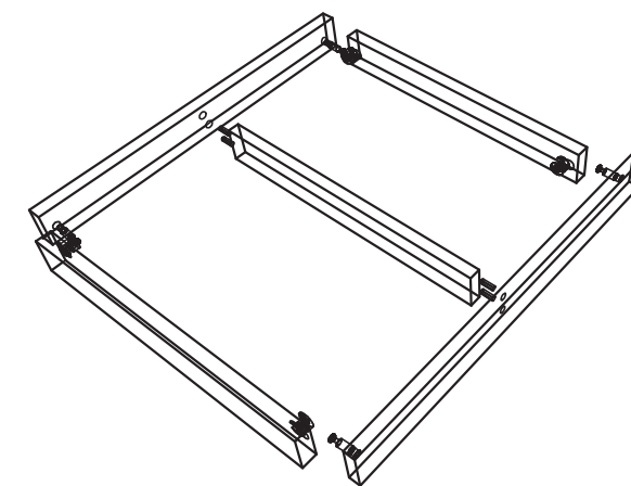
RODAPÉ PERSPECTIVA EXPLODIDA ESC. 1:25
