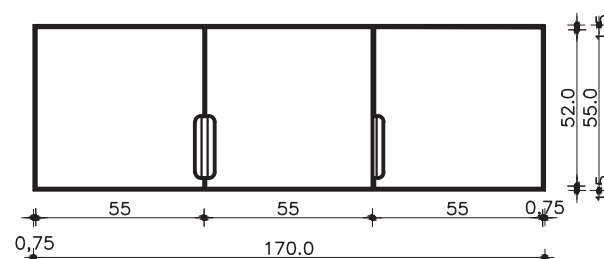
GUARDA-ROUPA COM 3 PORTAS VISTA FRONTAL C/ PORTAS ESC. 1:25
