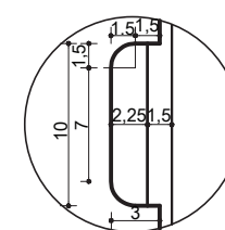
DETALHE 1 PUXADOR ESC. 1:5
