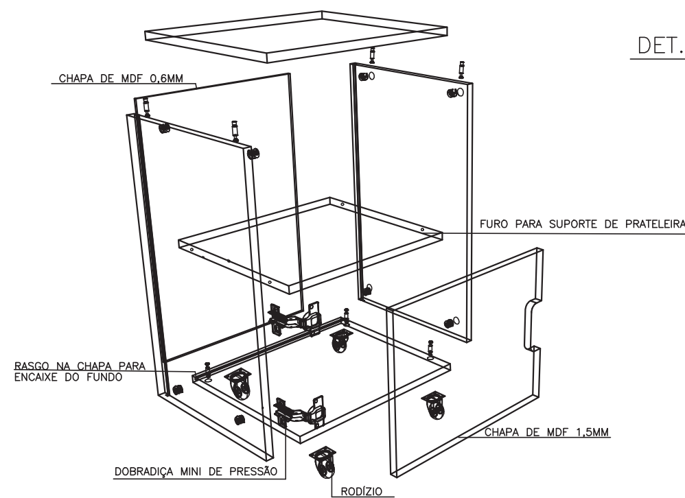
CRIADO COM RODÍZIO PERSPECTIVA EXPLODIDA
