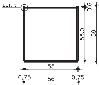
GUARDA ROUPA COM DE 1 PORTA PLANTA ESC. 1:25
