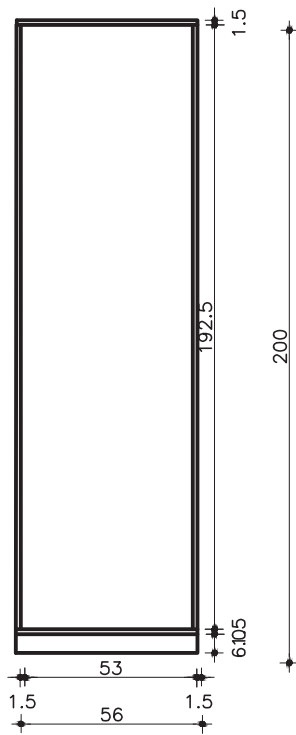
GUARDA-ROUPA COM 1 PORTA VISTA FRONTAL S/ PORTAS ESC. 1:25
