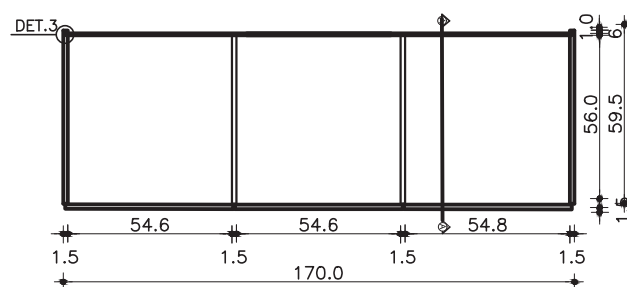
GUARDA-ROUPA COM 3 PORTAS PLANTA ESC. 1:25
