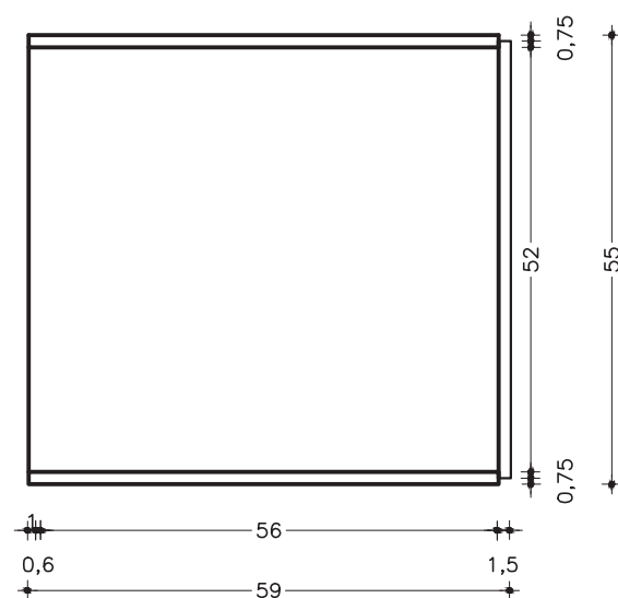
MALEIRO COM 1 PORTA VISTA LATERAL ESC. 1:10
