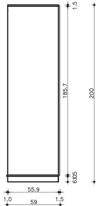
GUARDA-ROUPA COM 1 PORTA VISTA LATERAL ESC. 1:25
