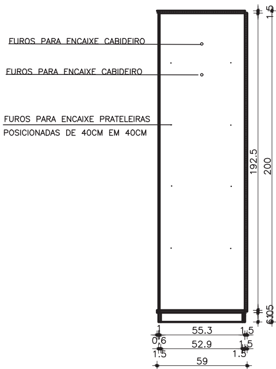
GUARDA ROUPA COM DE 2 PORTAS CORTE AA ESC. 1:25
