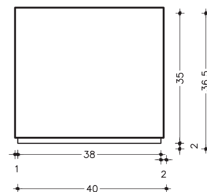
CRIADO COM RODAPÉ VISTA SUPERIOR ESC. 1:10
