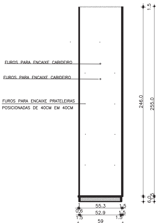
GUARDA ROUPA COM DE 3 PORTAS CORTE AA ESC. 1:25
