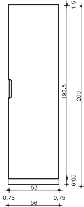
GUARDA-ROUPA COM 1 PORTA VISTA FRONTAL C/ PORTAS ESC. 1:25
