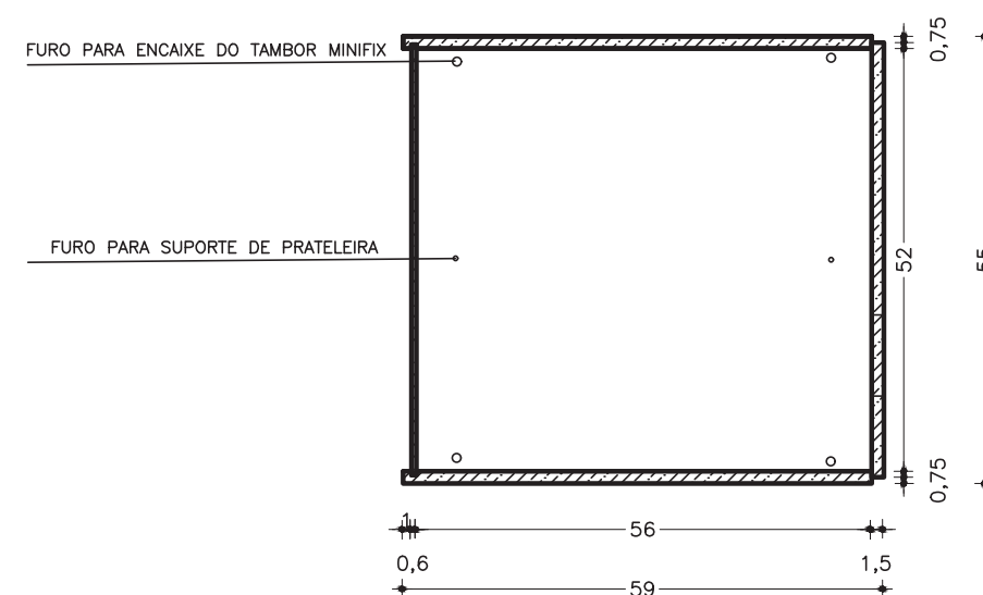
MALEIRO COM 1 PORTA CORTE AA ESC. 1:10
