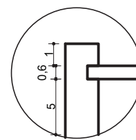
DETALHE 3 ENCAIXE CHAPA FUNDO ESC. 1:5
