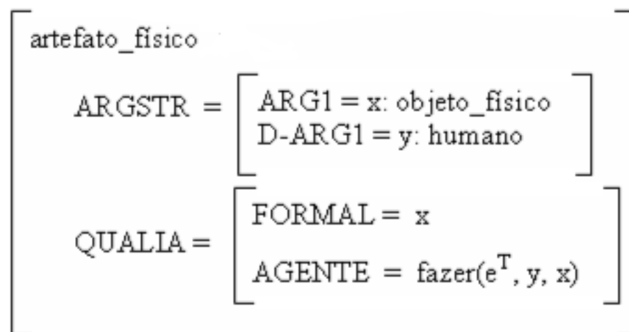
Figura 56: Estrutura lexical para o item artefato_fisico .
