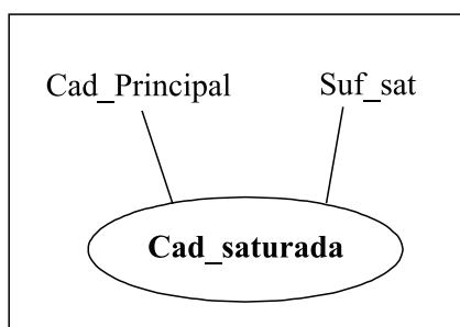
Figura 69: Regra para o Nome de Compostos Saturados
