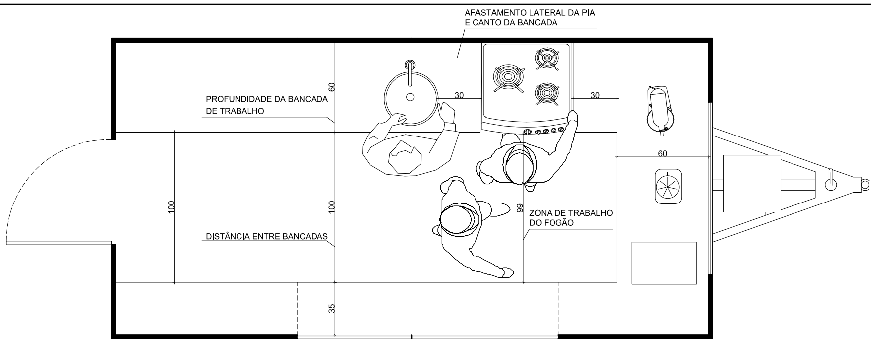
FOOD CART DOCERIA LUZ ANÁLISE ERGONÔMICA ESC. 1:25
