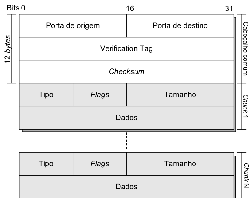
Figura 3.7: Formato do pacote SCTP
