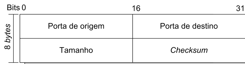
Figura 3.2: Cabeçalho do protocolo UDP
