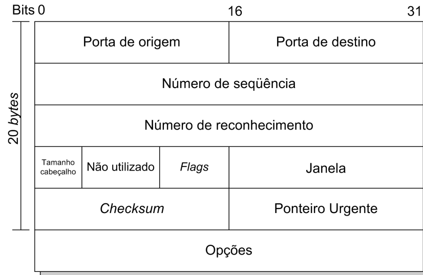
Figura 3.3: Cabeçalho do protocolo TCP
