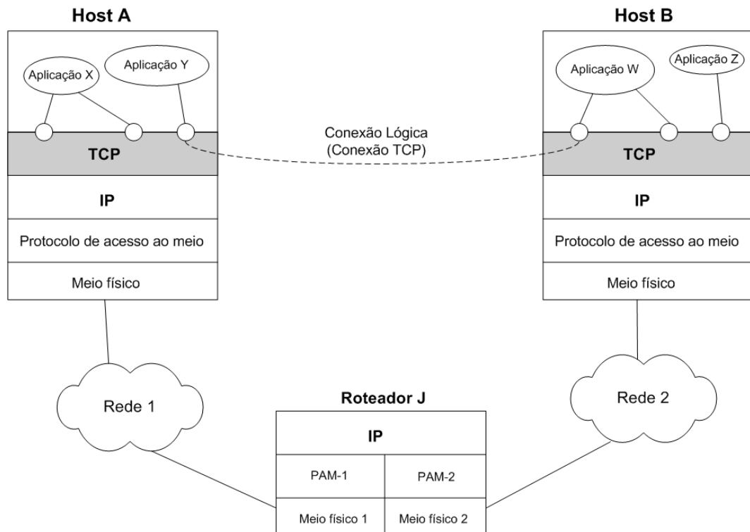
Figura 3.1: Comunicação lógica entre dois processos, em dois hosts diferentes
