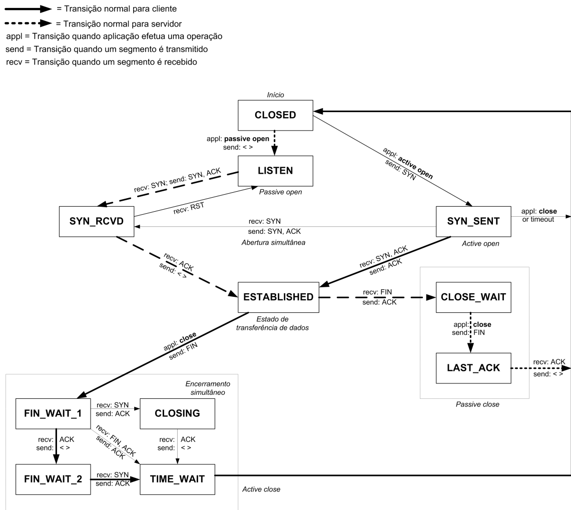
Figura 3.5: Estados de uma conexão TCP
