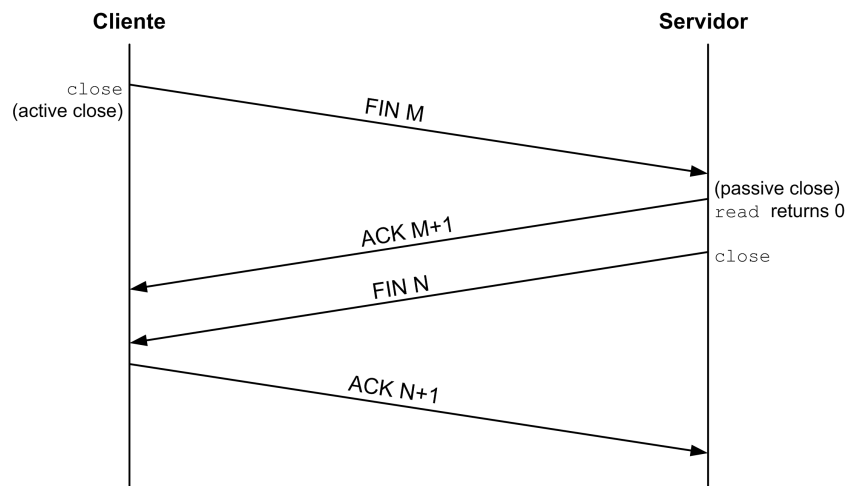
Figura 3.6: Encerramento de conexão TCP
