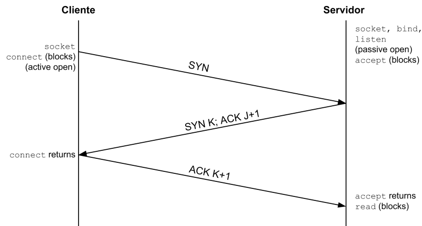
Figura 3.4: Iniciação de conexão TCP
