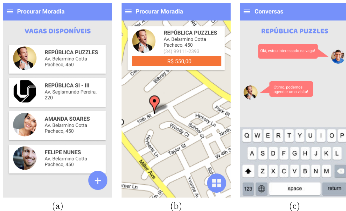
Figura 16 – (a) Tela de moradias disponíveis, (b) tela de informações adicionais e (c) tela de chat
