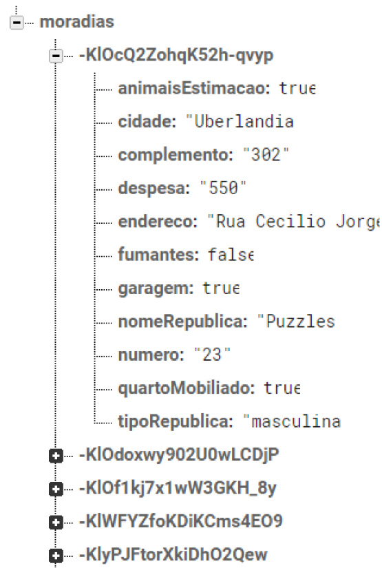
Figura 8 – Estrutura de nós do Firebase
