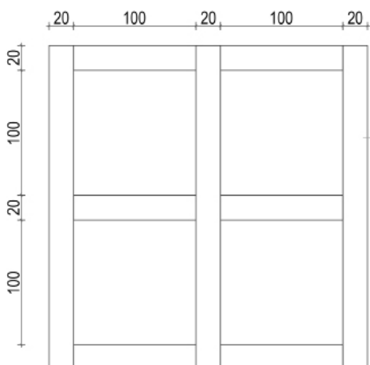
SISTEMA ESTRUTURAL DAS VIGAS / Centro de Extensão
