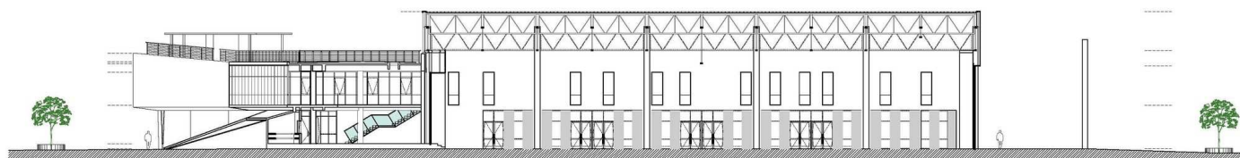
CORTE TRANSVERSAL 1
