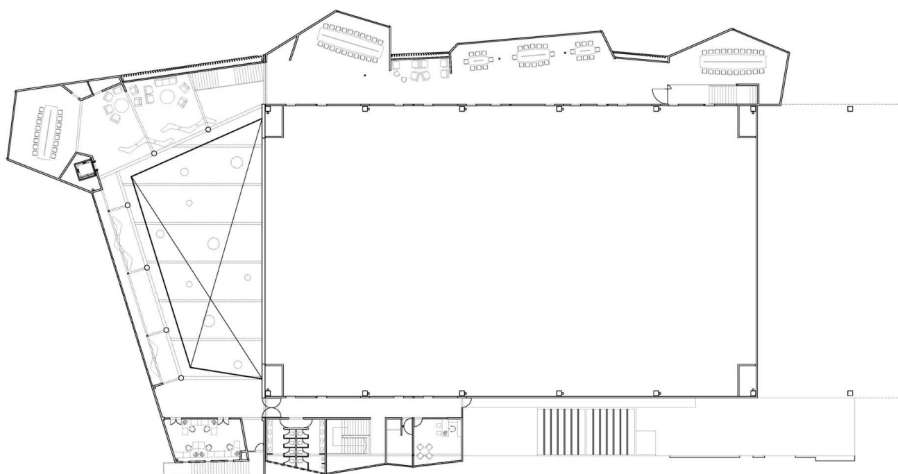
PLANTA NÍVEL 2
