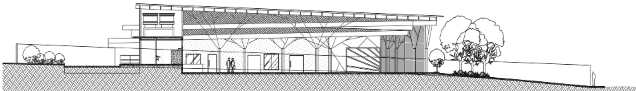
CORTE TRANSVERSAL / Centro de Extensão
