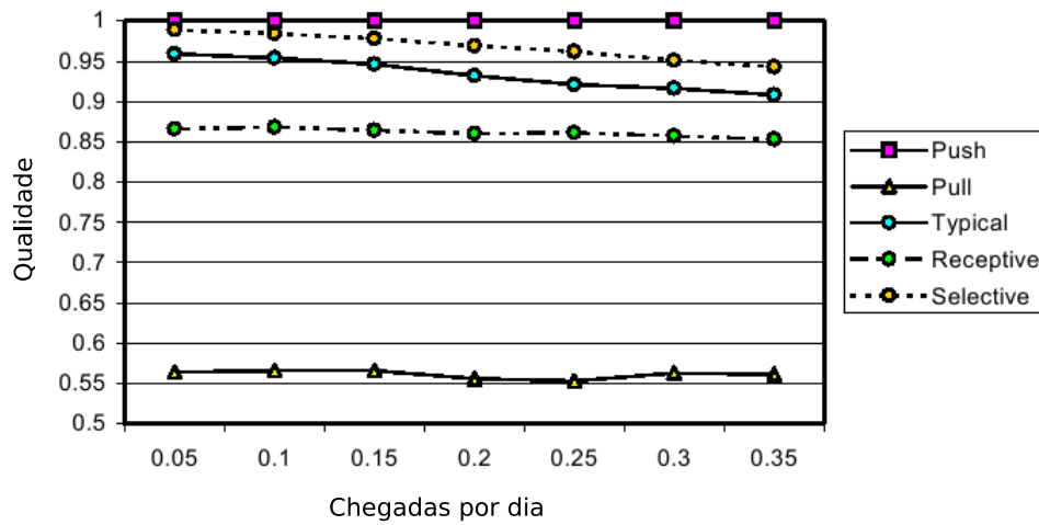
Figura 4.3: Resultados de Kumar et al. . Média de métricas de qualidade.
