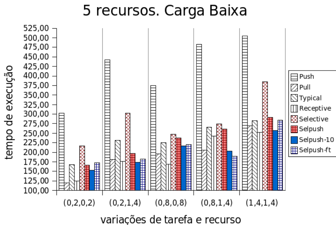
Figura 5.3: Variação de tempos com carga de sistema baixa no tempo de execução
