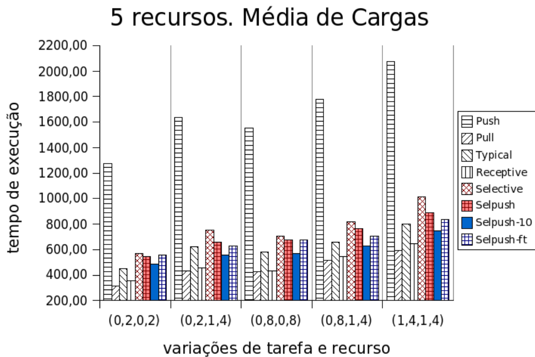
Figura 5.6: Impacto de variação de tarefa e recurso no tempo de execução com média de cargas de sistema
