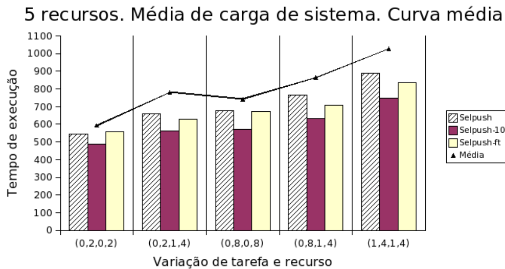
Figura 5.11: Comparação entre os mecanismos e a média de tempo
