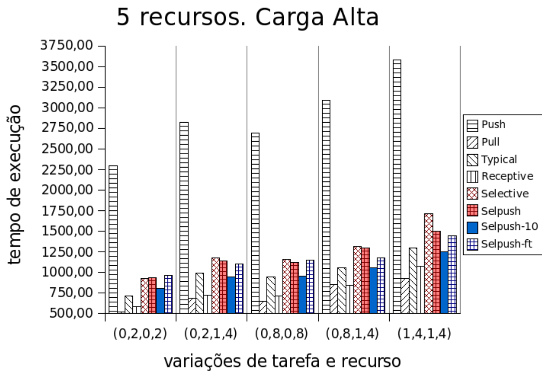
Figura 5.5: Variação de tempos com carga de sistema alta no tempo de execução
