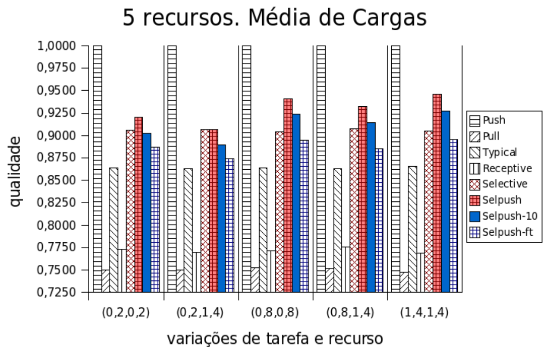
Figura 5.10: Impacto de variação de tarefa e recurso na qualidade com média de cargas de sistema
