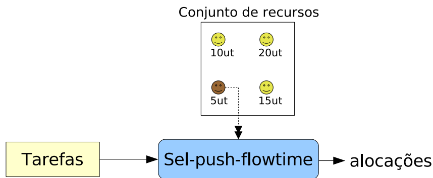
Figura 4.6: Esquema de funcionamento Sel-push-flowtime
