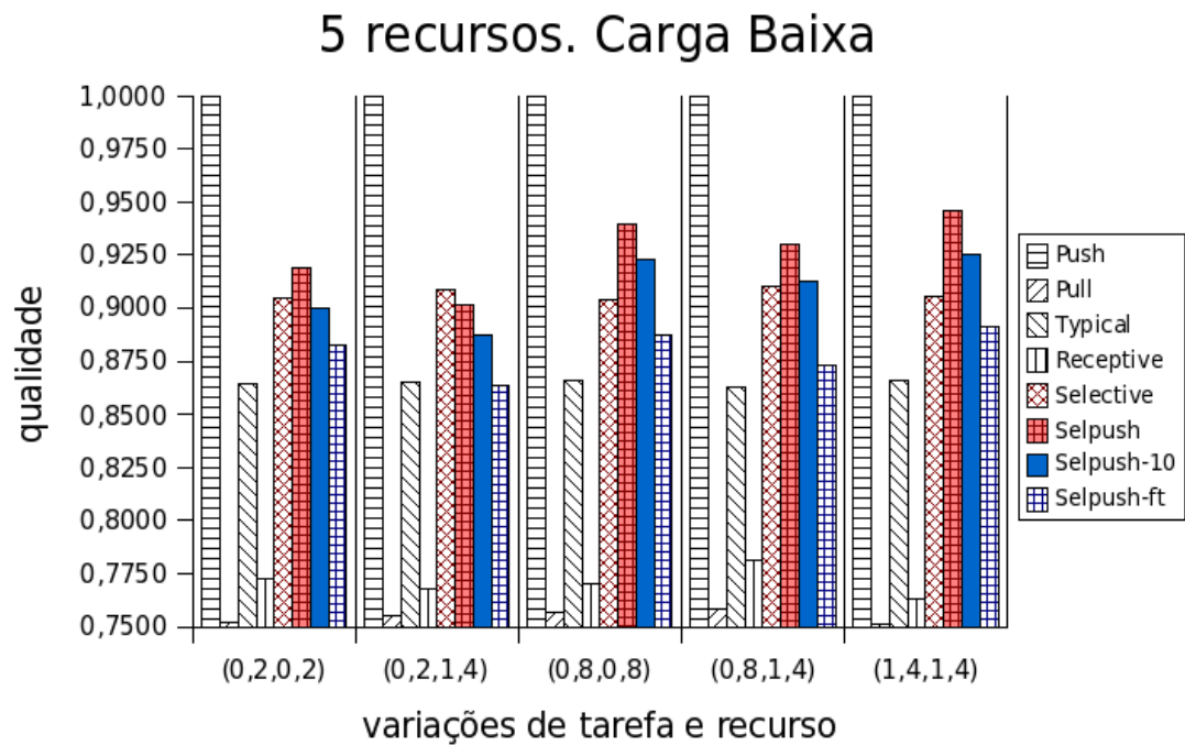
Figura 5.7: Variação de tempos com carga de sistema baixa na qualidade
