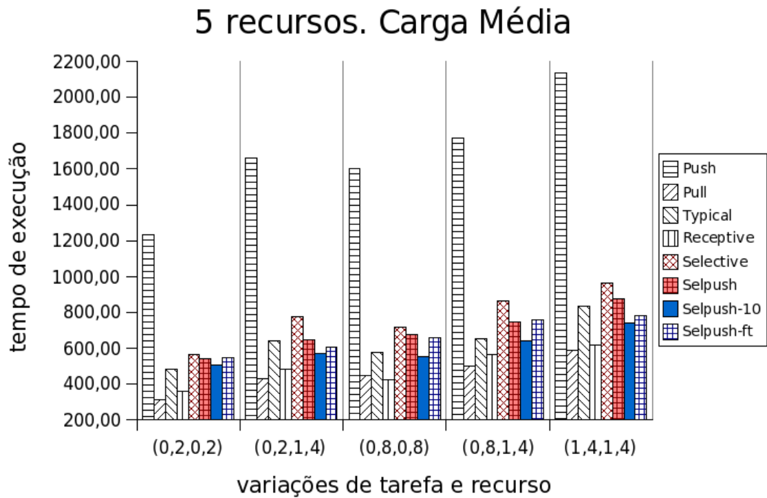
Figura 5.4: Variação de tempos com carga de sistema média no tempo de execução
