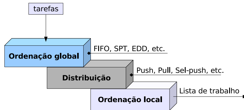
Figura 3.1: Passos que envolvem o processo de alocação de tarefas
