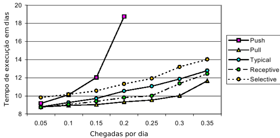
Figura 4.2: Resultados de Kumar et al. . Média de tempos de execução.
