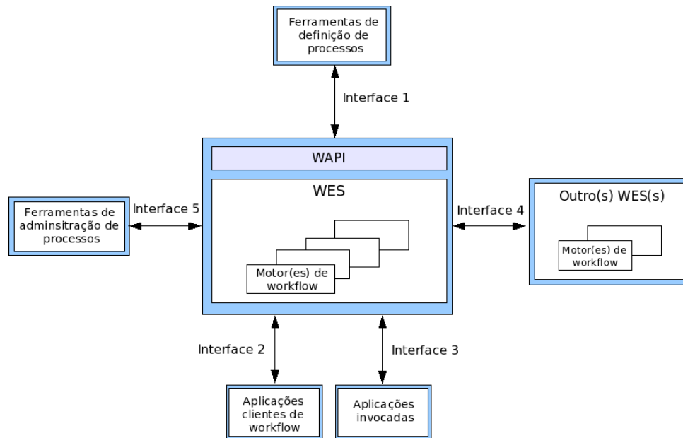
Figura 2.4: Modelo de referência da WfMC
