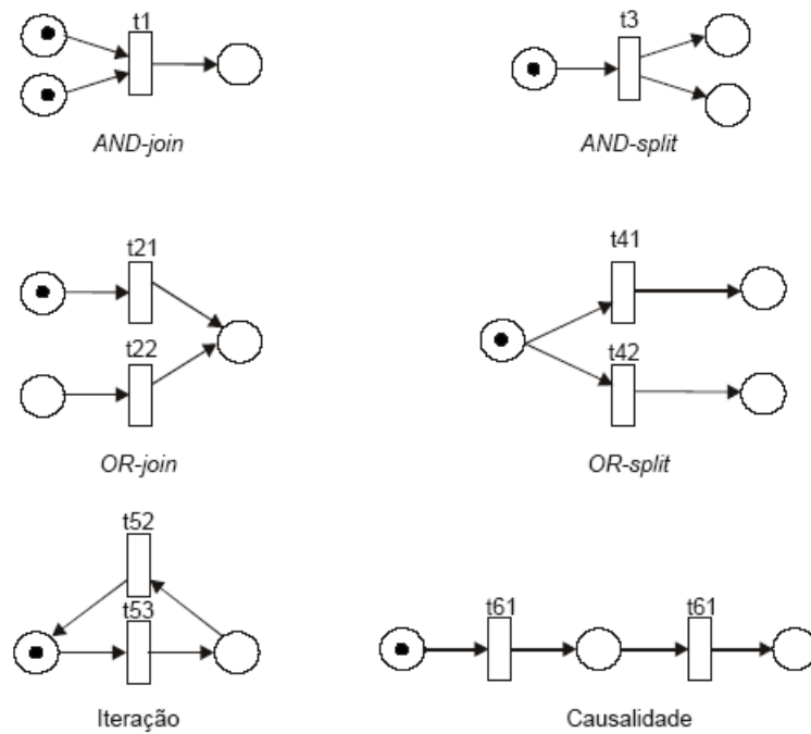
Figura 2.6: Tipos básicos de roteamento usando AND/OR e split/join por meio de Redes de Petri
