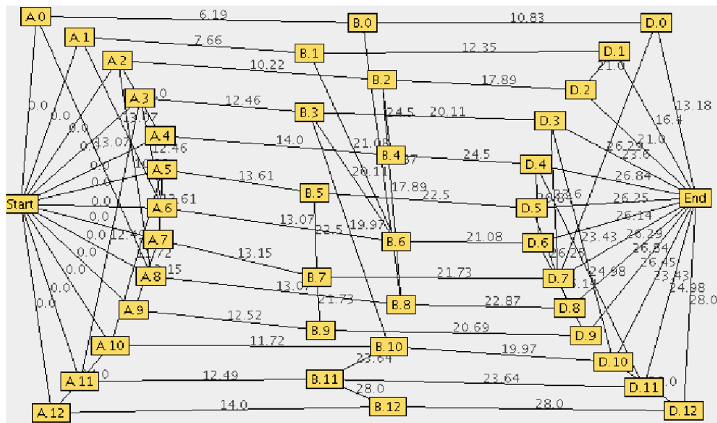
Figura 6.4: Grafo de escalonamento do Lambari
