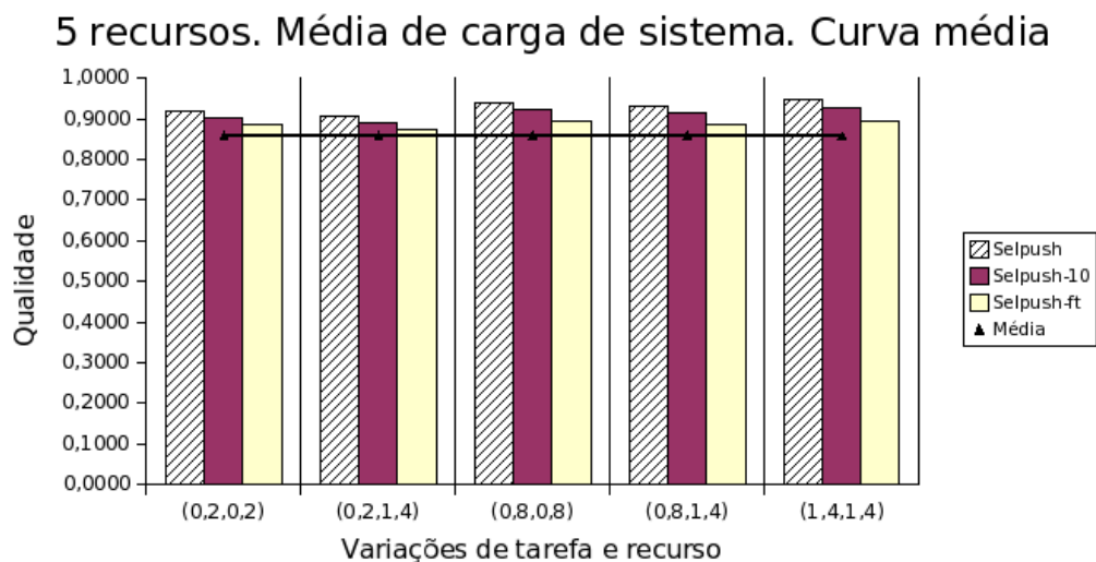
Figura 5.12: Comparação entre os mecanismos e a média de qualidade
