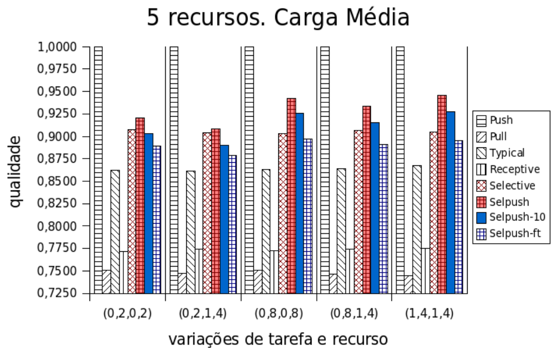
Figura 5.8: Variação de tempos com carga de sistema média na qualidade
