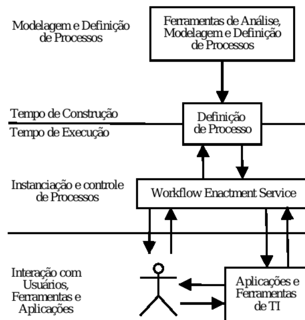
Figura 2.3: Relação entre as principais funções de um SGWf
