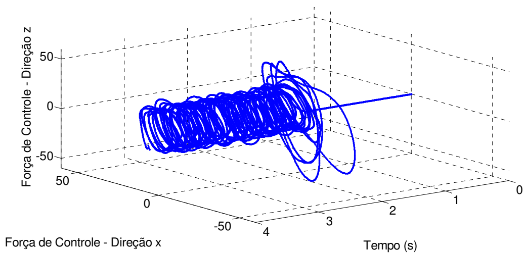
Figura D.10 – Força de Controle – Regime Permanente (1600rpm) – Lógica Fuzzy .
