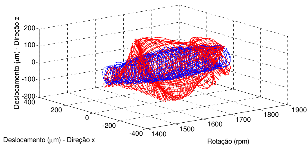
Figura D.7 – Órbita – Regime Transiente – Controle Ótimo.
