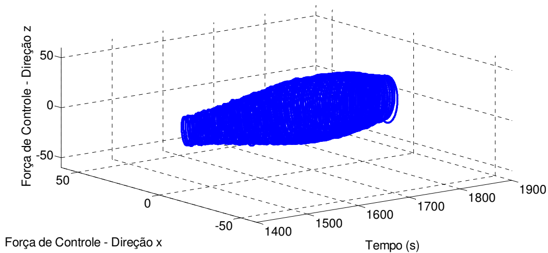
Figura D.4 – Força de Controle – Regime Transiente – Norma H_\infty .
