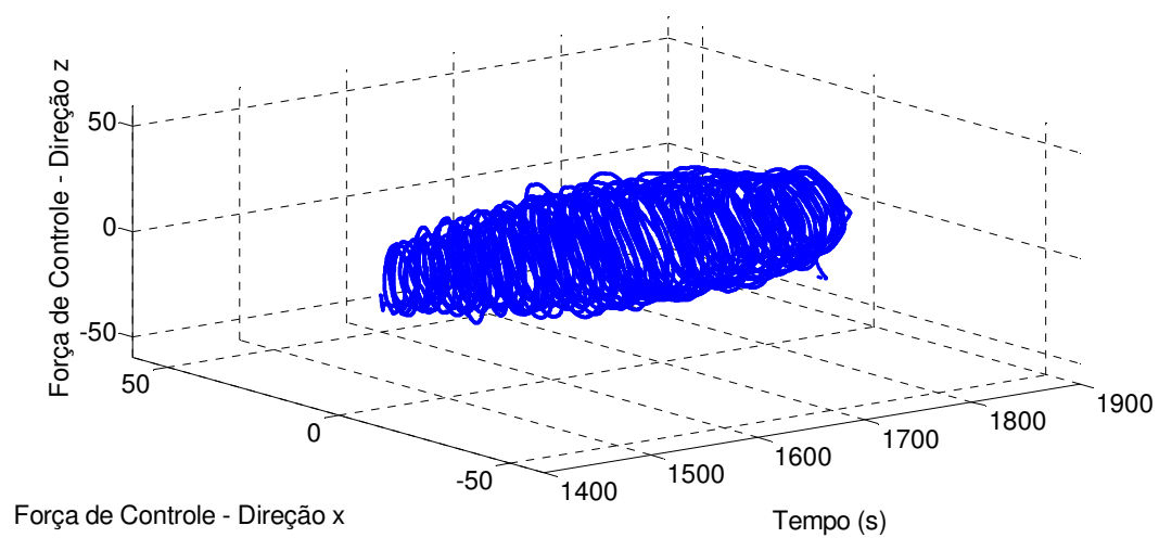
Figura D.12 – Força de Controle – Regime Transiente – Lógica Fuzzy .
