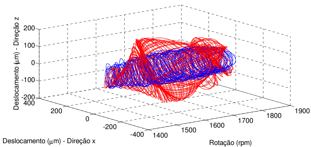
Figura D.11 – Órbita – Regime Transiente – Lógica Fuzzy .
