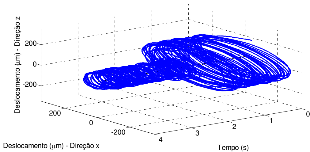
Figura D.9 – Órbita – Regime Permanente (1600rpm) – Lógica Fuzzy .
