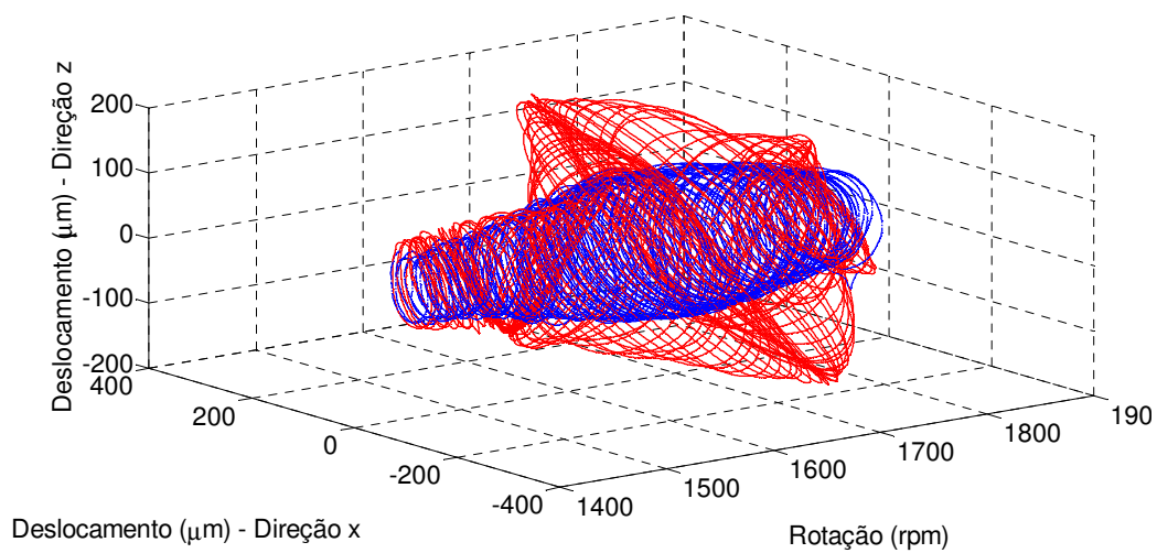
Figura D.3 – Órbita – Regime Transiente – Norma H_\infty .
