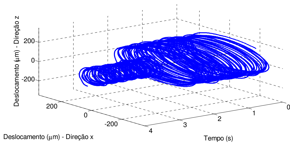
Figura D.5 – Órbita – Regime Permanente (1600rpm) – Controle Ótimo.
