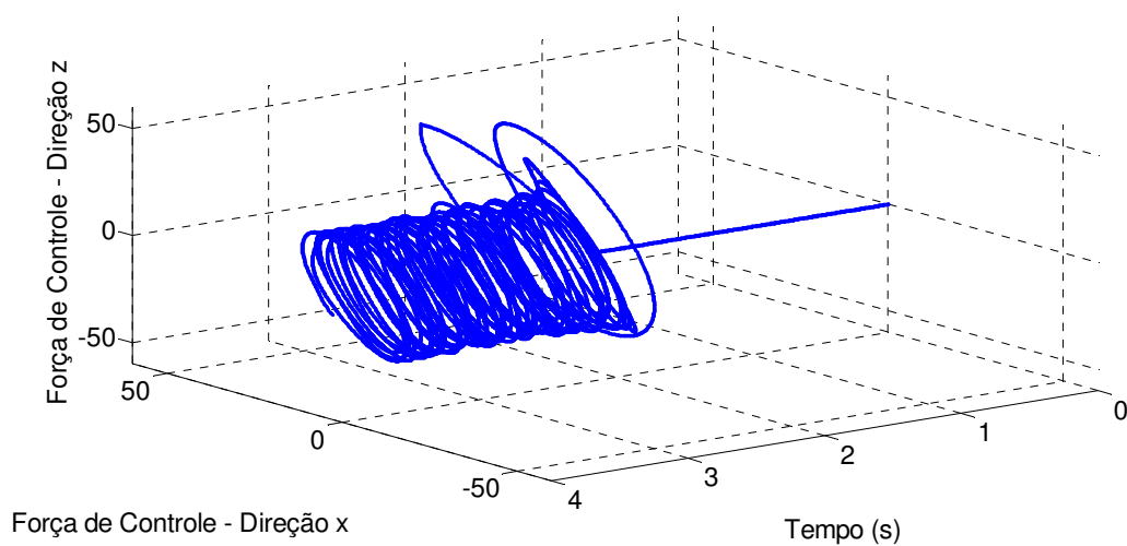
Figura D.6 – Força de Controle – Regime Permanente (1600rpm) – Controle Ótimo.
