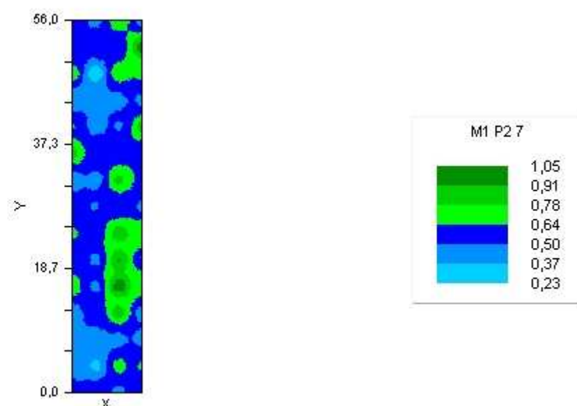
Figura 2D. Distribuição espacial do DMG (Diâmetro médio geométrico) dos agregados via úmida, para o sistema de manejo Irrigado com uso de Herbicida na profundidade de 20-40 cm, de Julho/Agosto de 2005.
