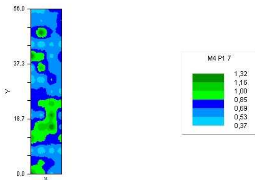
Figura 7D. Distribuição espacial do DMG (Diâmetro médio geométrico) dos agregados via úmida, para o sistema de manejo Sequeiro com uso de Herbicida na profundidade de 0-20 cm, de Julho/Agosto de 2005.
