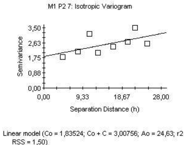
Figura 2A. Semivariograma do Carbono Orgânico Total (COT), para o sistema Irrigado com controle de plantas infestantes com uso de Herbicida na profundidade de 20-40 cm, de Julho/Agosto de 2005.
