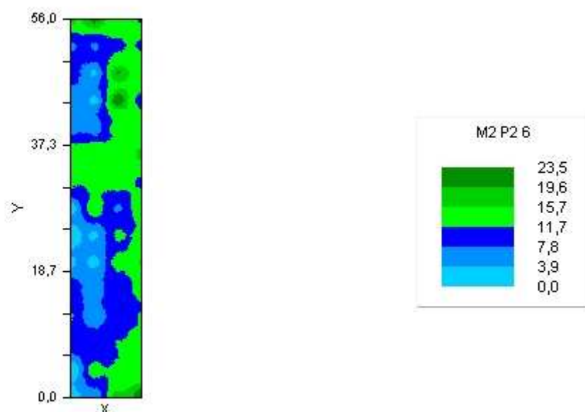
Figura 11B. Distribuição espacial do Carbono Orgânico Total (COT), para o sistema de Sequeiro com uso de Grade na profundidade de 0-20 cm, de Fevereiro/Março de 2006.
