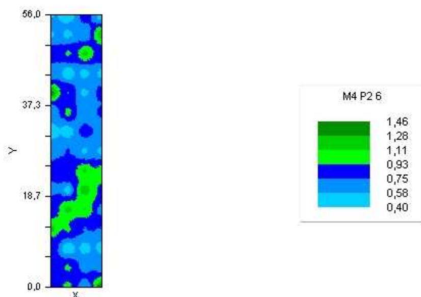
Figura 16D. Distribuição espacial do DMG (Diâmetro médio geométrico) dos agregados via úmida, para o sistema de manejo Sequeiro com uso de Herbicida na profundidade de 20-40 cm, de Fevereiro/Março de 2006.
