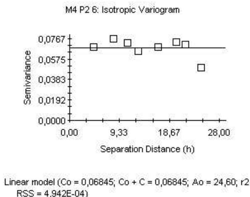
Figura 16C. Semivariograma de Diâmetro Médio Geométrico (DMG), para o sistema Sequeiro com controle de plantas infestantes com uso de Herbicida na profundidade de 20-40 cm, de Fevereiro/Março de 2006.
