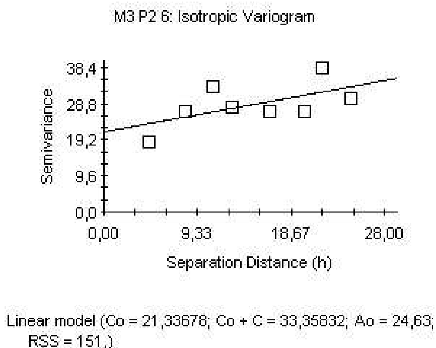
Figura 13A. Semivariograma do Carbono Orgânico Total (COT), para o sistema Irrigado com controle de plantas infestantes com uso de Grade na profundidade de 0-20 cm, de Fevereiro/Março de 2006.
