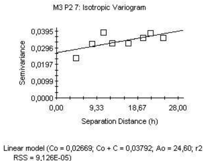
Figura 6C. Semivariograma de Diâmetro Médio Geométrico (DMG), para o sistema Irrigado com controle de plantas infestantes com uso de Grade na profundidade de 20-40 cm, de Julho/Agosto de 2005.
