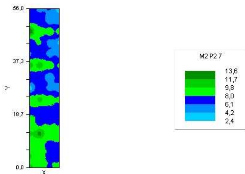
Figura 4B. Distribuição espacial do Carbono Orgânico Total (COT), para o sistema de Sequeiro com uso de Grade na profundidade de 20-40 cm, de Julho/Agosto de 2005.
