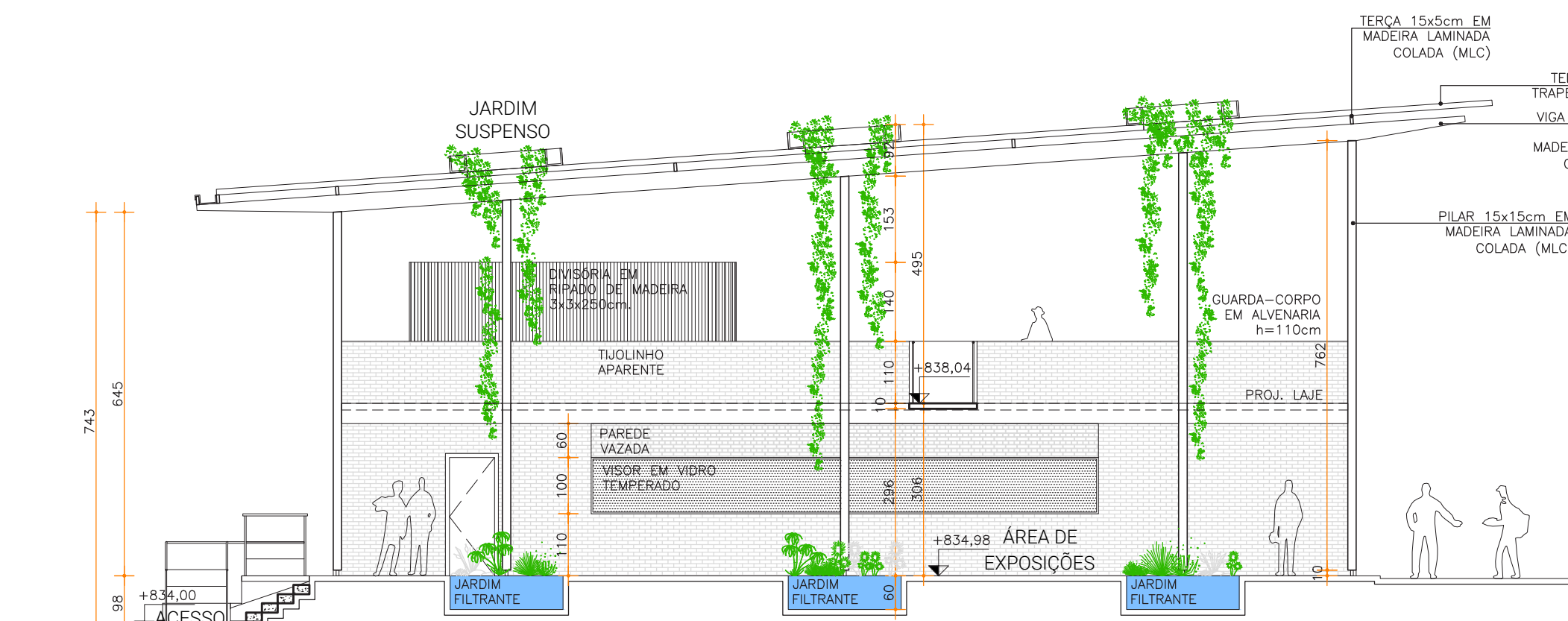
CORTE CC 1:100
