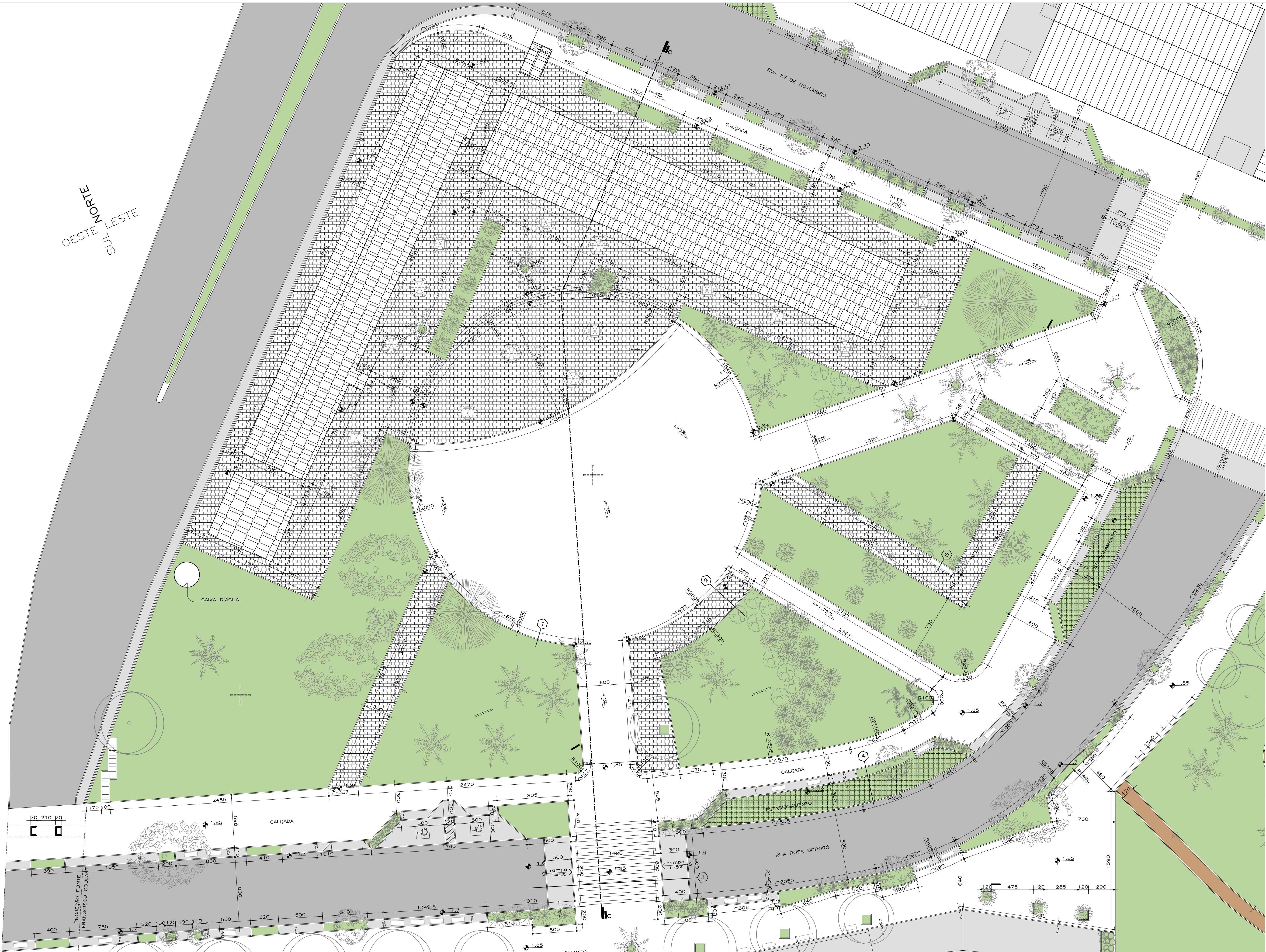
PLANTA CASARIO ESC. 1:200
