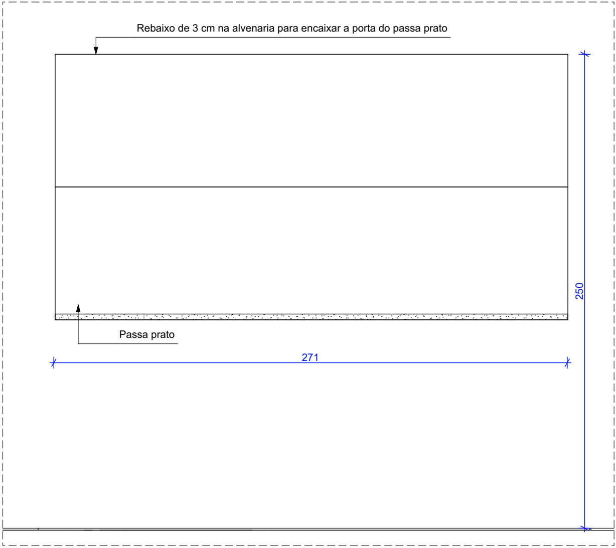
Det.1 Det em vista passa prato com fechamento
