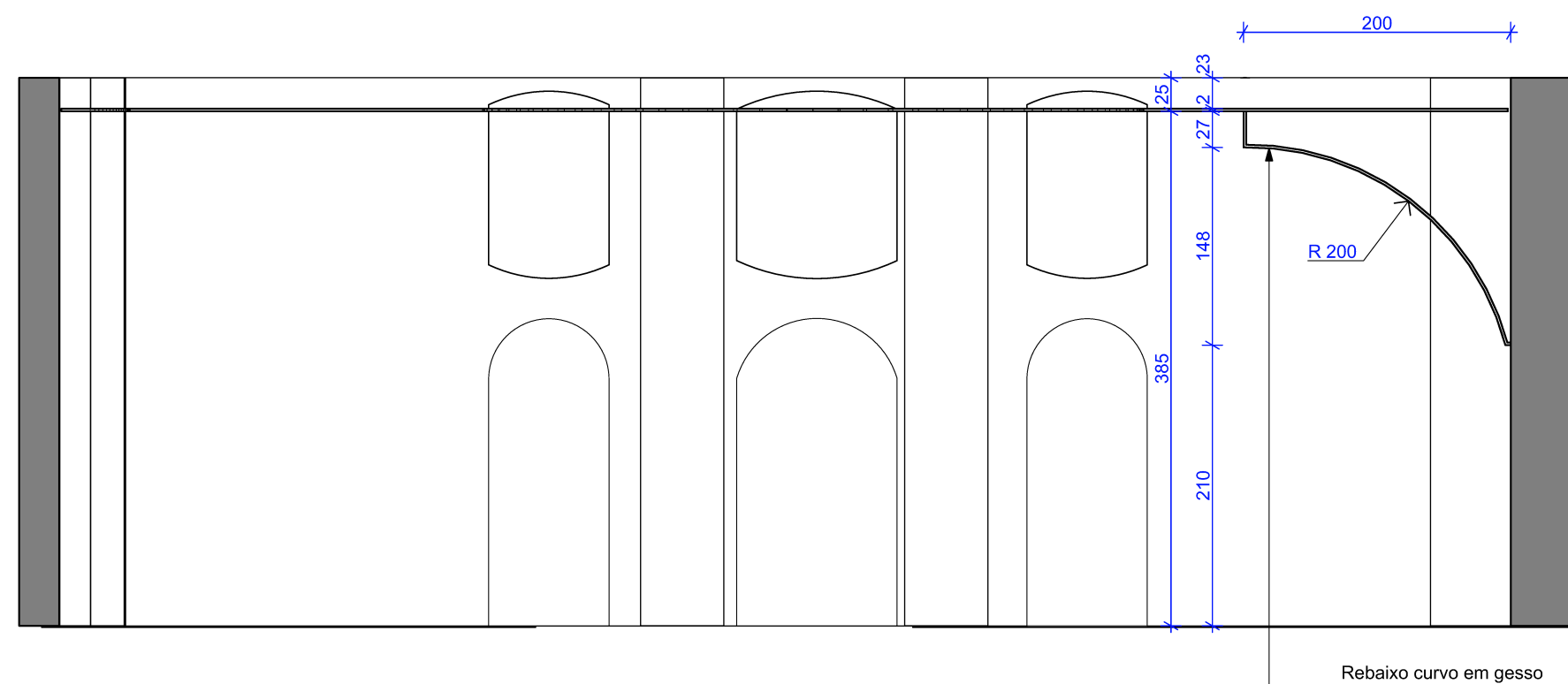
12. Corte GG Escala: 1:50
