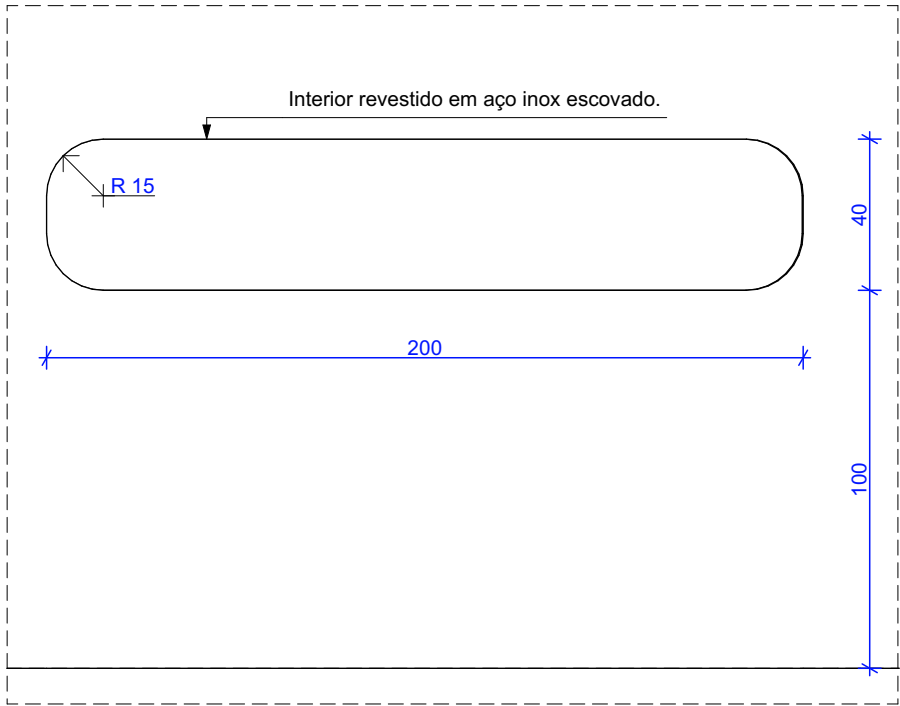
Det.2 Detalhe em vista passa prato cozinha
