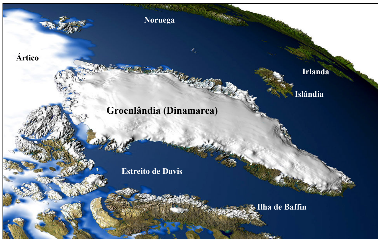
Figura 3 - Imagem da Groenlândia – NASA.
