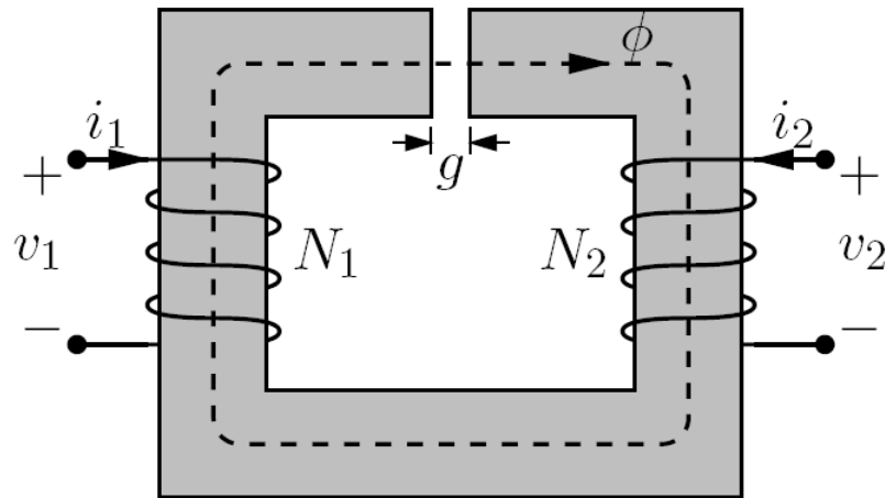
Figura 1.7: Transformador
