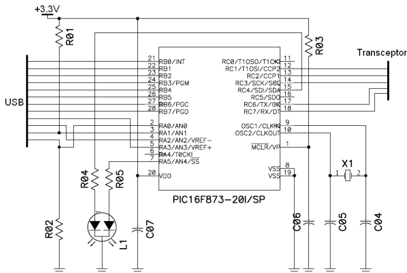
Figura 3.14: Diagrama elétrico do circuito de controle do sistema de recepção
