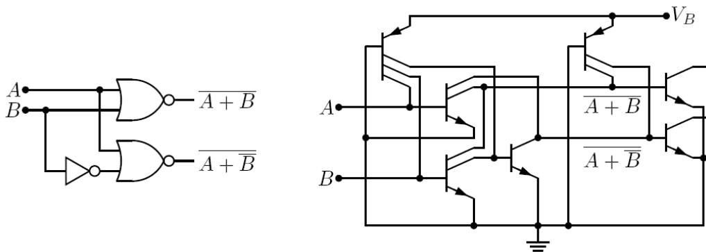
Figura 1.9: Portas Lógicas
