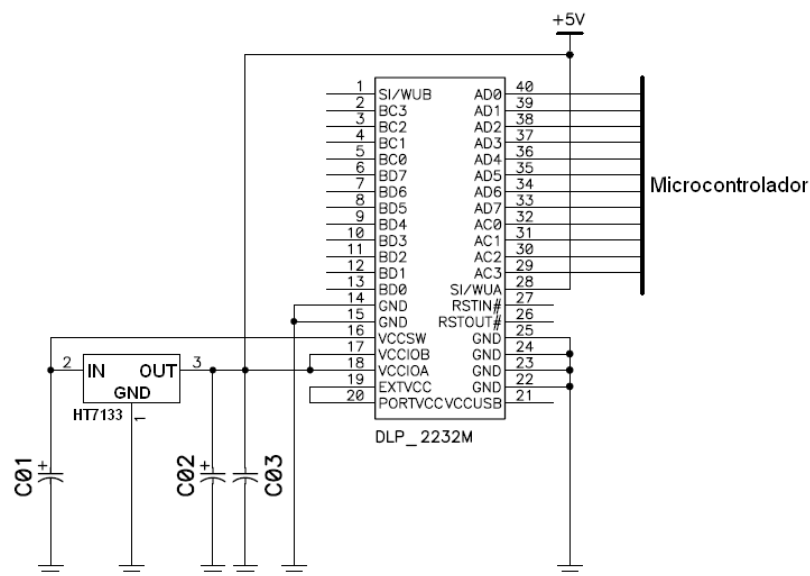
Figura 3.15: Diagrama elétrico de conexão do módulo USB
