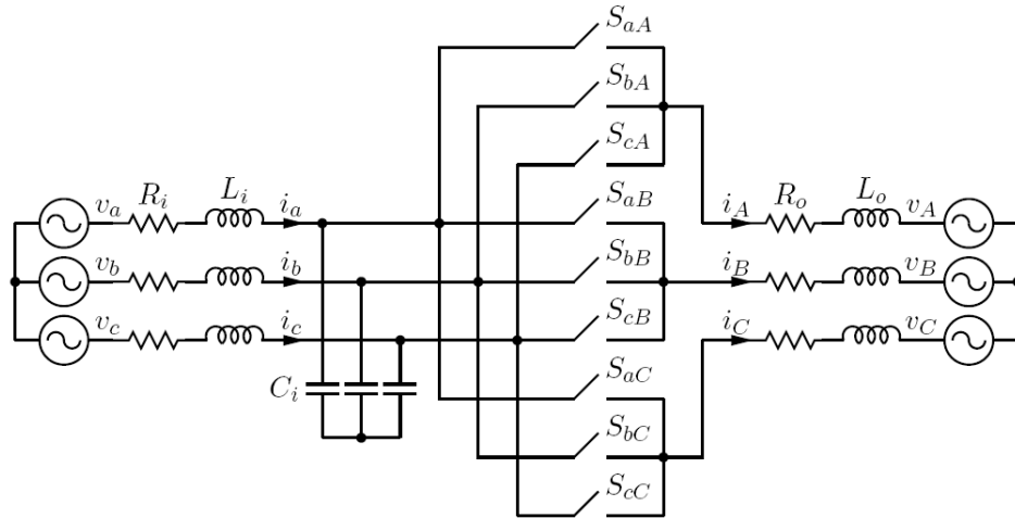
Figura 1.15: Grupo Gerador-Motor
