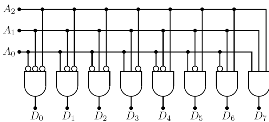
Figura 1.18: Decodificador lógico
