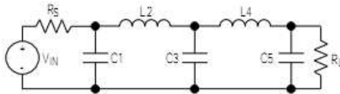
Figura 3.7: Modelo do filtro utilizado
