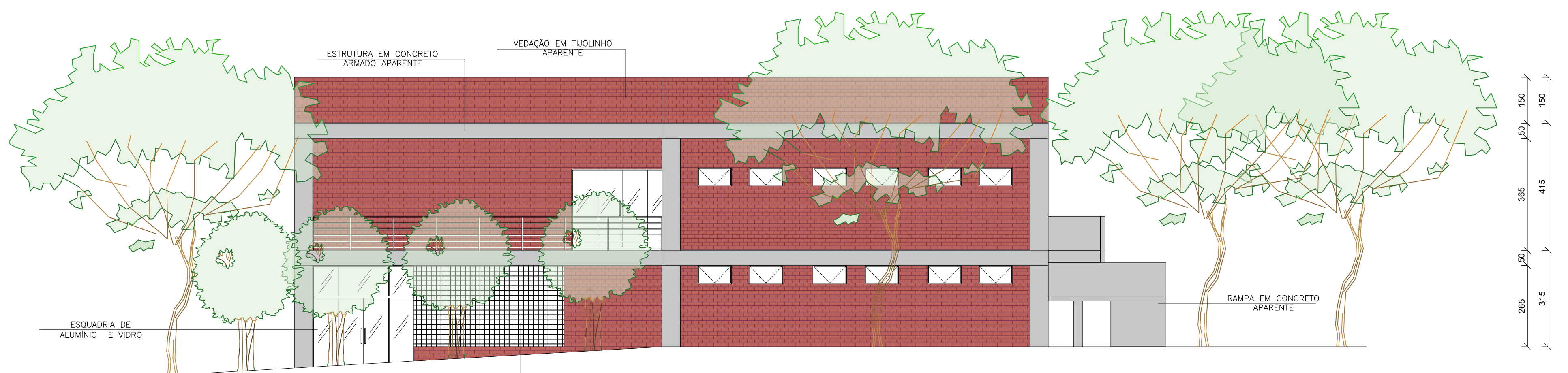
ELEVÇÃO 02 1:100
