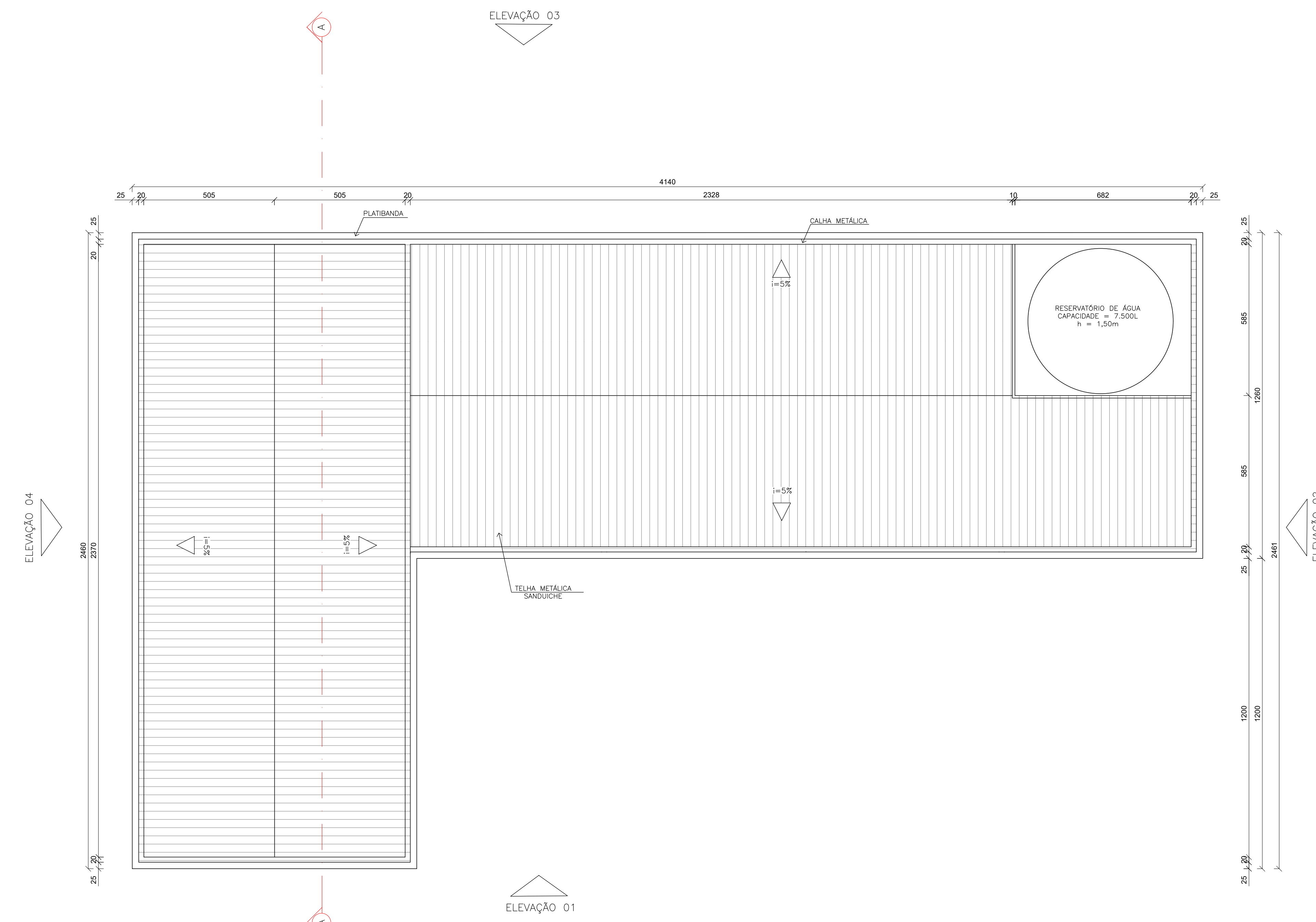
COBERTURA 1:100
