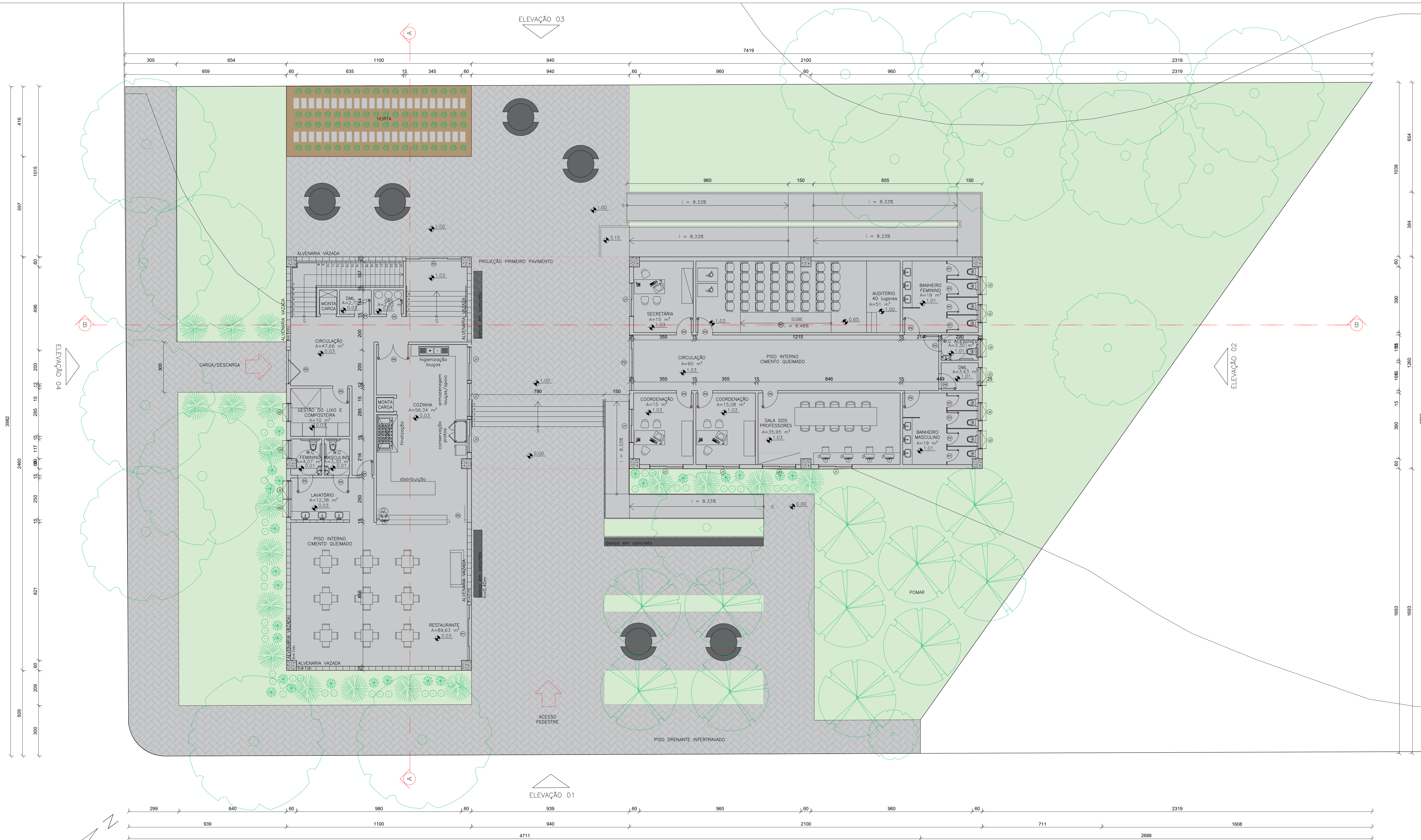
IMPLANTAÇÃO/TERREO 1:100
