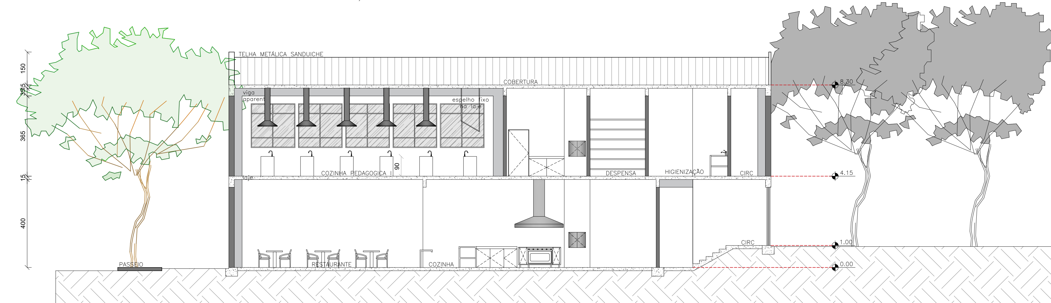
CORTE AA 1:100
