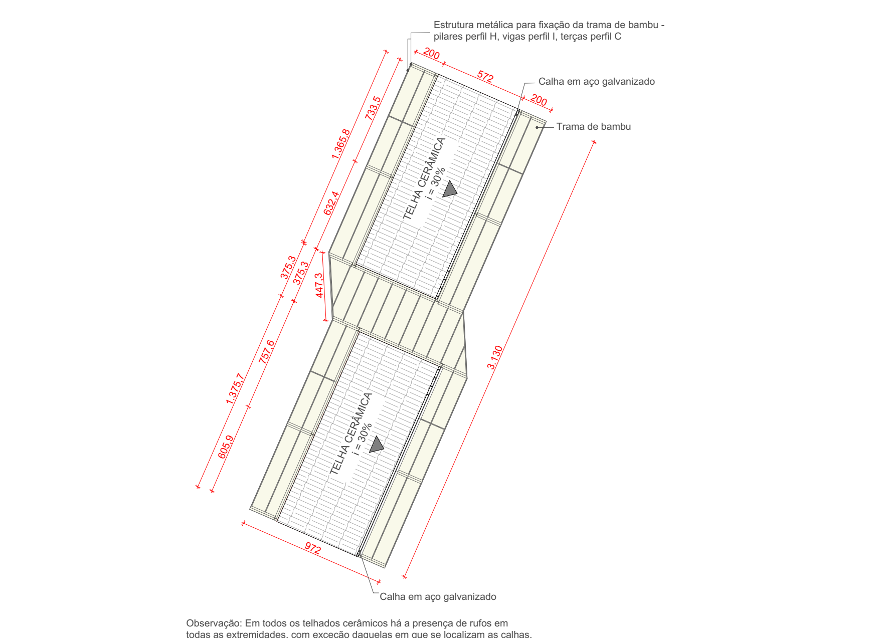
8 Planta de Cobertura Setor de Esporte Escala: 1:250
