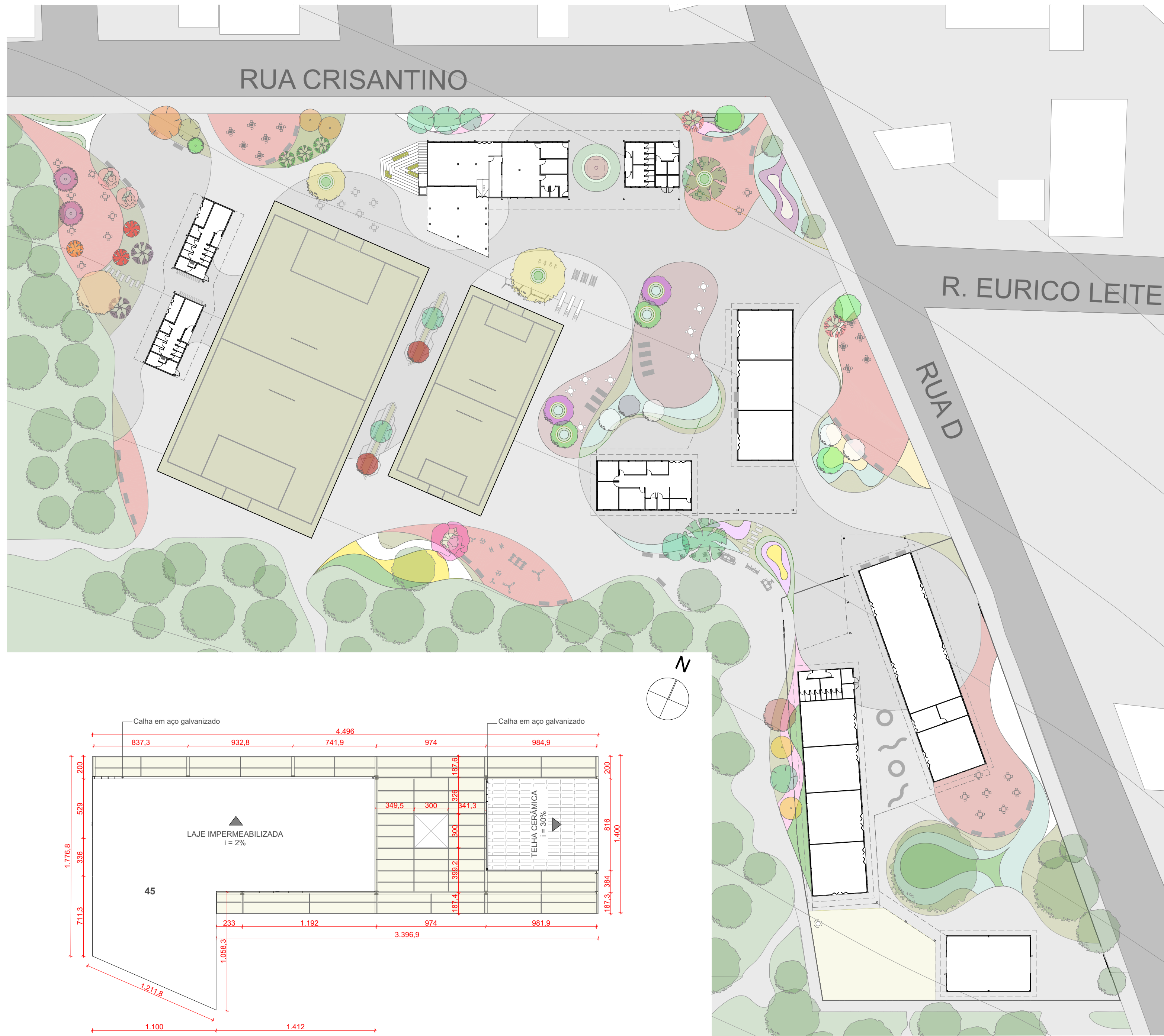
7 Planta de Cobertura Setor Alimentação e Banheiros Escala: 1:250
