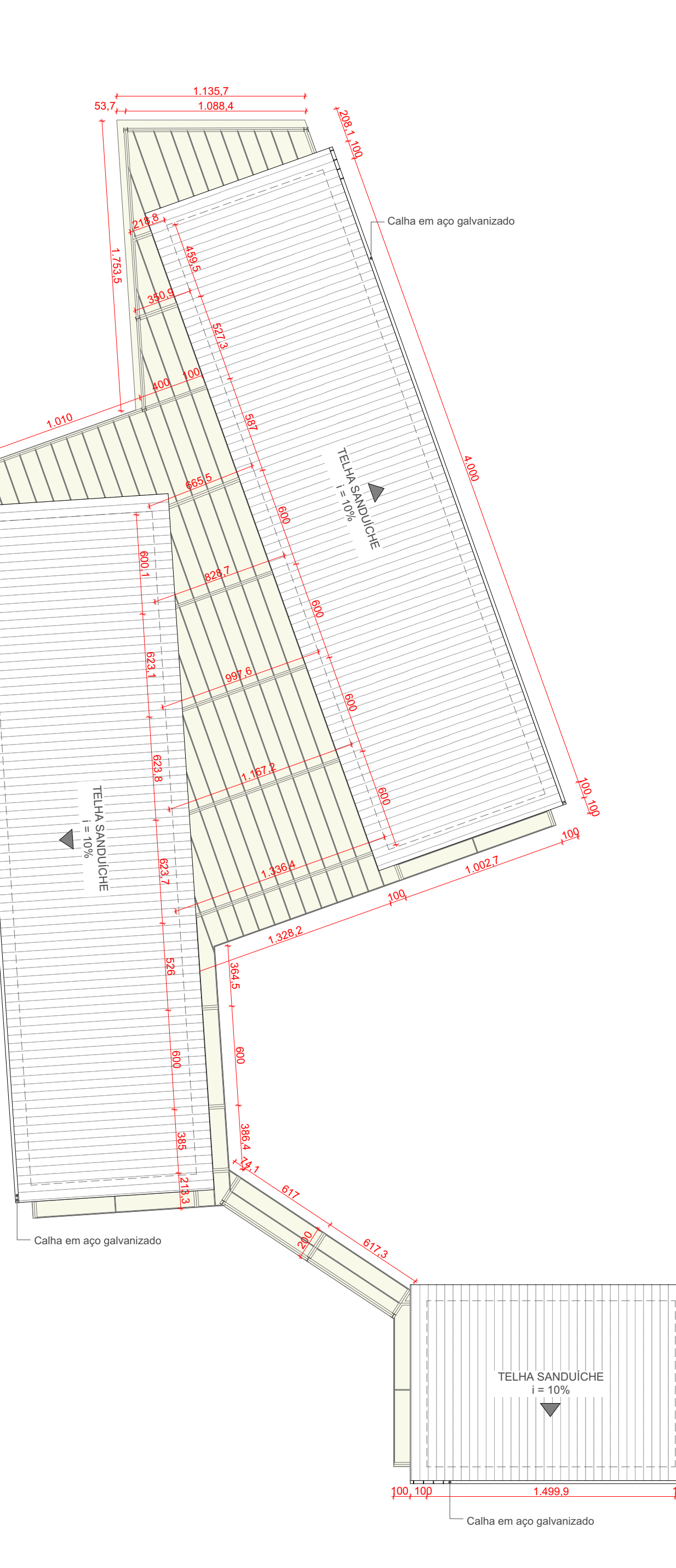
10 Planta de Cobertura Setor Técnico/Formativo Escala: 1:250
