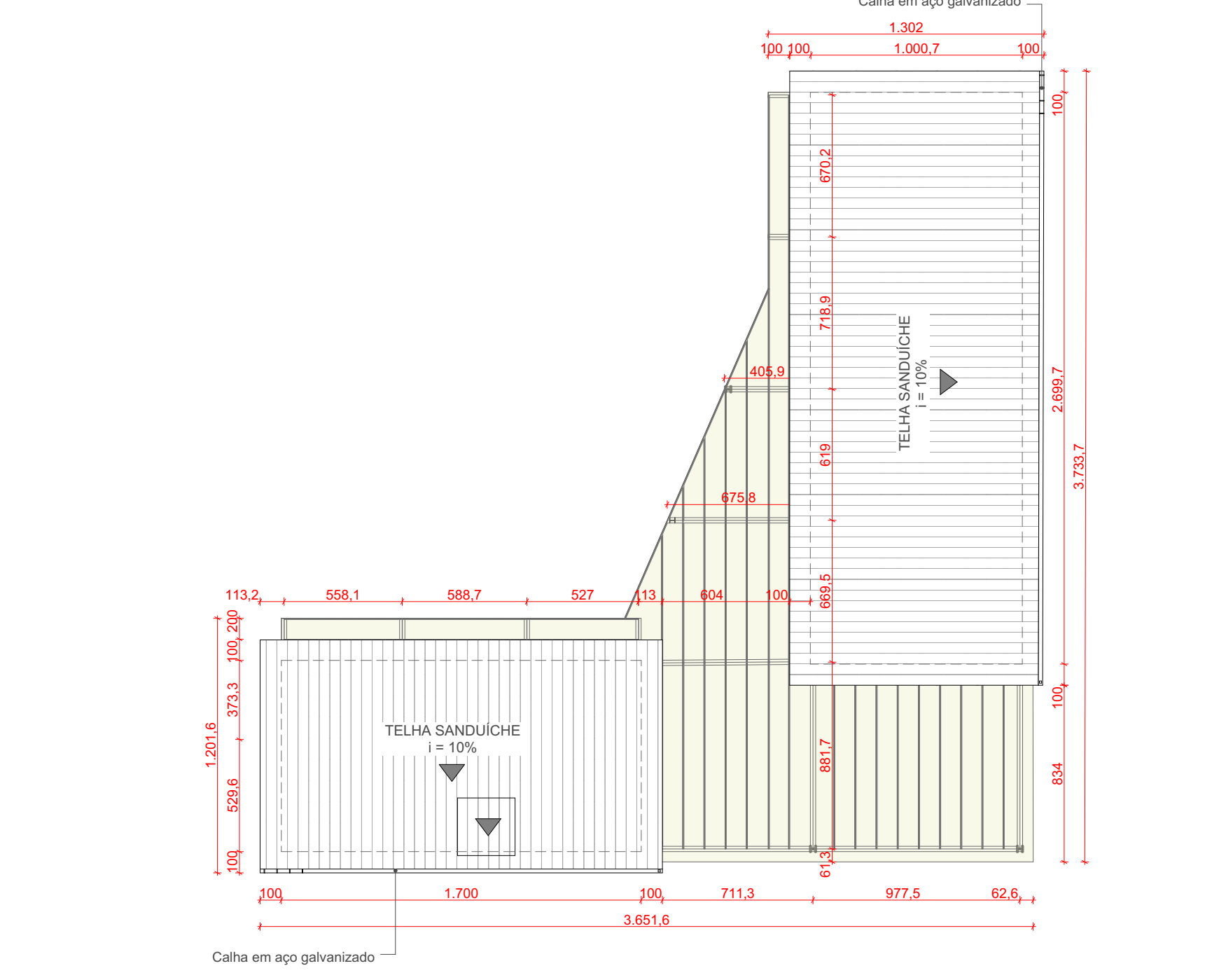
9 Planta de Cobertura Setores Administrativo e Cultural Escala: 1:250
