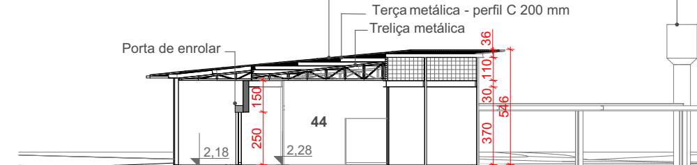
15 Corte 04 Escala: 1:250
