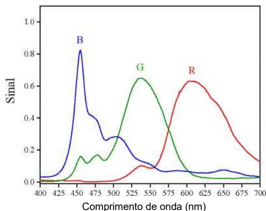
Figura 12. Resposta efetiva dos sensores: Resposta obtida a partir da multiplicação do sinal da resposta espectral pelo sinal obtido do espectro de emissão dos LED's. a) AS7341; b) AS7262; c) TCS34725
