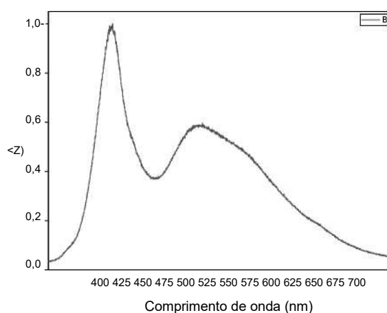
Figura 11. Espectro de emissão do LED branco de alto brilho presente nos sensores de cor
