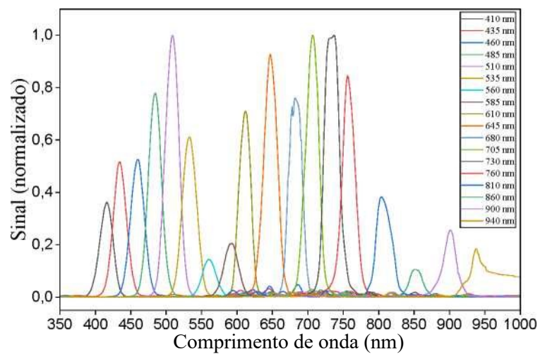
Figura 20. Resposta espectral do sensor AS7265x
