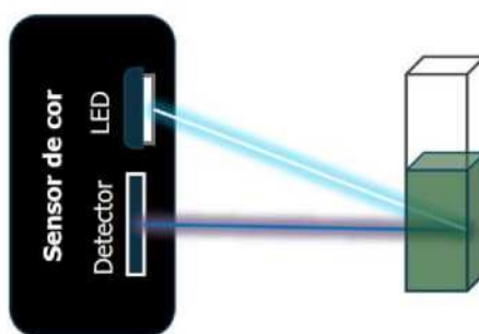
Figura 3. Esquema representativo do funcionamento dos sensores de cor.
