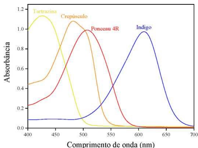
Figura 25. Espectros de absorção de soluções aquosas dos corantes amarelo tartrazina ( 50 \text{ mmol L}^{-1} ), amarelo crepúsculo ( 45 \text{ mmol L}^{-1} ), vermelho ponceau 4R ( 58 \text{ mmol L}^{-1} ), e azul indigo ( 90 \text{ mmol L}^{-1} ).
