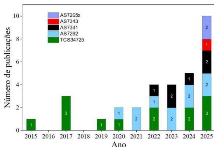
Figura 5. Evolução anual do número de publicações relacionadas aos sensores espectrais AS7343, AS7265x, AS7341, AS7262 e TCS34725, no período de 2015 a 2025.
