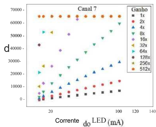
Figura 22. Sinais obtidos em função da corrente aplicada ao LED (5-100 mA) em diferentes ganhos (1 a 512X) para otimização e seleção dos parâmetros para cada um dos canais disponíveis no sensor
