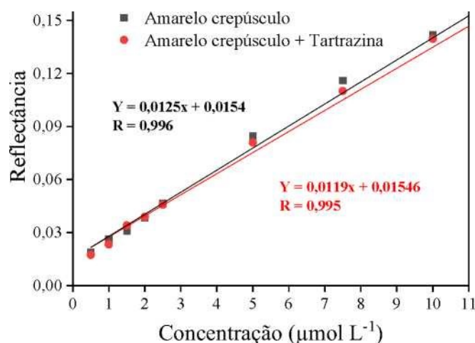
Figura 27. Curvas de calibração para quantificação do corante AC. Em preto, apenas o corante de interesse. E em vermelho, na presença do corante AT em mesmas concentrações
