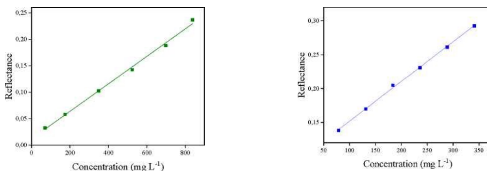
Figura 42. Curvas de calibração obtidas para cada um dos corantes avaliados: Amarelo tartrazina, vermelho Bordeaux, azul índigo e verde de Bromocresol.
