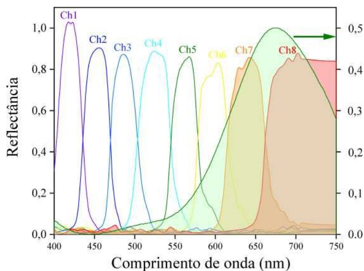
Figura 44. Espectro de absorção do indophenol (verde) em sobreposição com a resposta efetiva do sensor AS7341
