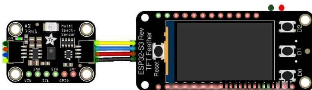
Figura 29. Esquema representativo da ligação do sensor AS7341 com o microcontrolador ESP 32-S3
