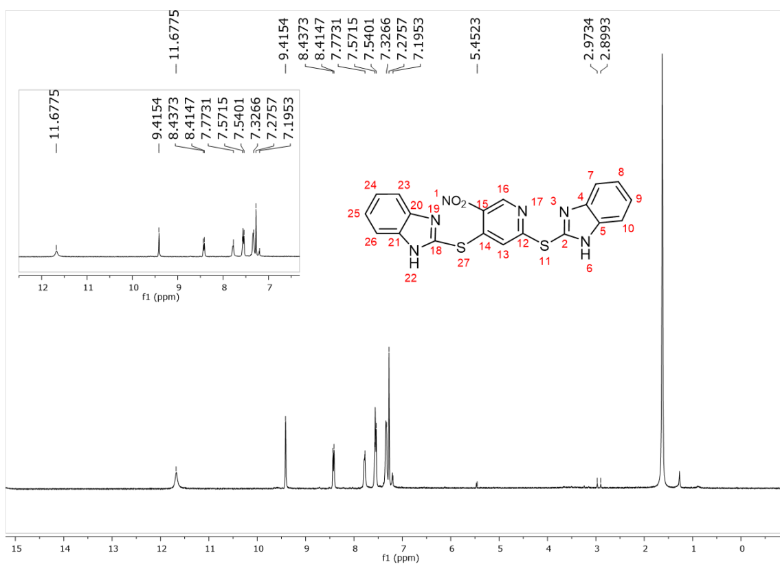
Figura 23. Espectro de RMN de ^1\text{H} de 6 (400MHZ, \text{CDCl}_3 )
