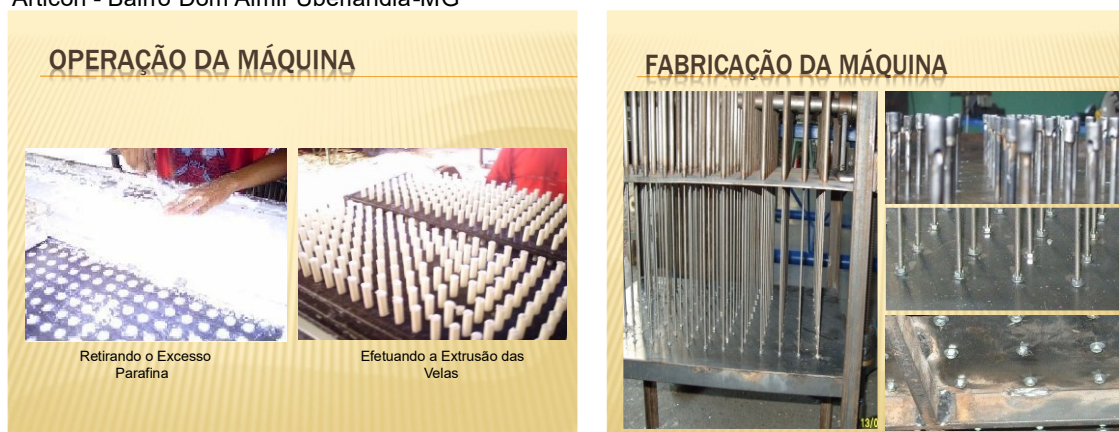
Figura 13 – Máquina extrusora de velas feita pelos estudantes da Engenharia Mecânica - Projeto Articon - Bairro Dom Almir Uberlândia-MG
