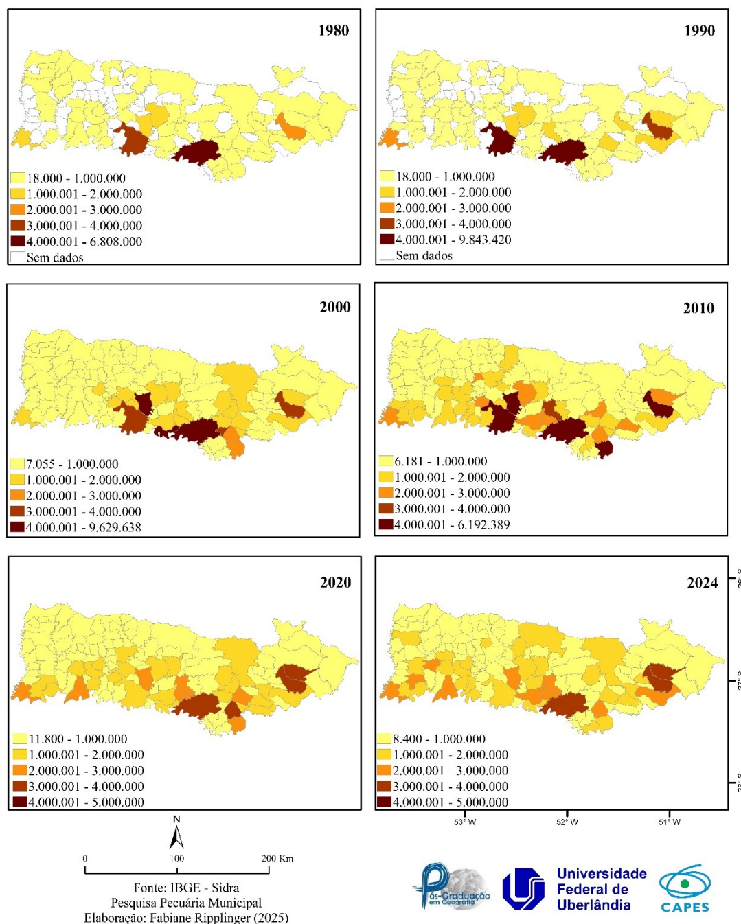
Figura 8 - Galináceos: Efetivo (cabeças) por município no Oeste Catarinense
