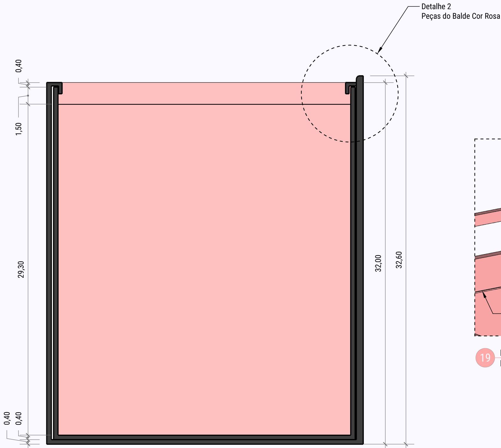
18 Corte BB - Balde Destampado Escala 1:2
