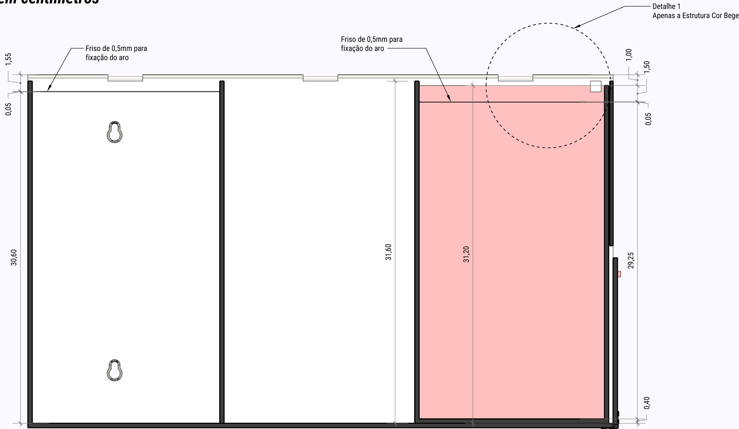
17 Corte AA Balde Destampado
