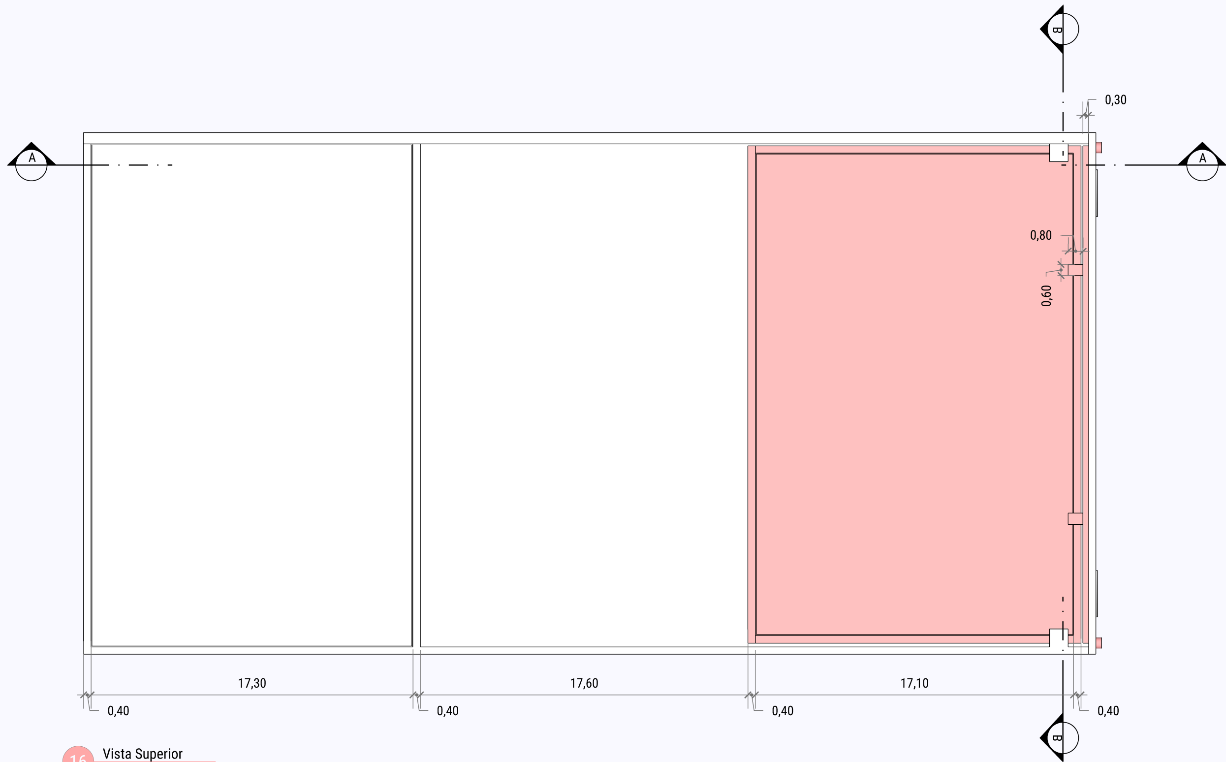
16 Vista Superior Balde Destampado
