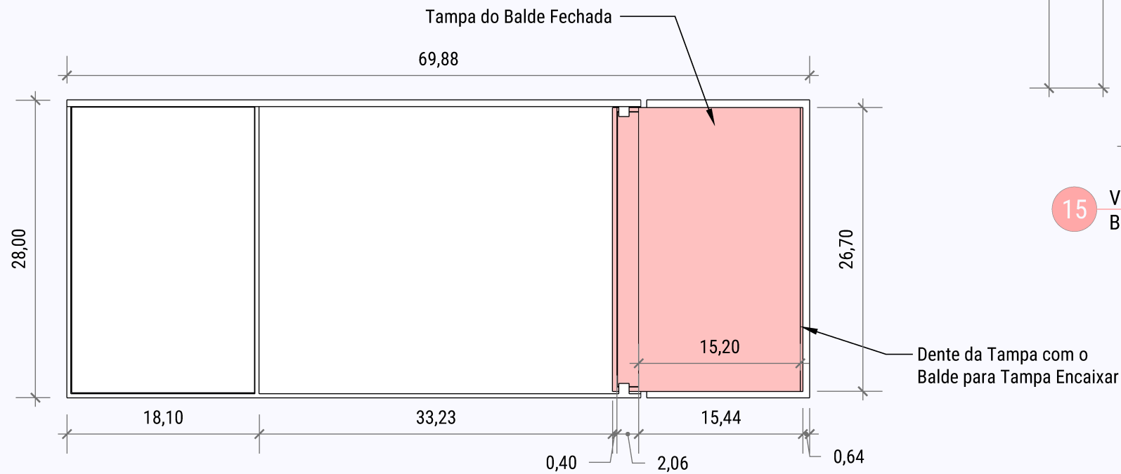
14 Vista Superior Balde Tampado
