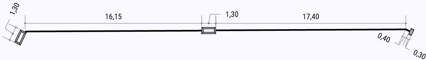
22 Limitador de Movimento com Dois Elos Escala 1:2
