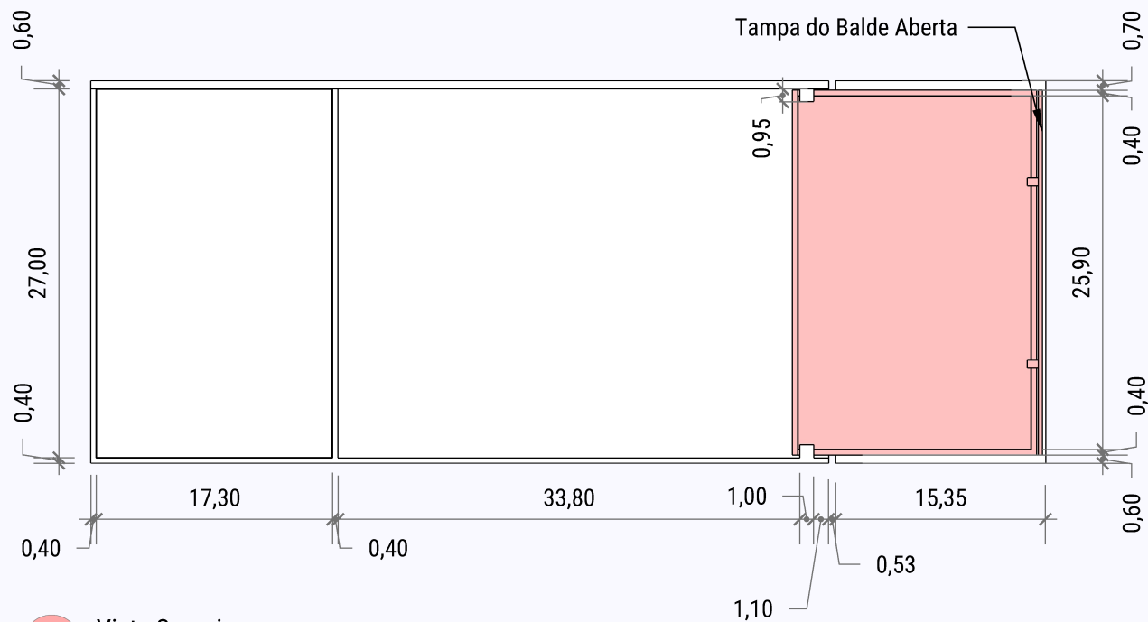
13 Vista Superior Balde Destampado
