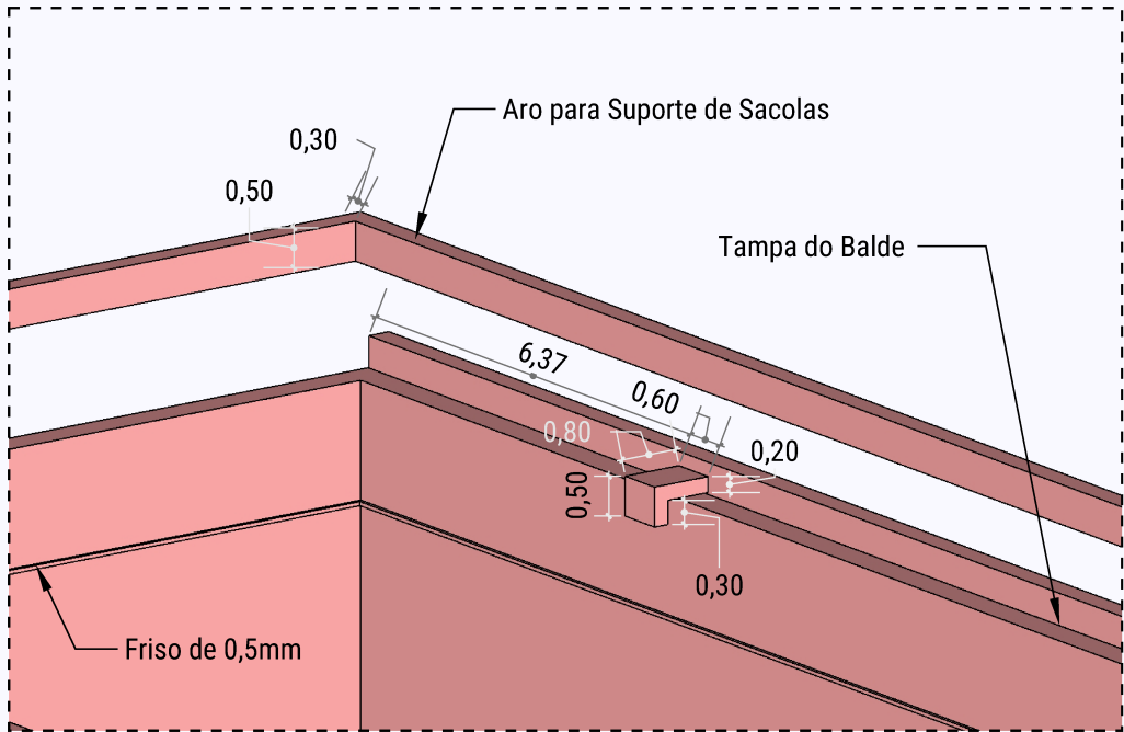
19 Detalhe 2 Escala 1:1
