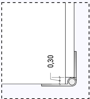
24 Dobradiça Vista Lateral Direita Escala 1:1
