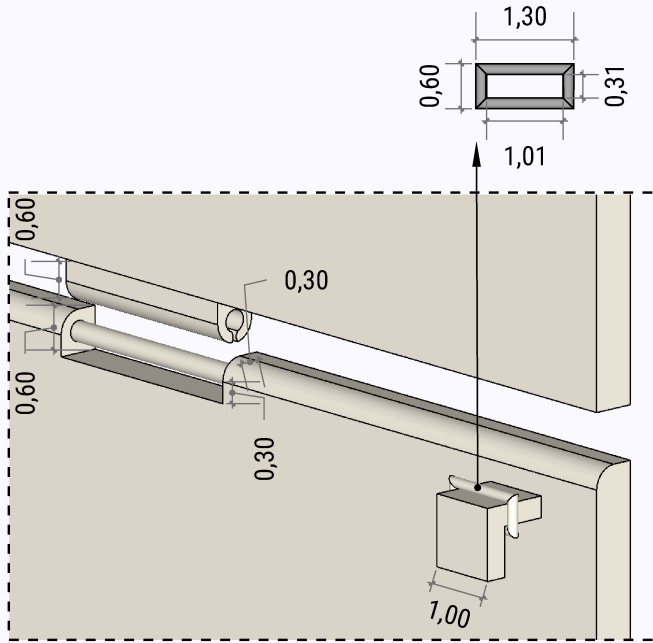
21 Detalhe 1 Explodido Escala 1:1
