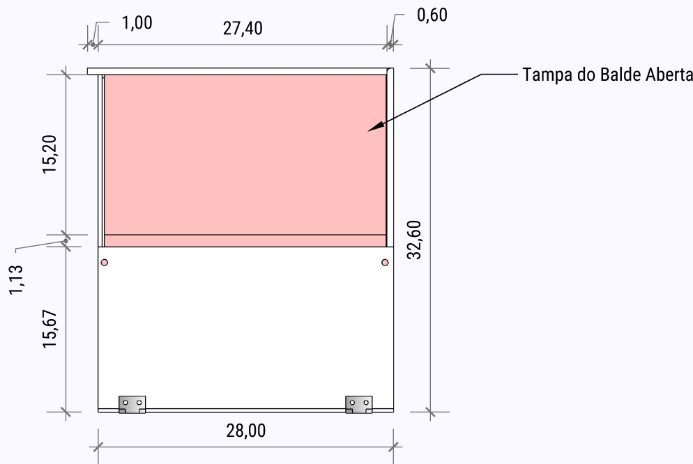
12 Vista Lateral Direita
