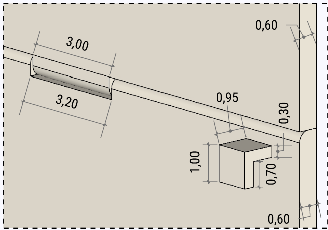
20 Detalhe 1 Escala 1:1
