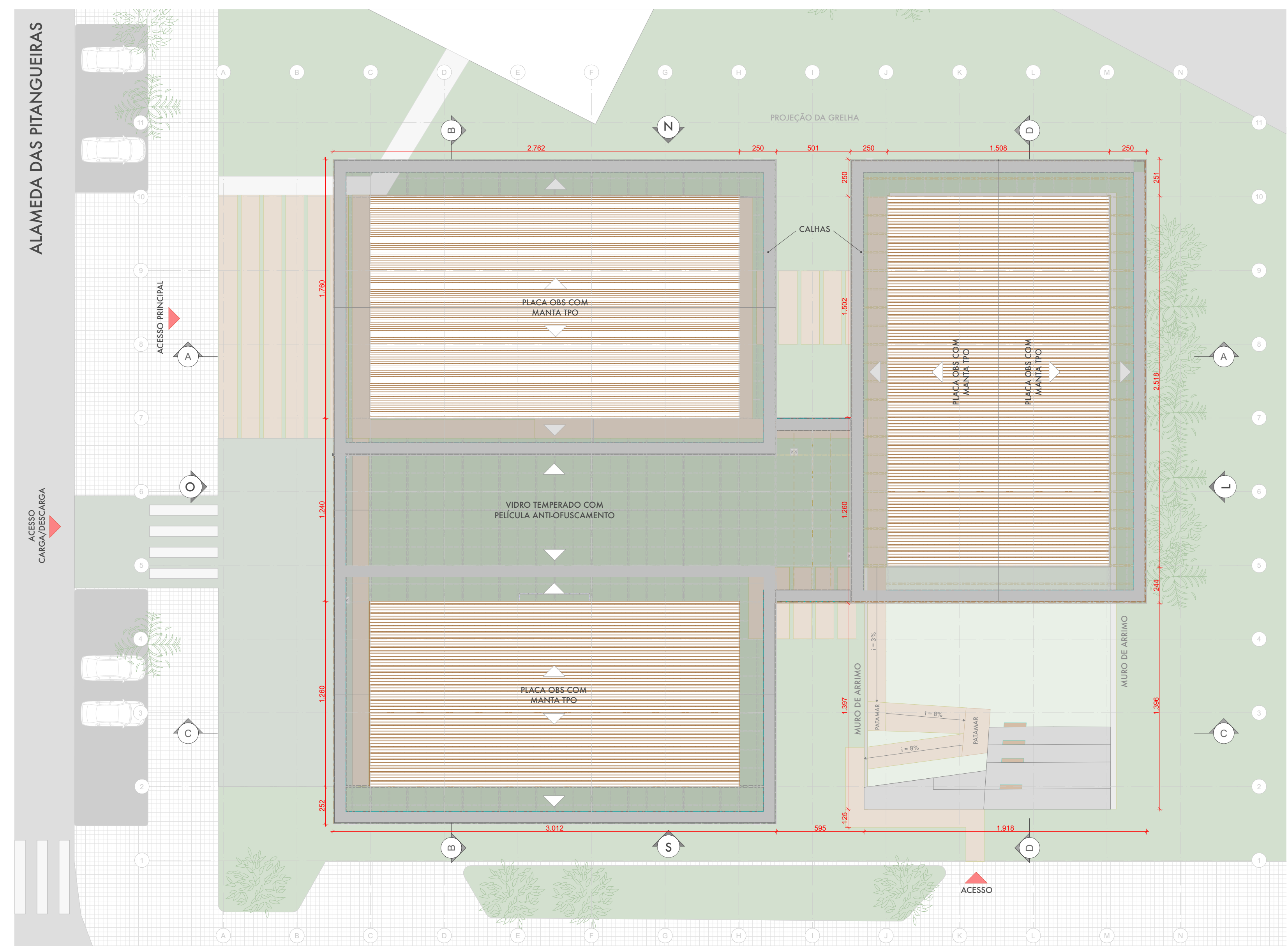
08 | PLANTA DE COBERTURA 1:200
