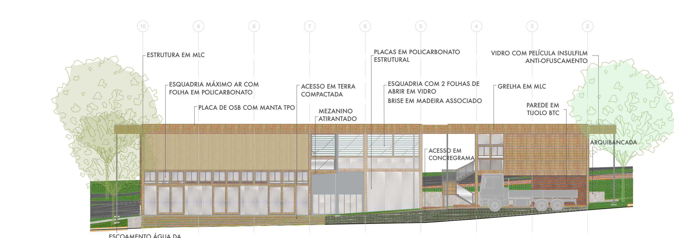
12 | ELEVÇÃO OESTE 1:200
