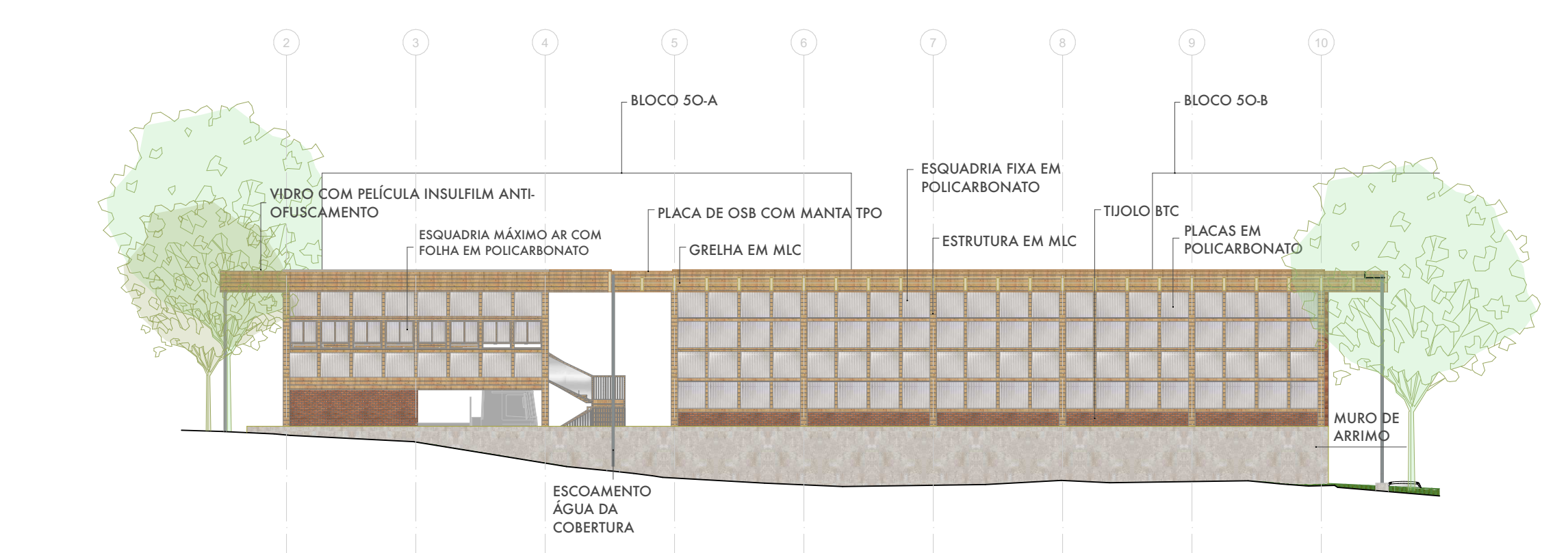
10 | ELEVÇÃO LESTE 1:200
