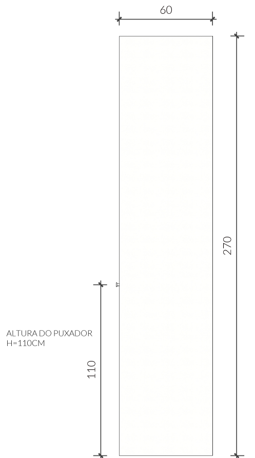
09 VISTA LATERAL PARTE 02 - GUARDA-ROUPAS Esc: 1/25
