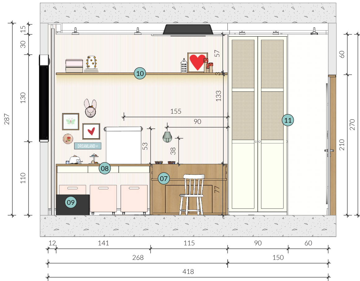
01 CORTE A - VISTA FRONTAL Esc: 1/35
