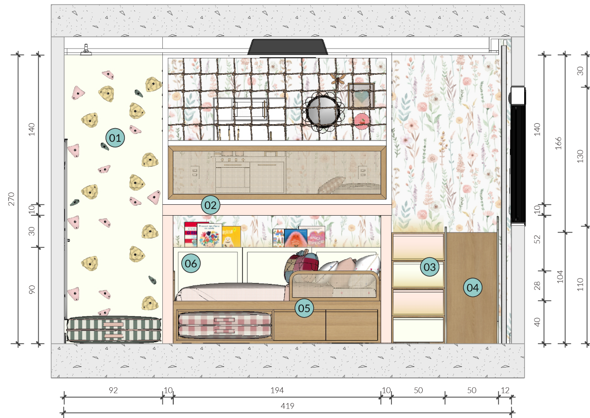
03 CORTE C - VISTA FRONTAL Esc: 1/35
