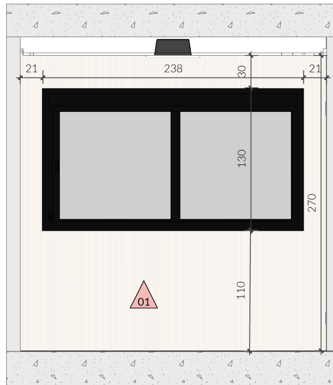
CORTE D - REVESTIMENTO
