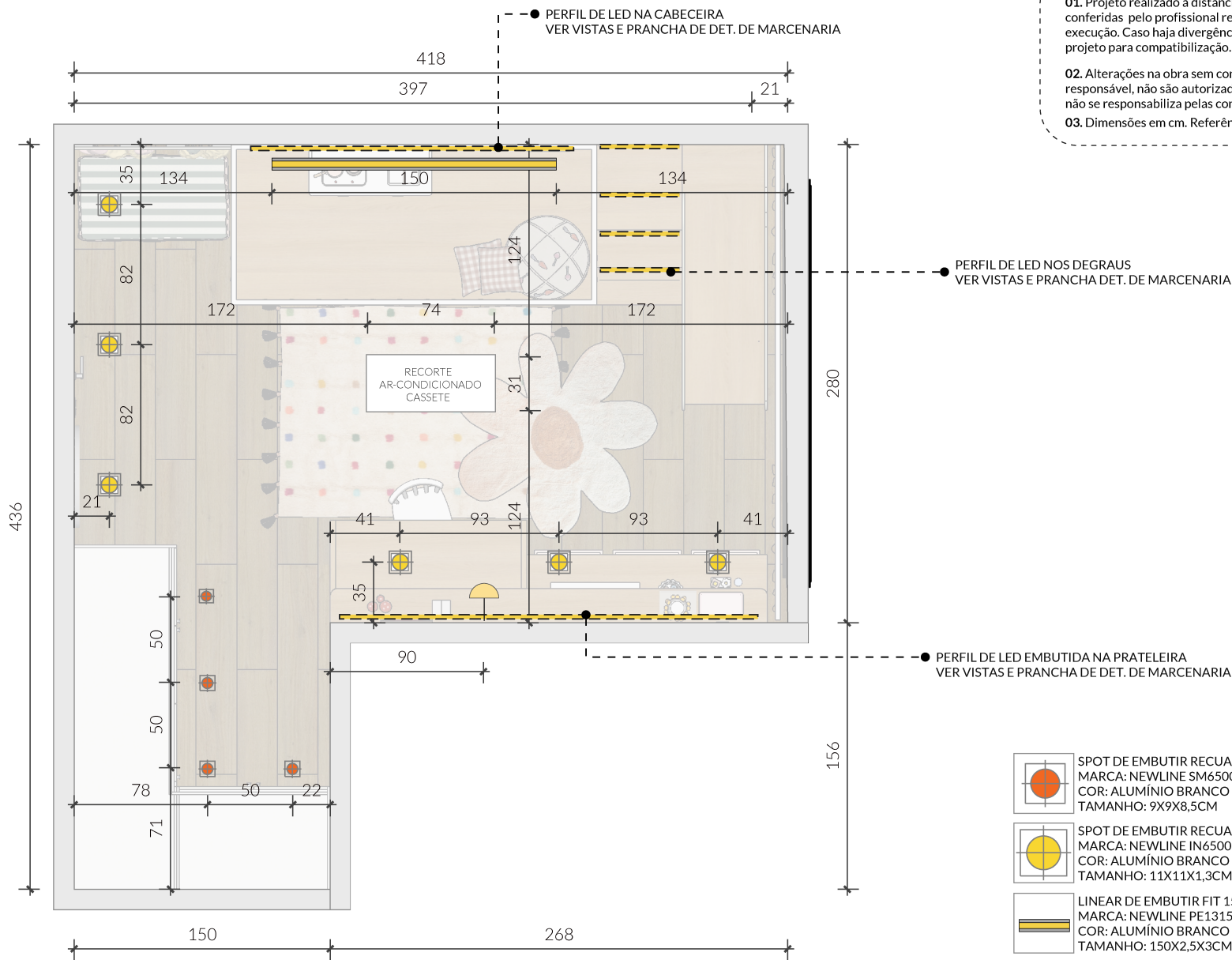
01 VISTA SUPERIOR GESSO QUARTO Esc: 1/35
