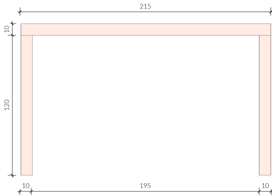
07 VISTA ISOLADA FRONTAL MEZANINO Esc: 1/20
