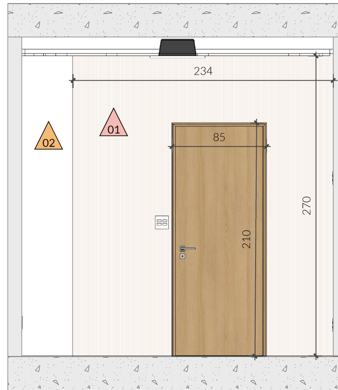
CORTE B - REVESTIMENTO
