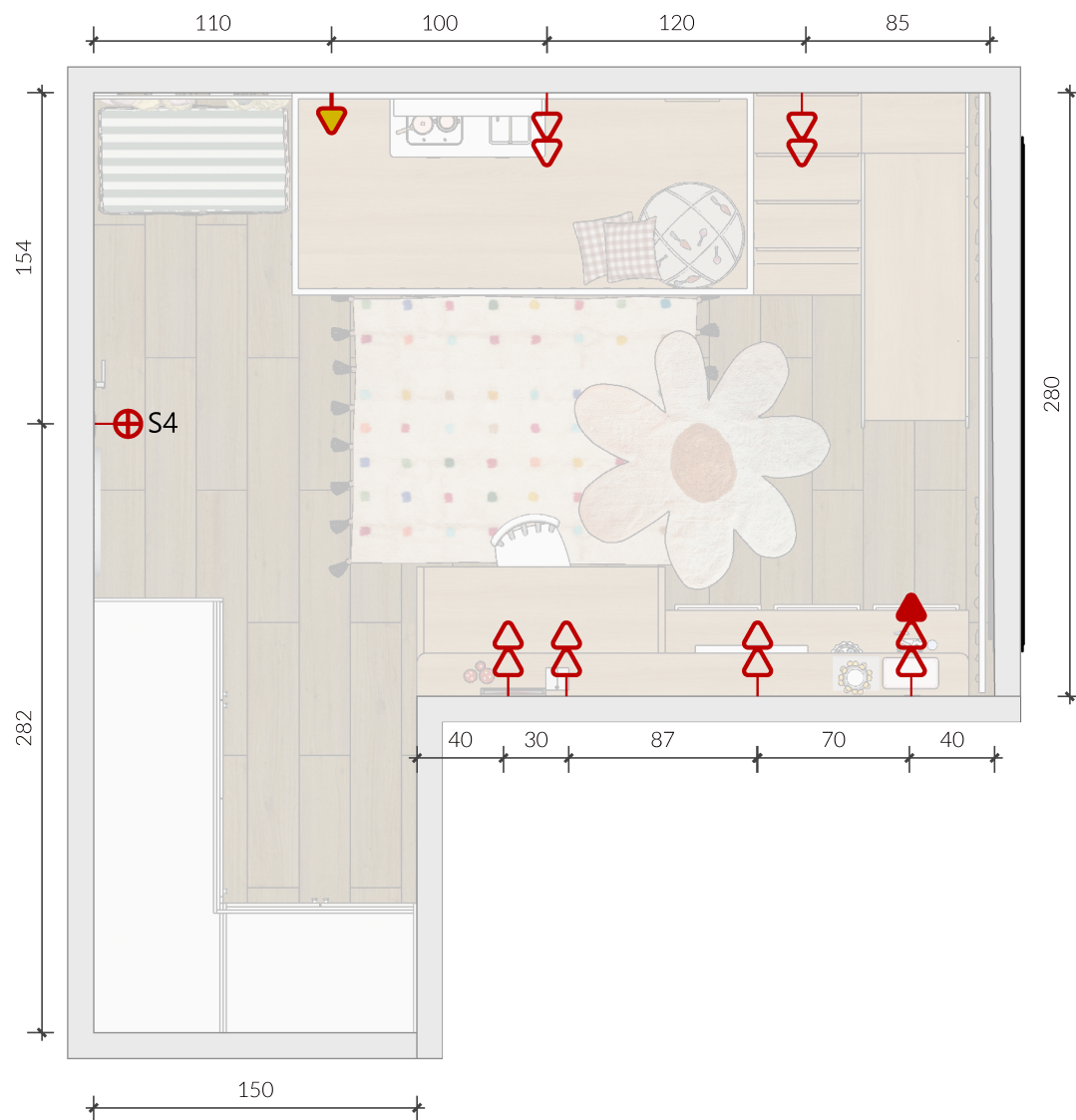
01 VISTA SUPERIOR PONTOS ELÉTRICOS Esc: 1/35
