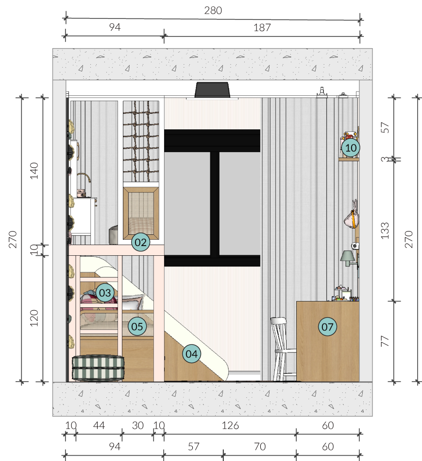
04 CORTE D - VISTA FRONTAL Esc: 1/35
