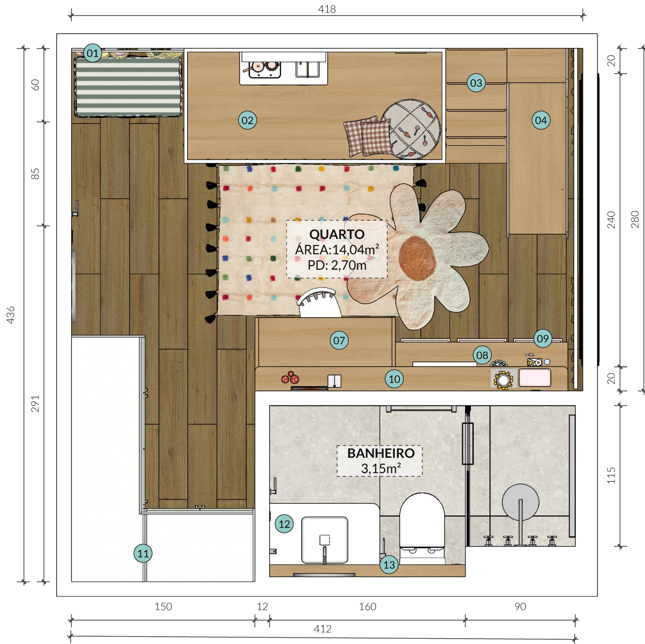
01 LAYOUT HUMANIZADO Esc: 1/30
