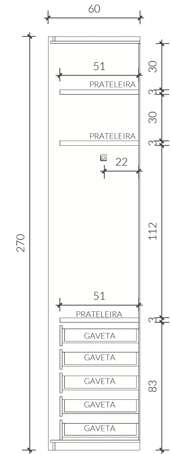
06 VISTA A PARTE 01 - GUARDA-ROUPAS Esc: 1/25
