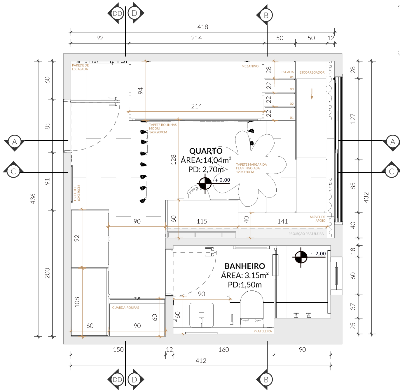
01 PLANTA TÉCNICA Esc: 1/35
