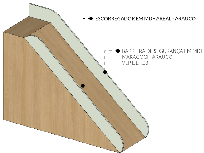
01 VISTA ISOMÉTRICA ESCADA Esc: 1/25
