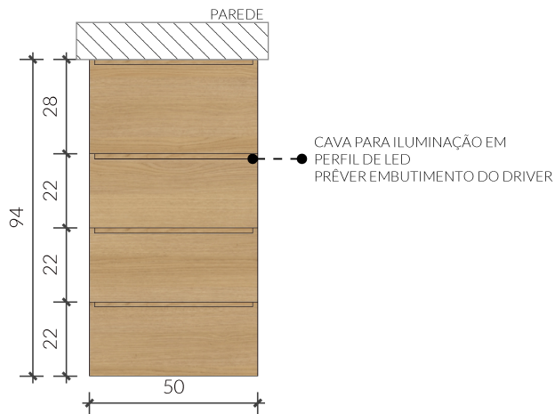
02 VISTA SUPERIOR ESCADA C/ GAVETAS Esc: 1/20
