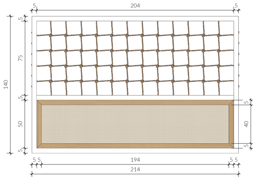
05 VISTA ISOLADA FRONTAL MEZANINO Esc: 1/20
