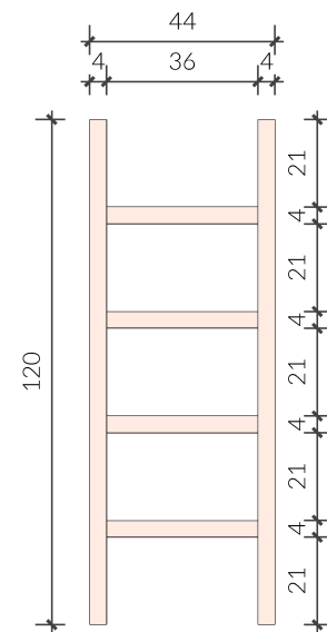
11 VISTA FRONTAL ESCADA MARINHEIRO Esc: 1/20
