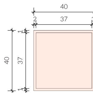
02 VISTA SUPERIOR BAÚ ORGANIZADOR Esc: 1/15
