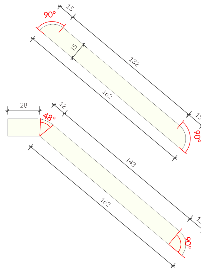
05 VISTA LATERAL GUARDA-CORPO Esc: 1/20
