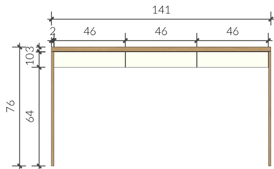
03 VISTA FRONTAL MÓVEL DE APOIO Esc: 1/25
