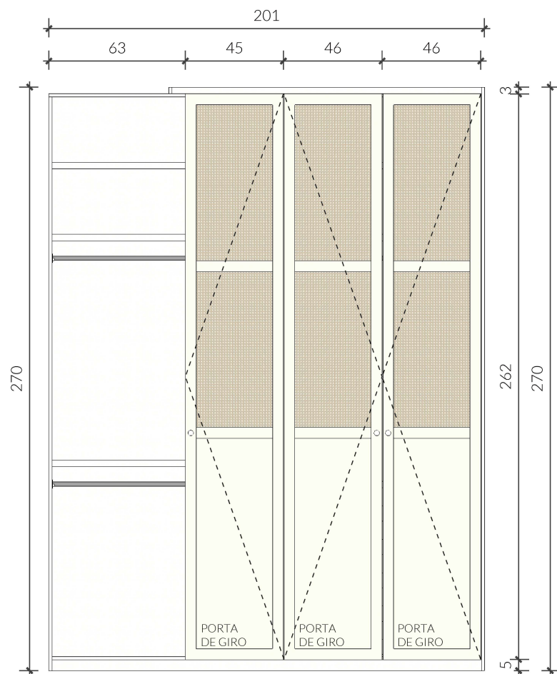
07 VISTA FRONTAL CORTE B PARTE 02 - GUARDA-ROUPAS Esc: 1/25
