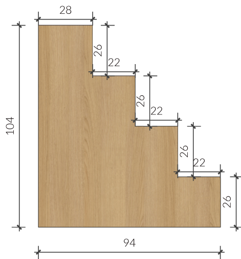
04 VISTA LATERAL ESCADA C/ GAVETAS Esc: 1/20
