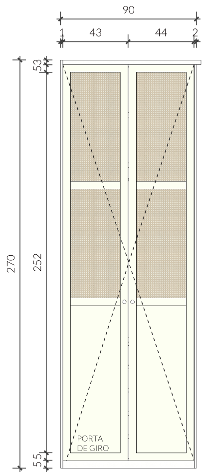
03 VISTA FRONTAL PARTE 01 - GUARDA-ROUPAS Esc: 1/25
