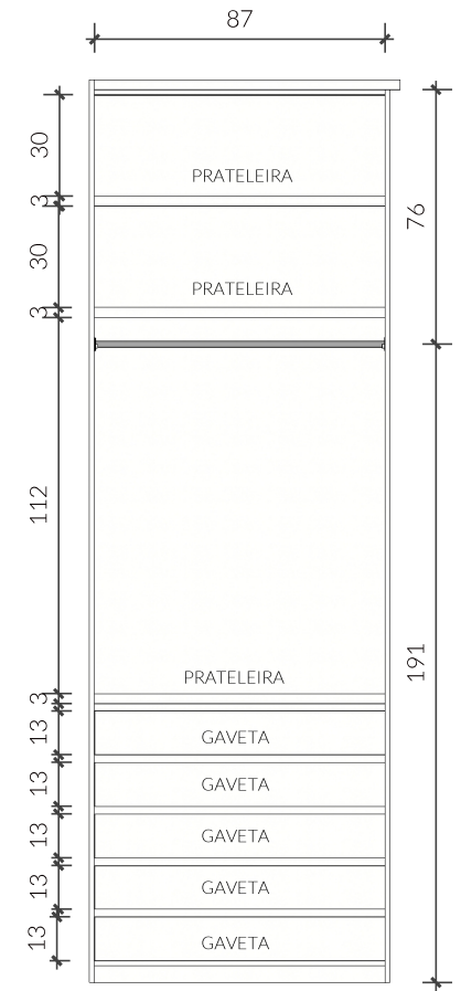
05 VISTA INTERNA PARTE 01 - GUARDA-ROUPAS Esc: 1/25
