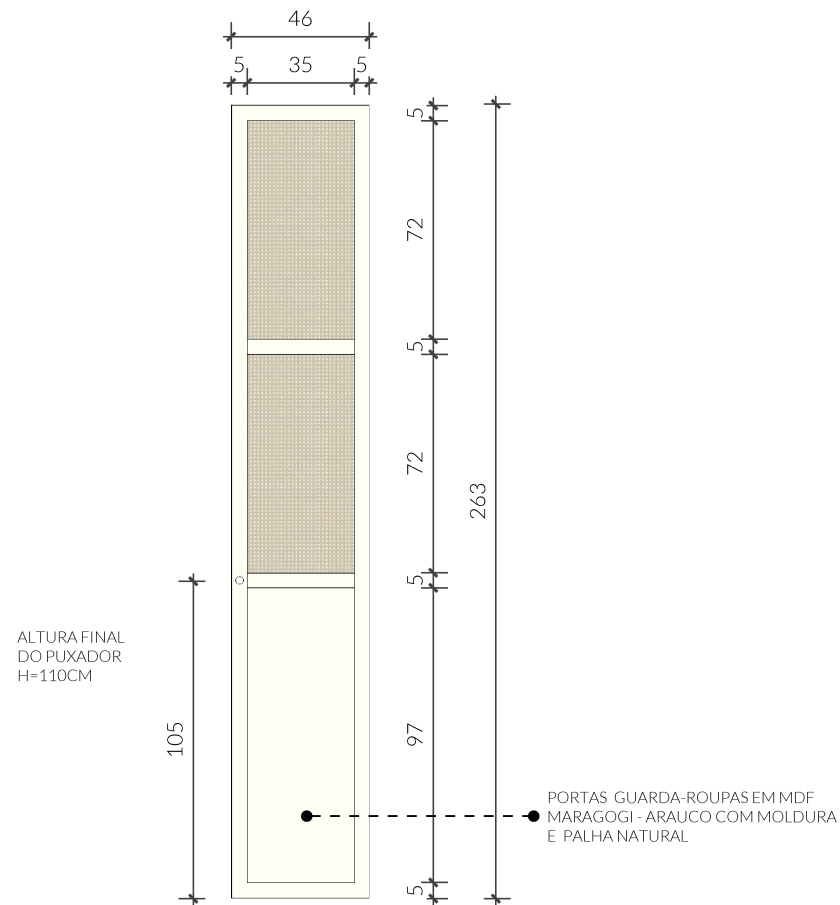
10 PORTAS DE GIRO PARTE 02 - GUARDA-ROUPAS Esc: 1/25
