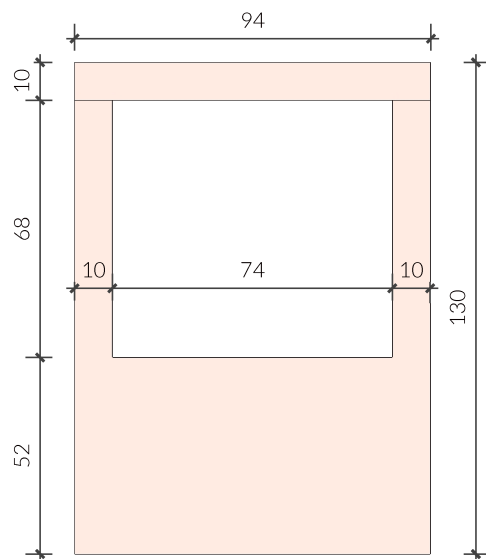
09 VISTA ISOLADA LATERAL MEZANINO Esc: 1/20
