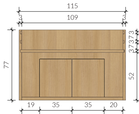
03 VISTA FRONTAL MESA EVOLUTIVA Esc: 1/25
