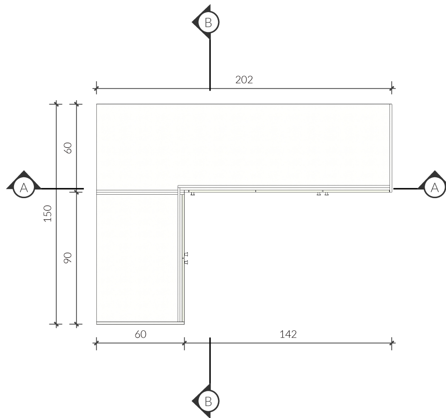
02 VISTA SUPERIOR GUARDA-ROUPAS Esc: 1/25
