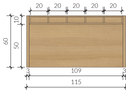
02 VISTA DUPERIOR MESA EVOLUTIVA Esc: 1/25
