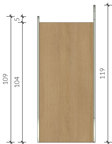
02 VISTA FRONTAL ESCORREGADOR Esc: 1/20
