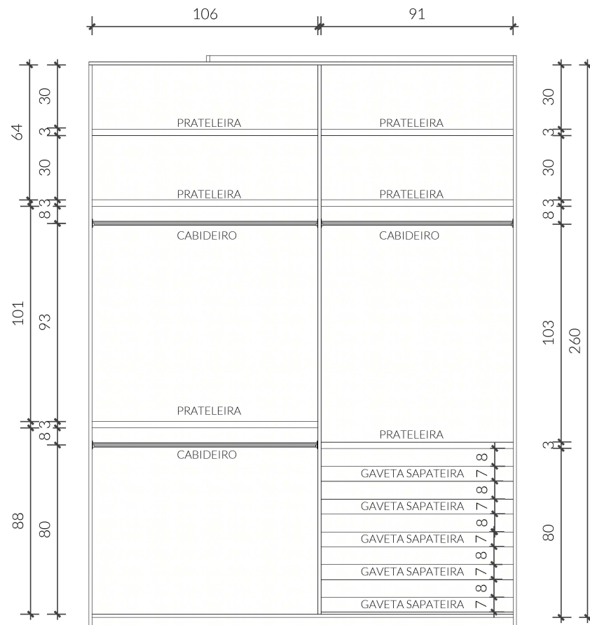
08 VISTA INTERNA CORTA B PARTE 02 - GUARDA-ROUPAS Esc: 1/25
