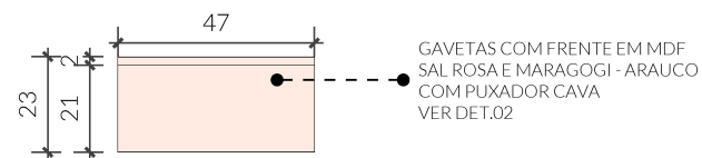
06 VISTA FRONTAL GAVETA Esc: 1/25
