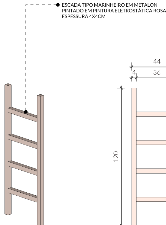
10 VISTA ISOMÉTRICA ESCADA MARINHEIRO Esc: 1/20
