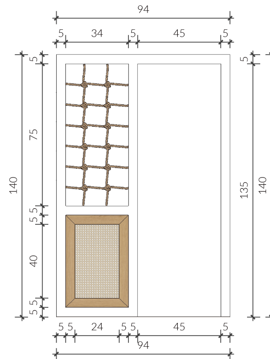
06 VISTA ISOLADA LATERAL MEZANINO Esc: 1/20
