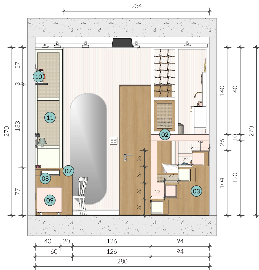
02 CORTE B - VISTA FRONTAL Esc: 1/35
