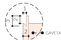
DET. 02 PUXADOR CAVA GAVETAS Esc: 1/05
