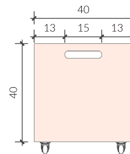
03 VISTA FRONTAL BAÚ ORGANIZADOR Esc: 1/15
