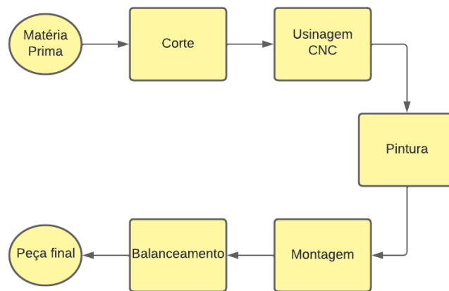
Figura 17 – Fluxograma da linha de produção por usinagem CNC
