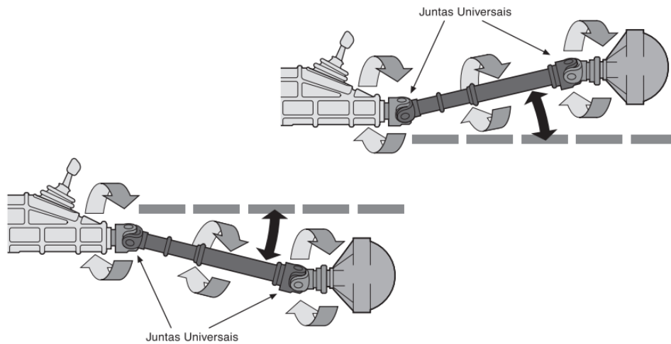
Figura 1 – Eixo de transmissão (Spicer, 2022)
