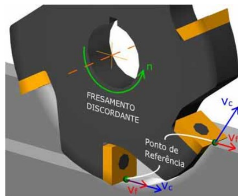
Figura 5 – Fresamento com parâmetros de sentido de rotação ( n ), velocidade de corte ( V_c ) e avanço ( V_f ) definidos. (CIMM, 2010)
