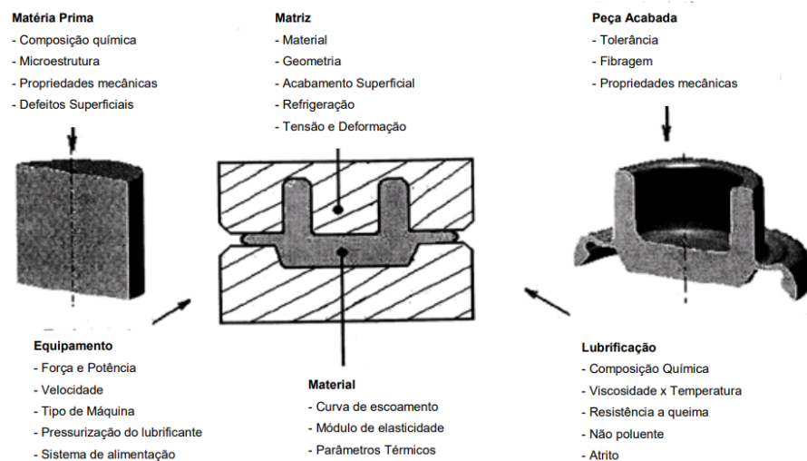
Figura 3 - Parâmetros fundamentais do forjamento (SCHAEFFER, 2006)
