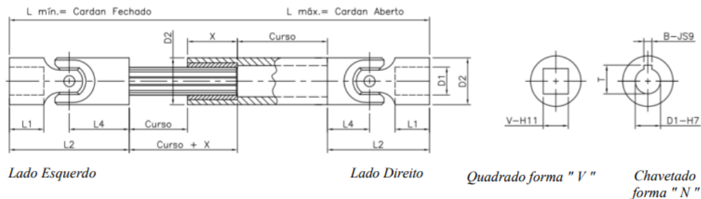
Figura 9 – Parâmetros do eixo (IMETEX, 2006).
