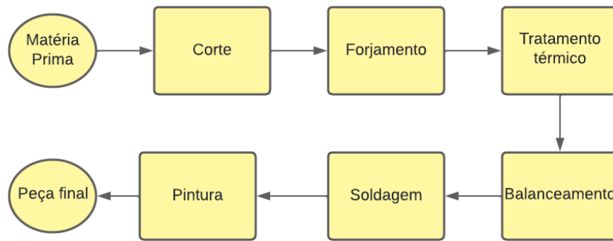
Figura 10 – Fluxograma da linha de produção por conformação mecânica.
