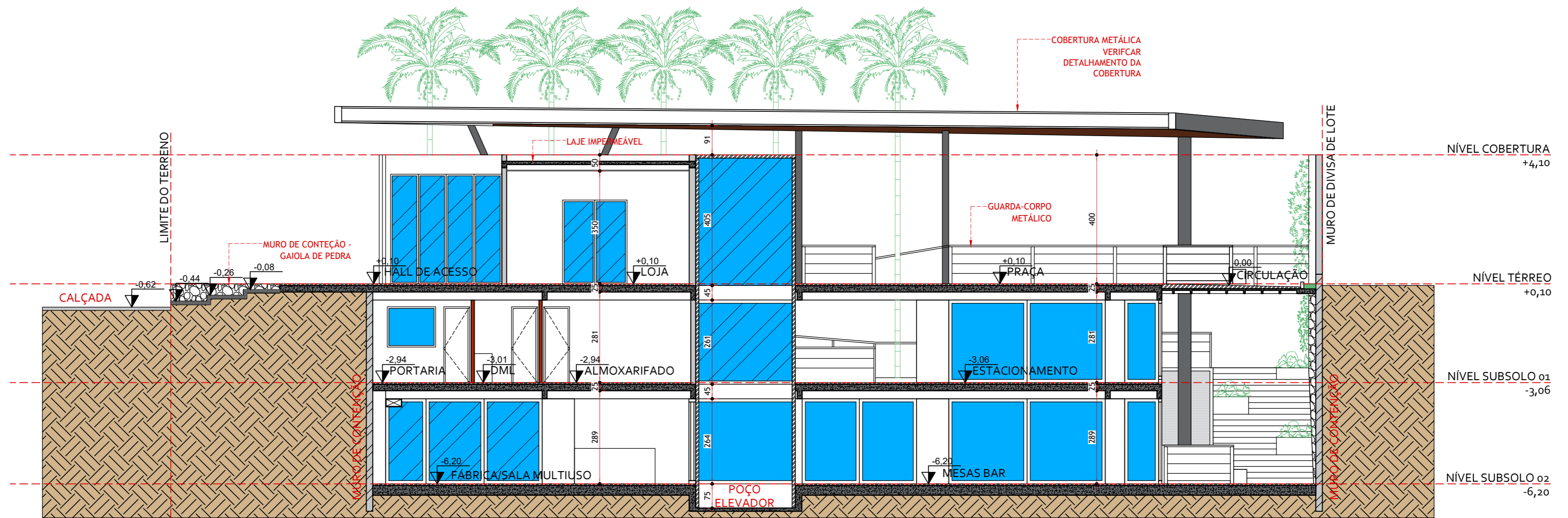
CORTE CC ESC 1:100
