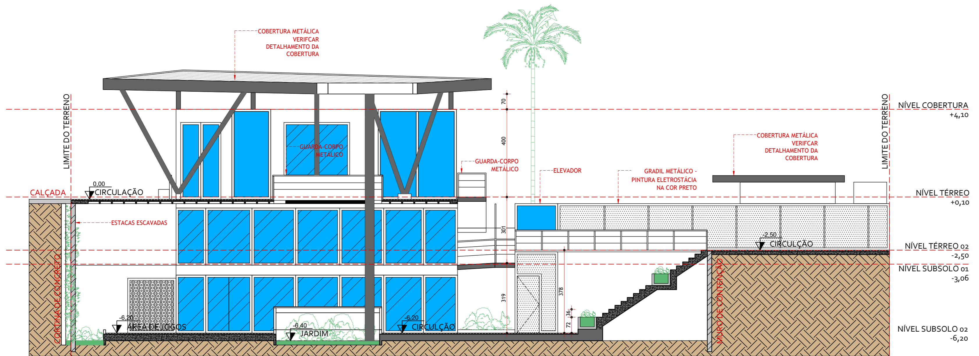
CORTE DD ESC 1:100
