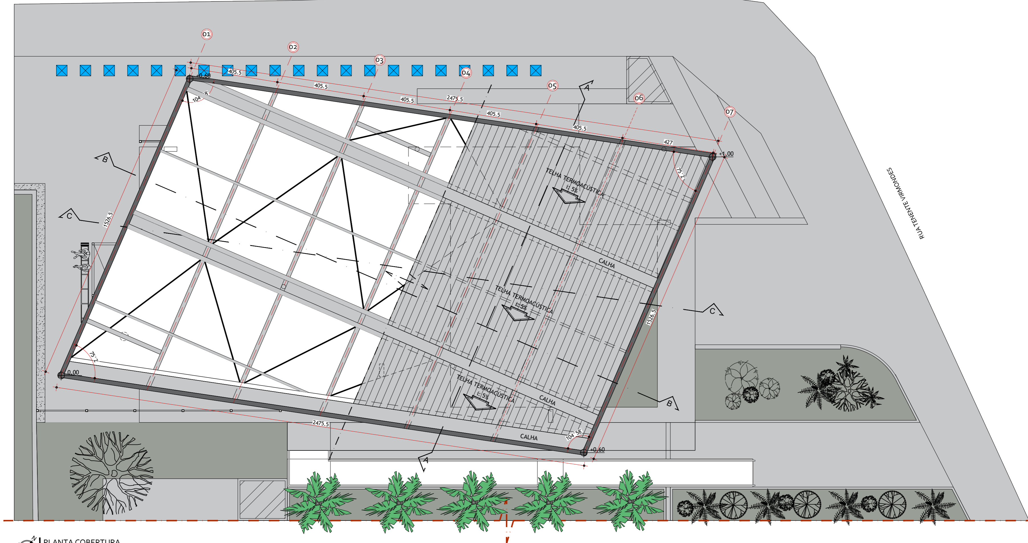
PLANTA COBERTURA ESC 1:100
