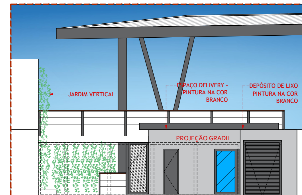
ELEVAÇÃO 03 ESC 1:100
