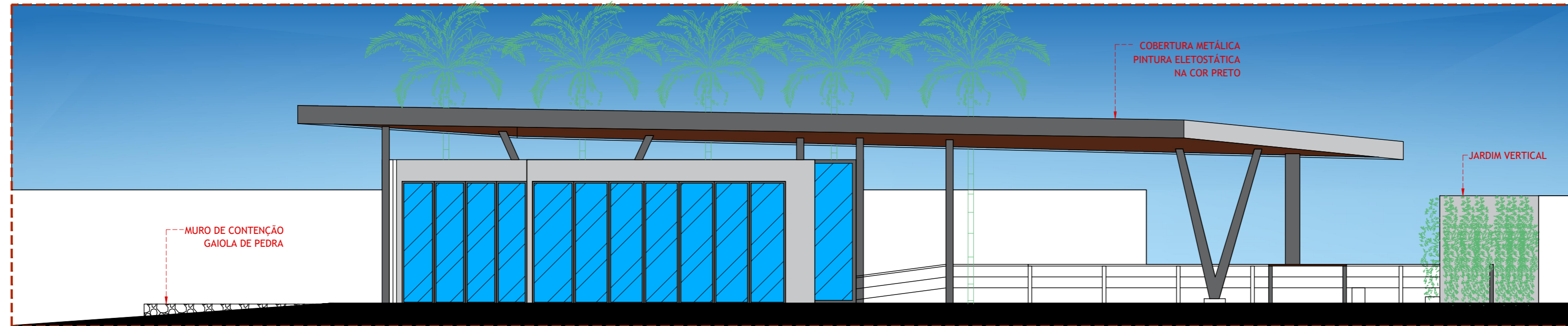
ELEVAÇÃO 01 ESC 1:100
