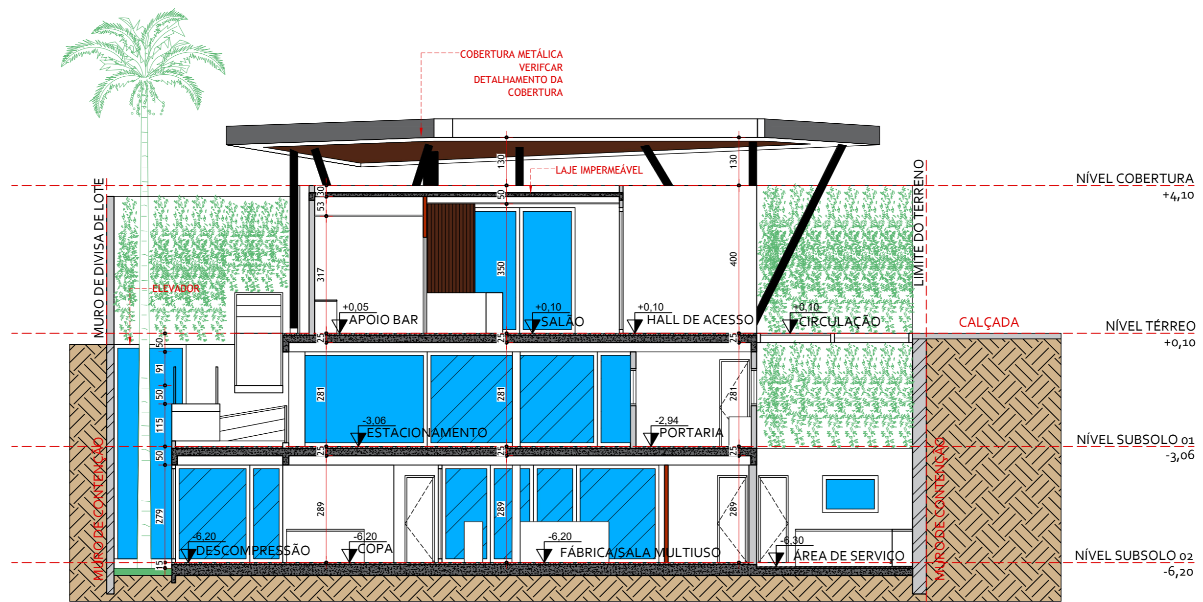
CORTE EE ESC 1:100
