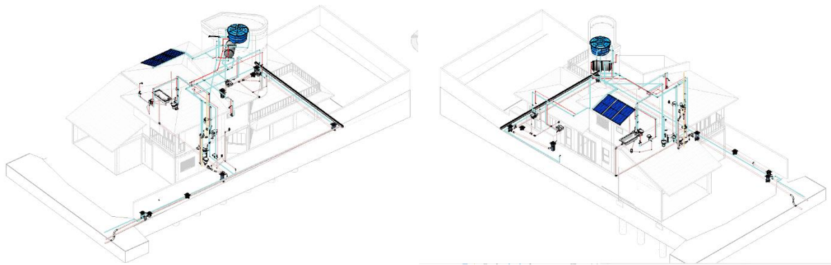
Figura 3 – Modelo hidrossanitário
