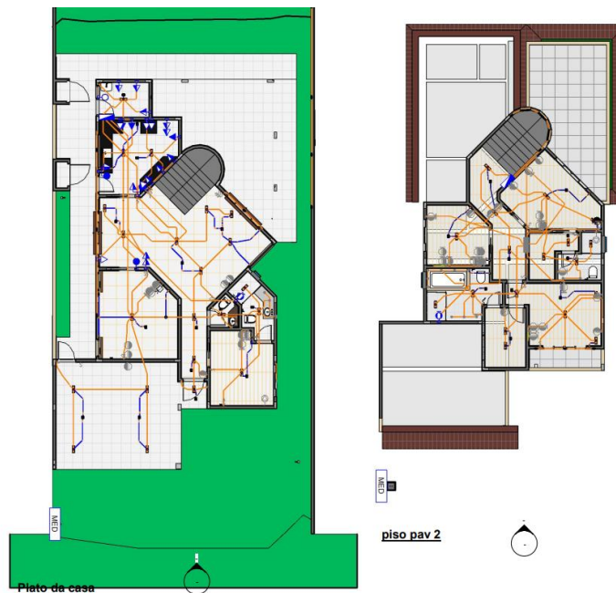
Figura 6 – Planta baixa com as tubulações elétricas.
