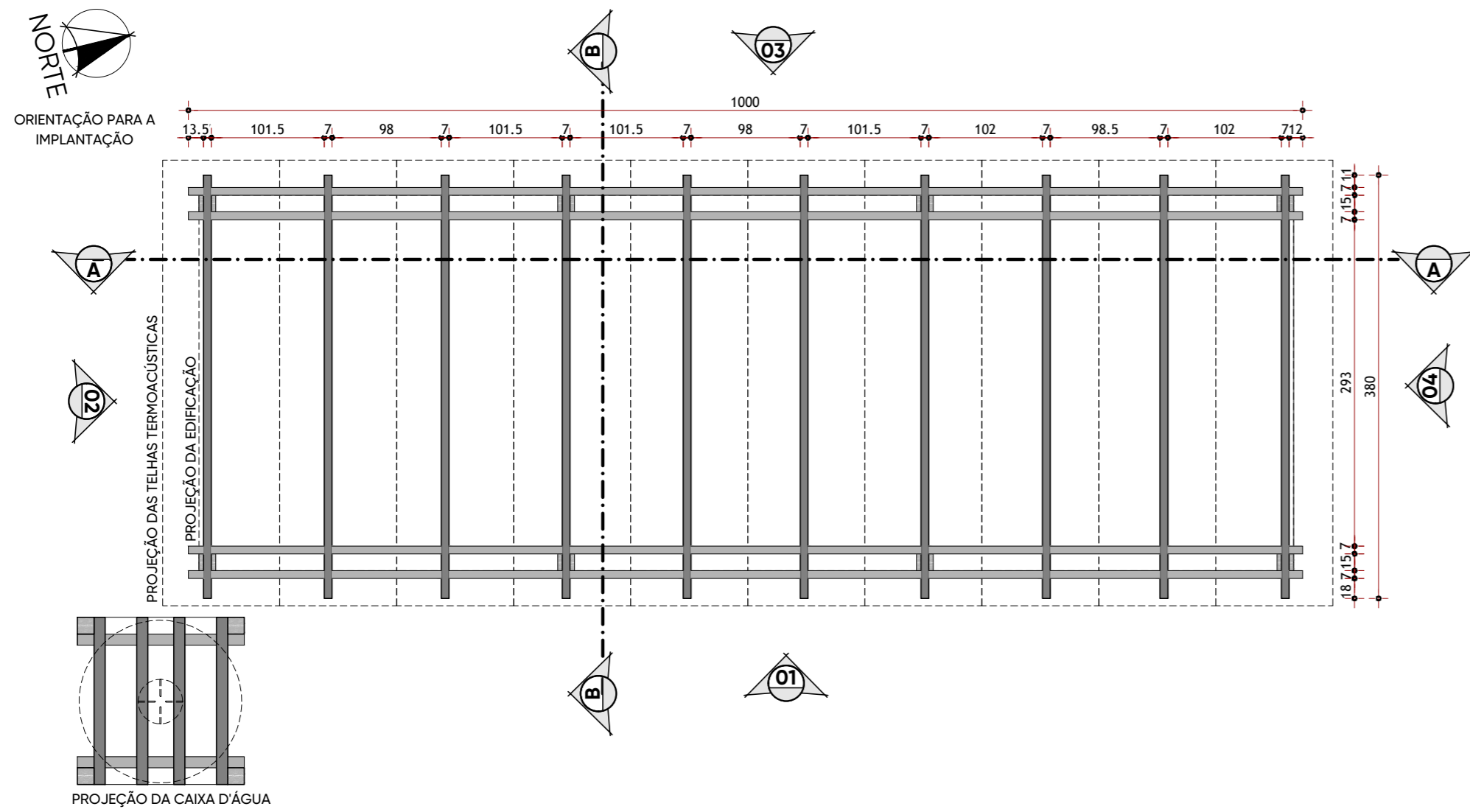
PLANTA DA ESTRUTURA DA COBERTURA - MÓDULO MAIOR (5 A 6 PESSOAS) ESC 1:50
