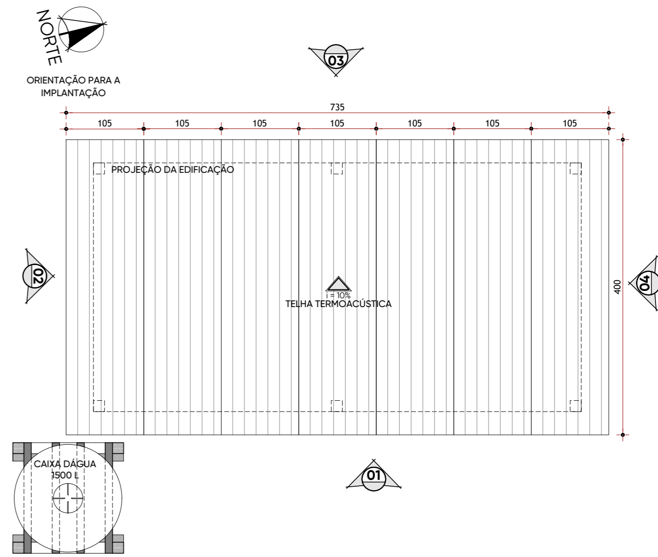
PLANTA DE COBERTURA - MÓDULO MENOR (2 PESSOAS) ESC 1:50
