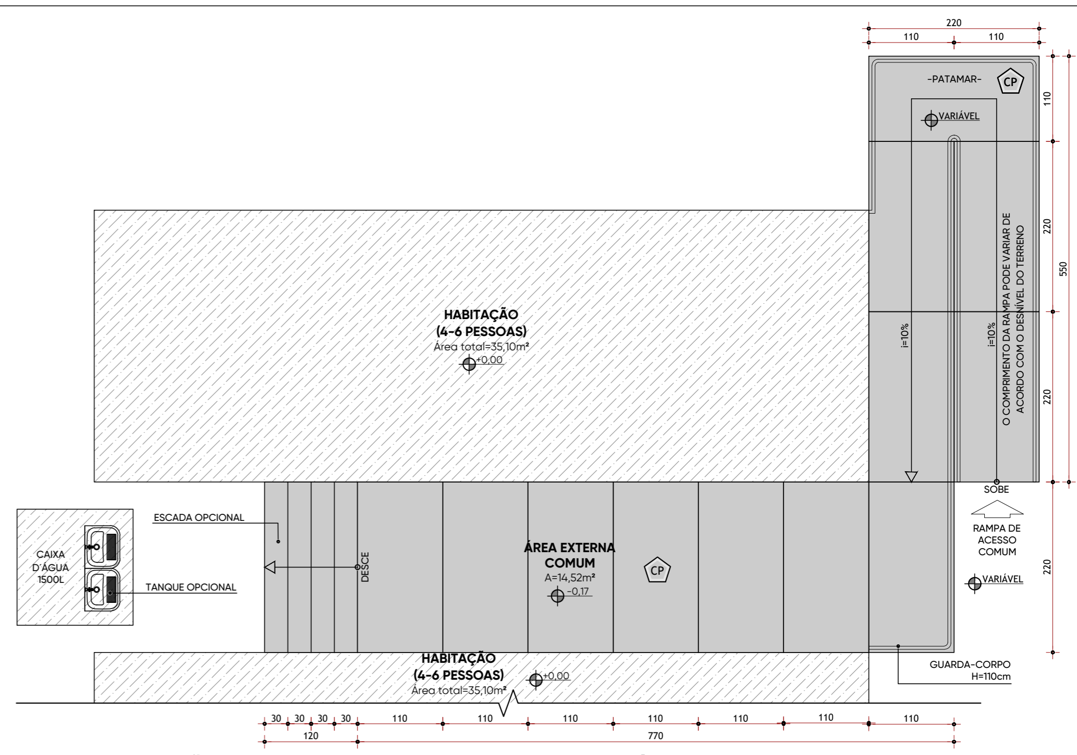
PAGINAÇÃO DE PISO DA ÁREA EXTERNA COMUM - MÓDULO MAIOR (5 A 6 PESSOAS)
