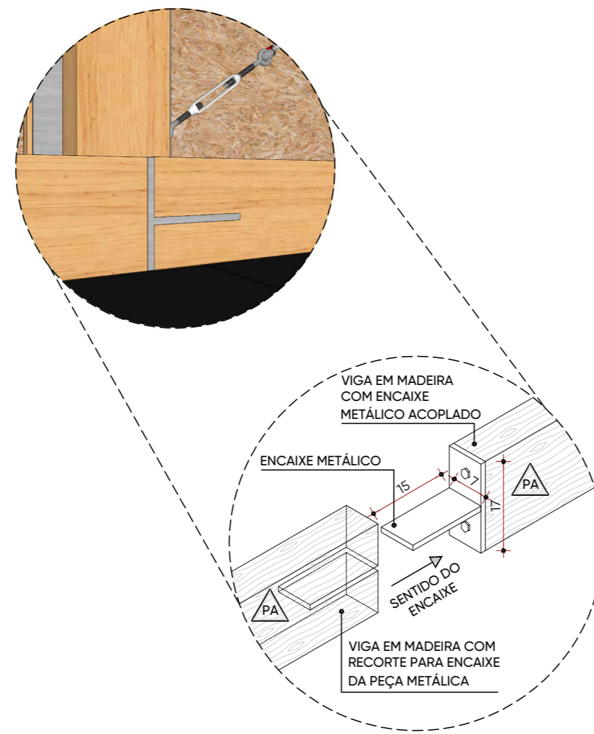
DET. 08 - ENCAIXE METÁLICO DAS VIGAS ESC 1:10
