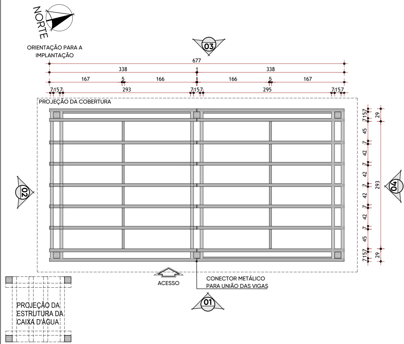
PLANTA ESTRUTURAL - MÓDULO MENOR (2 PESSOAS) ESC 1:50
