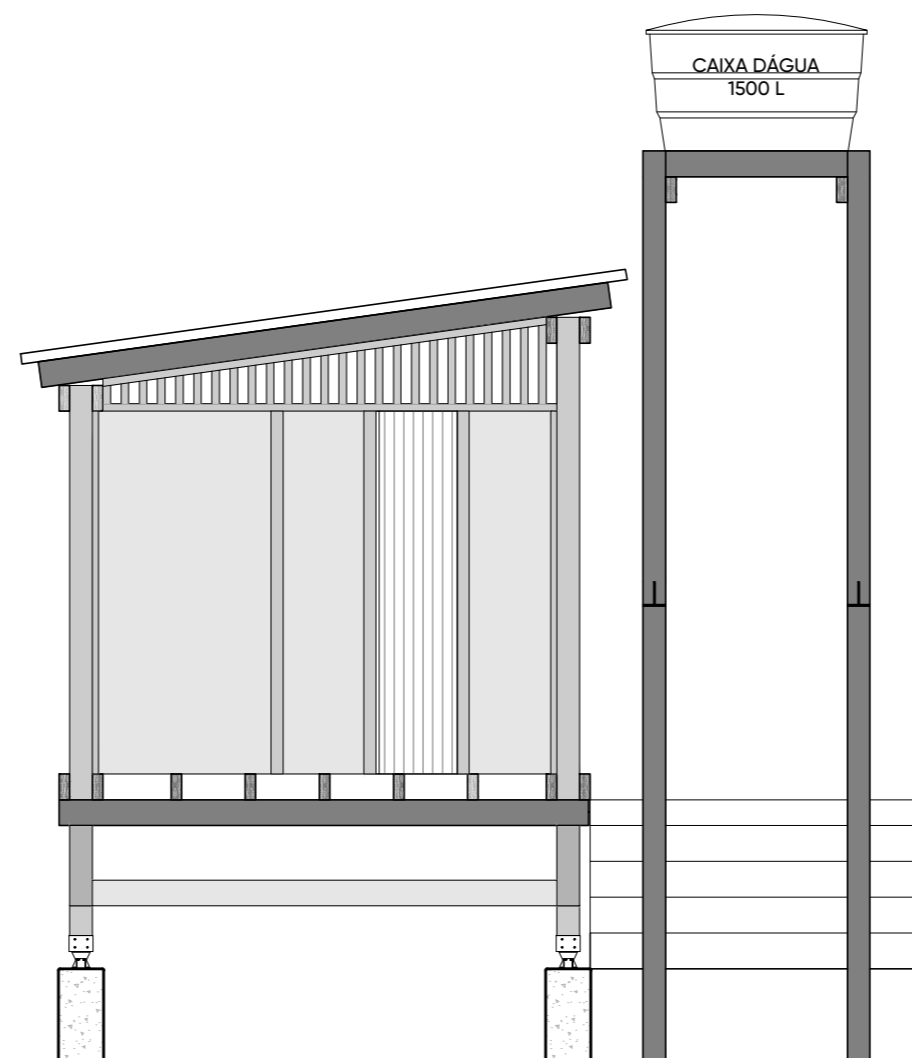
FACHADA 02 - MÓDULO MENOR (2 PESSOAS)
