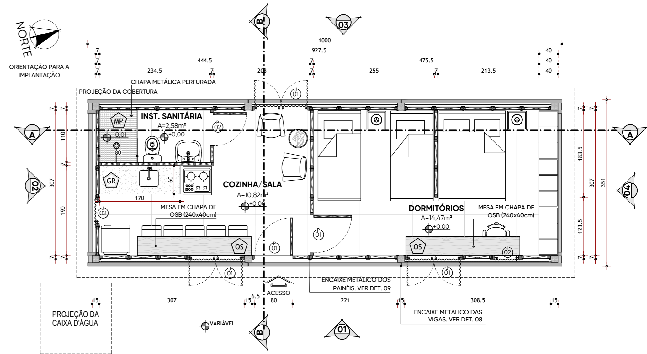
PLANTA COM SUGESTÃO DE LAYOUT - MÓDULO MAIOR (5 A 6 PESSOAS)
