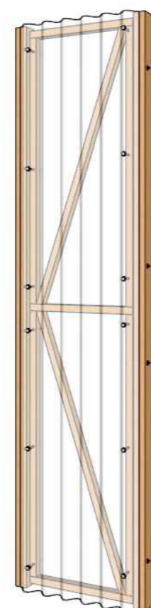
DET. 03 - PAINEL LUZ TELHA TRANSLÚCIDA ESC 1:20
