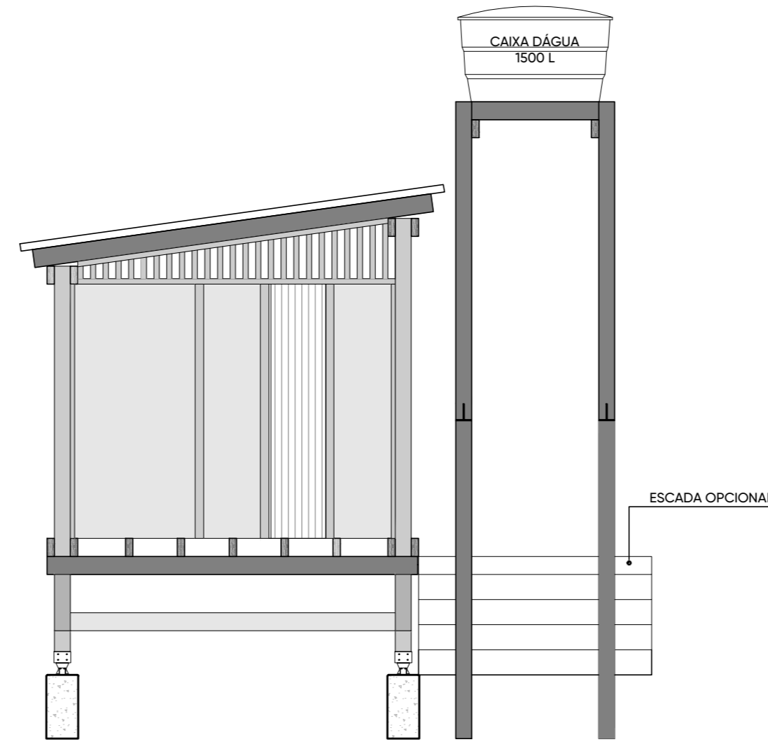
FACHADA 02 - MÓDULO MAIOR (4 A 6 PESSOAS) ESC 1:50
