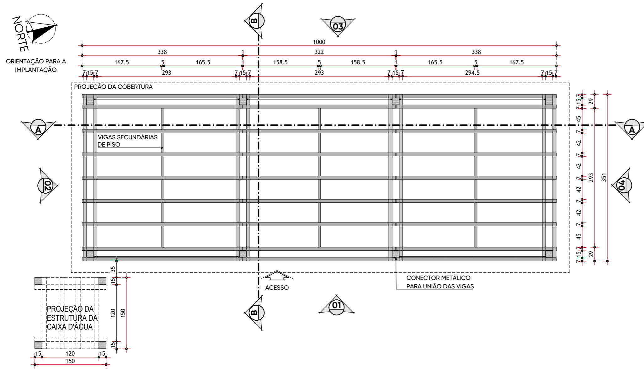
PLANTA ESTRUTURAL - MÓDULO MAIOR (5 A 6 PESSOAS) ESC 1:50
