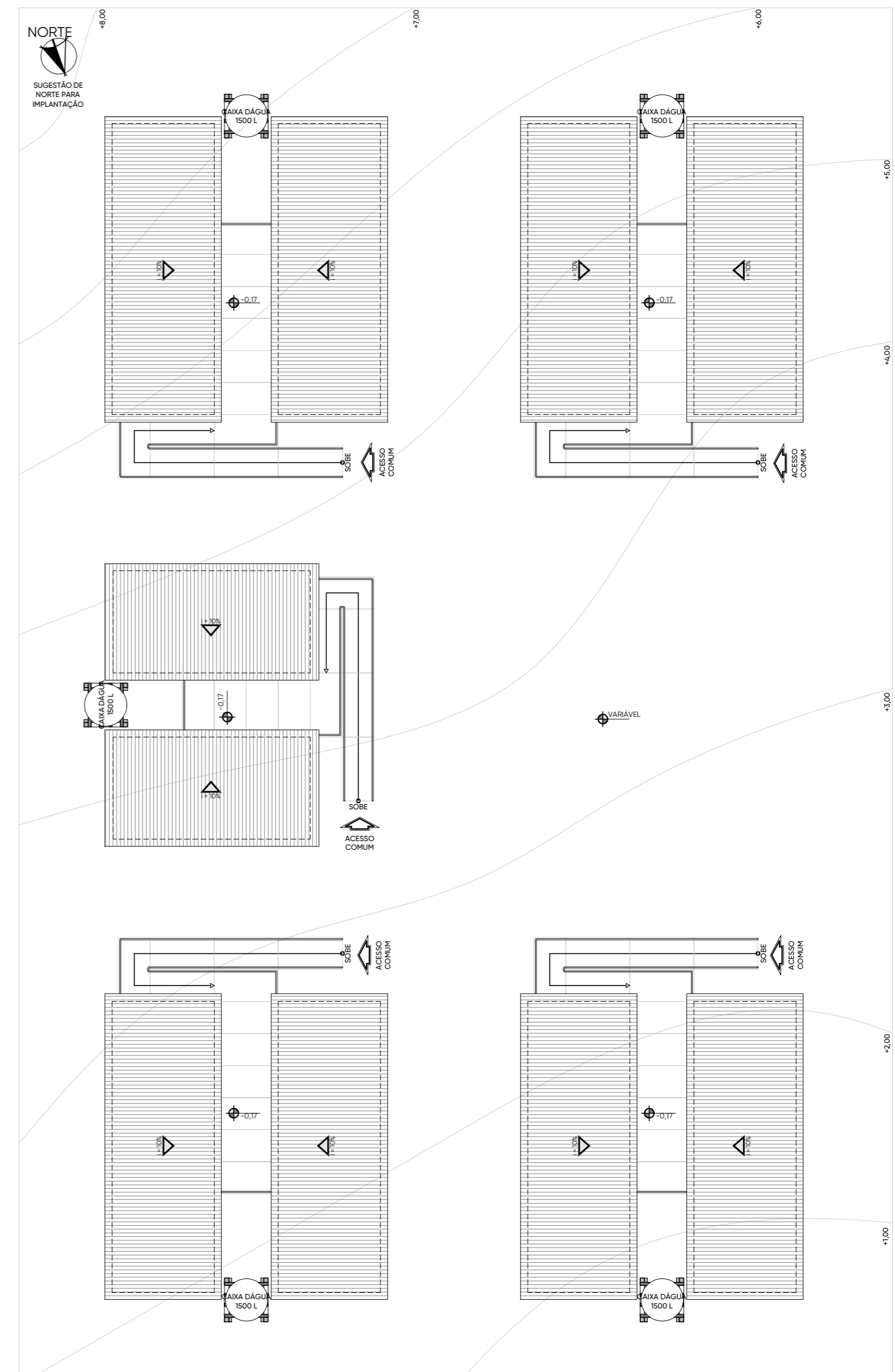
EXEMPLO DE IMPLANTAÇÃO 2 ESC 1:150
