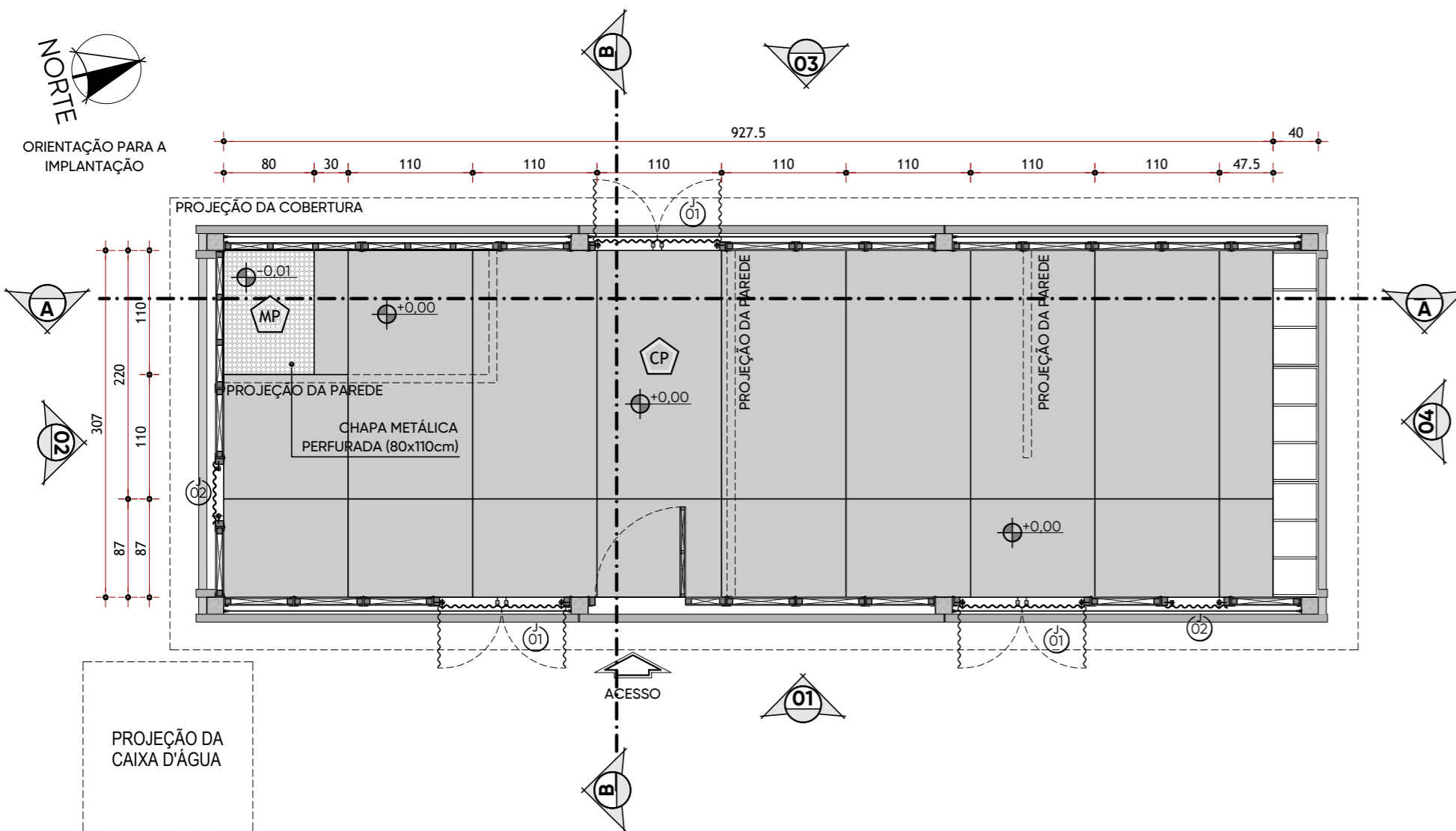
PAGINAÇÃO DE PISO - MÓDULO MAIOR (5 A 6 PESSOAS) ESC 1:50
