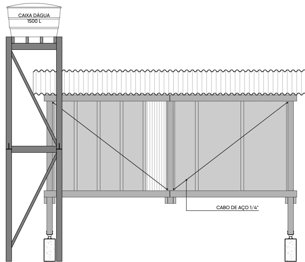
FACHADA 03 - MÓDULO MENOR (2 PESSOAS) ESC 1:50
