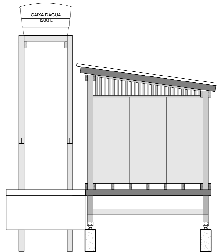
FACHADA 04 - MÓDULO MENOR (2 PESSOAS) ESC 1:50
