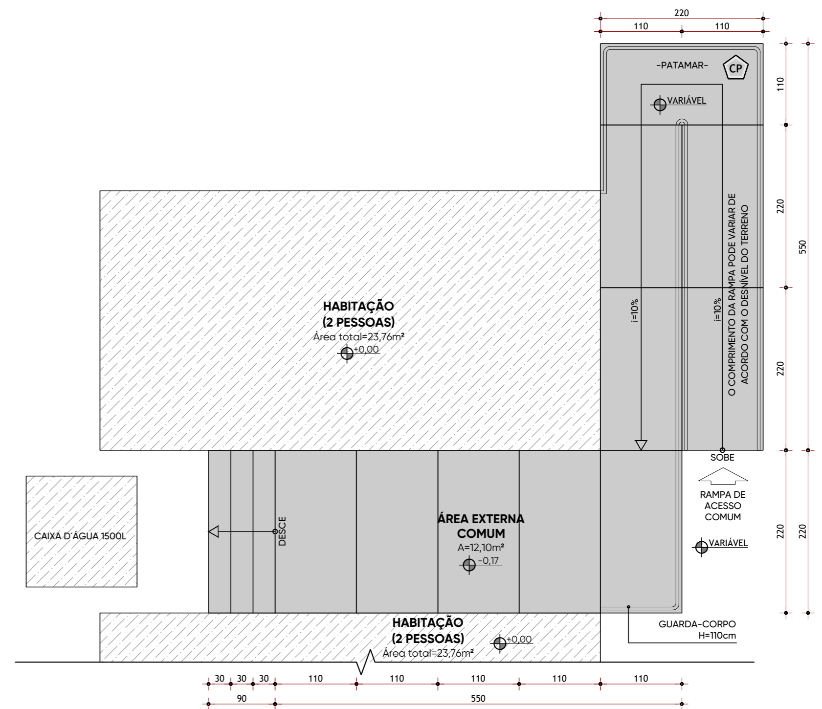
PAGINAÇÃO DE PISO DA ÁREA EXTERNA COMUM - MÓDULO MAIOR (2 PESSOAS)
