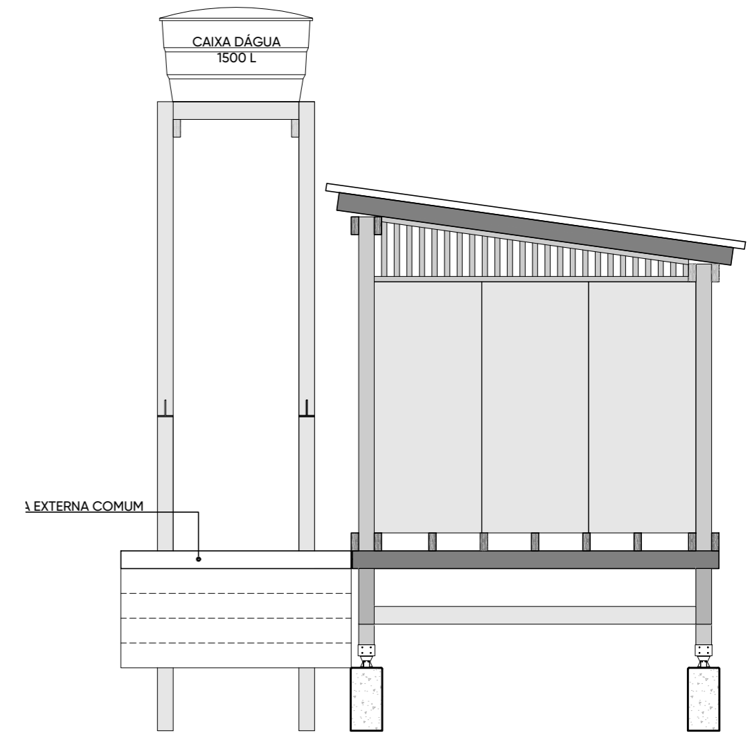
FACHADA 04 - MÓDULO MAIOR (4 A 6 PESSOAS) ESC 1:50
