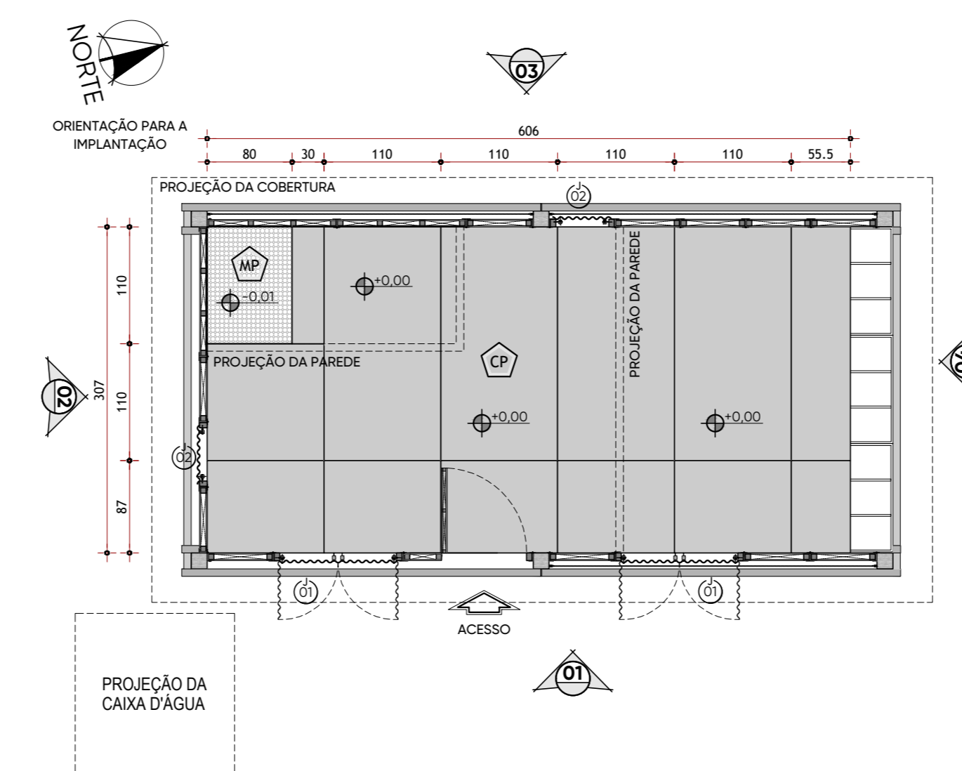
PAGINAÇÃO DE PISO - MÓDULO MENOR (2 PESSOAS) ESC 1:50
