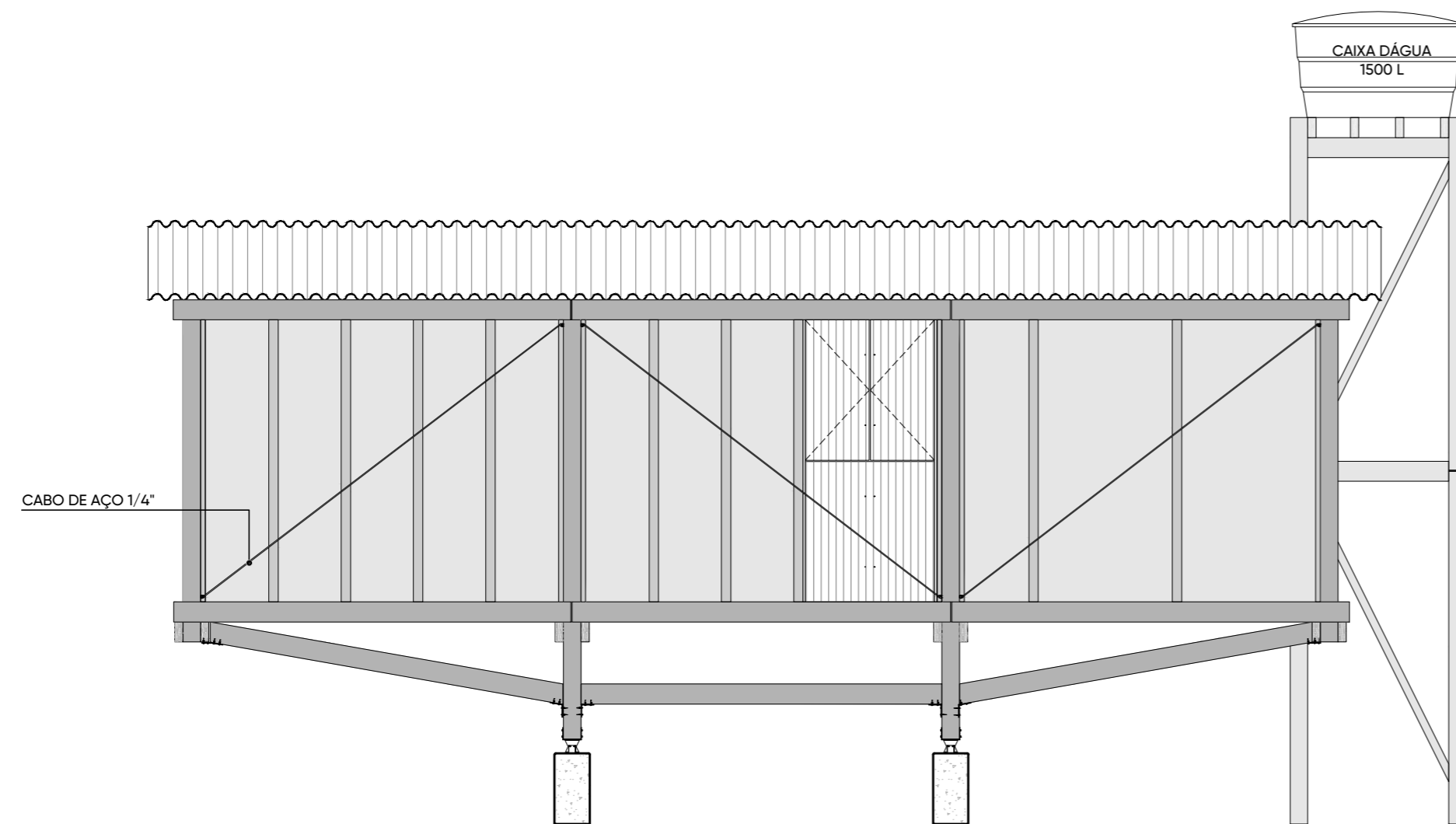
FACHADA 03 - MÓDULO MAIOR (4 A 6 PESSOAS) ESC 1:50
