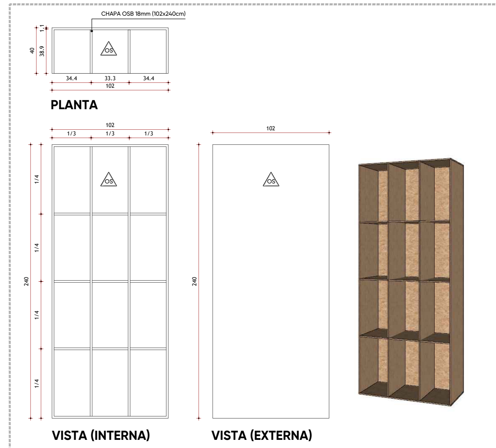
DET. 06 - PAINEL ESTRUTURAL NICHU ESC 1:20
