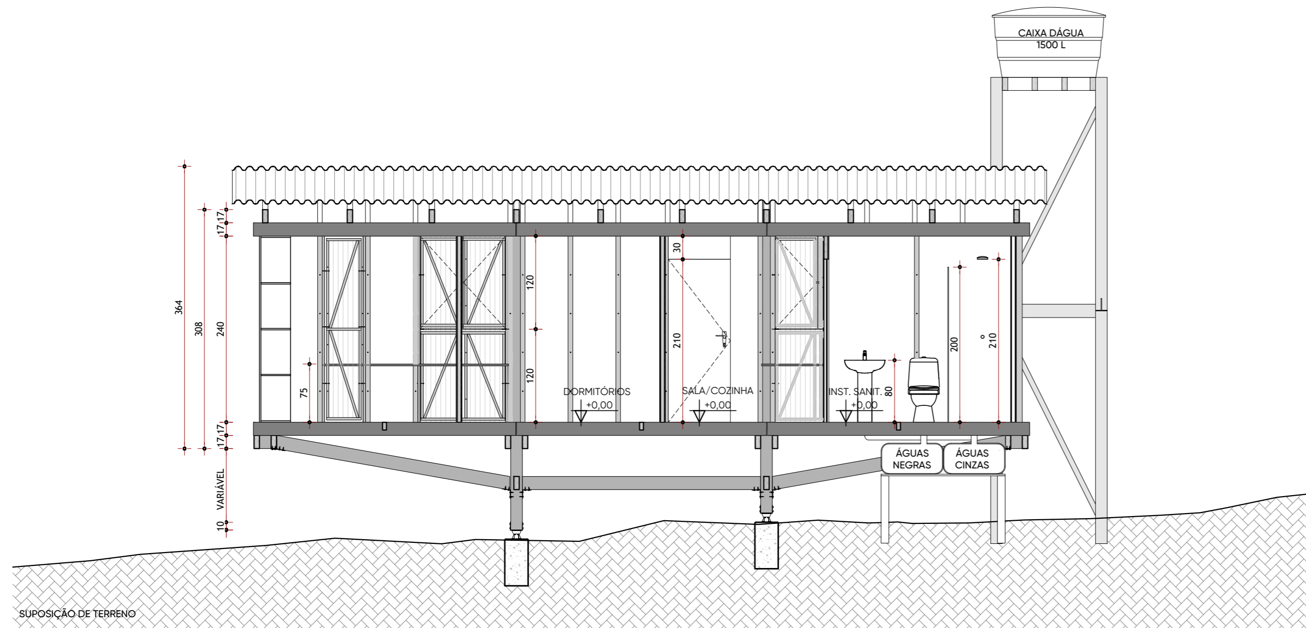
CORTE AA - MÓDULO MAIOR (4 A 6 PESSOAS) ESC 1:50
