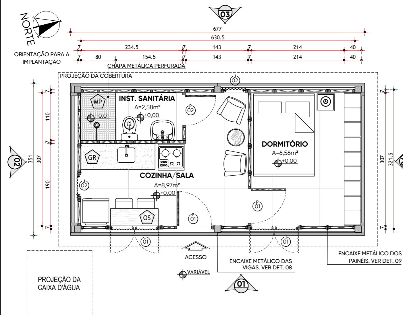
PLANTA COM SUGESTÃO DE LAYOUT - MÓDULO MENOR (2 PESSOAS) ESC 1:50 ÁREA INTERNA: 18,60 m²
