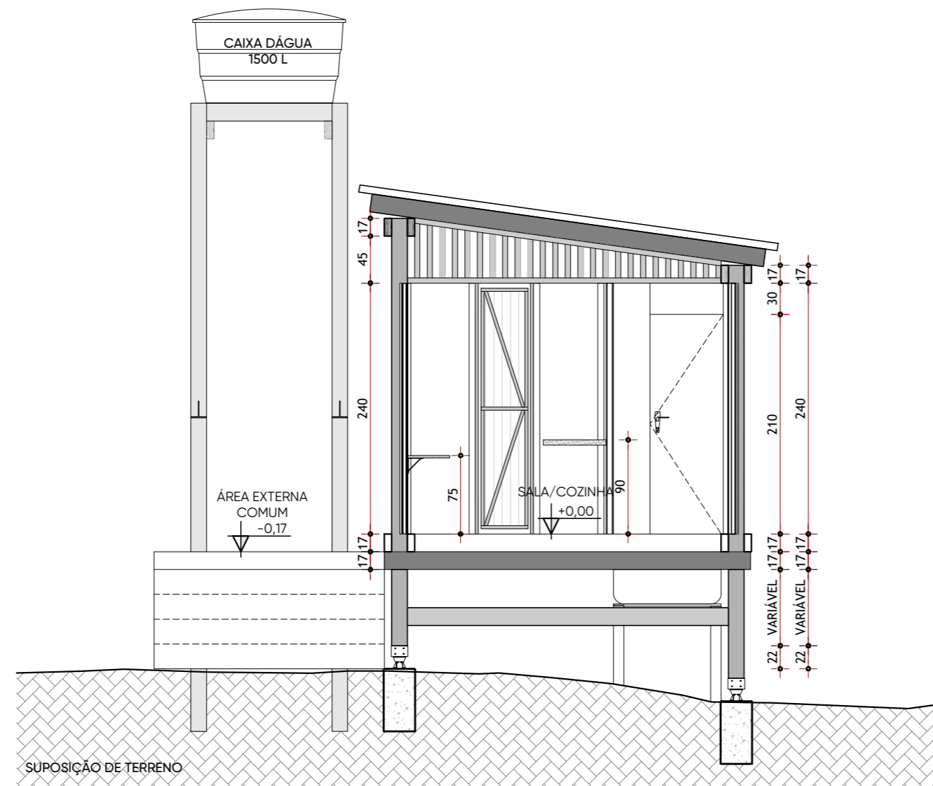
CORTE BB - MÓDULO MAIOR (4 A 6 PESSOAS)
