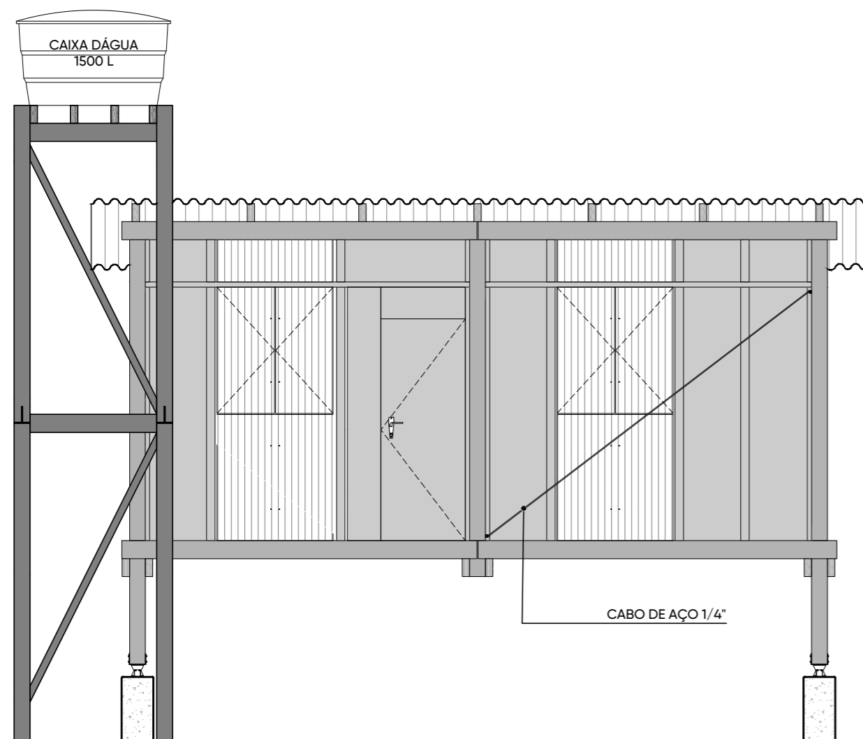
FACHADA 01 - MÓDULO MENOR (2 PESSOAS)
