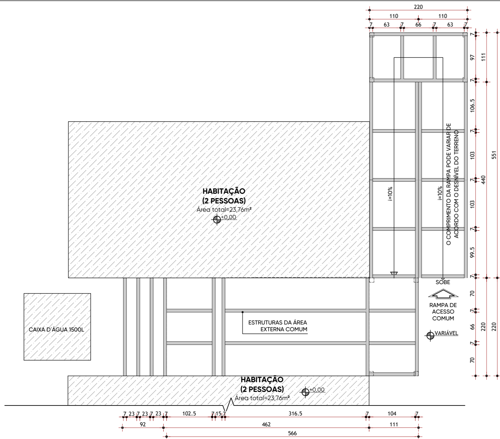
PLANTA ESTRUTURAL DA ÁREA EXTERNA COMUM - MÓDULO MAIOR (2 PESSOAS)
