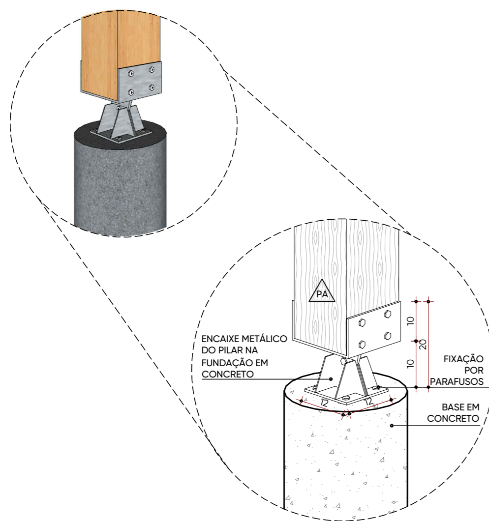
DET. 07 - JUNÇÃO DO PILAR NA FUNDAÇÃO ESC 1:10
