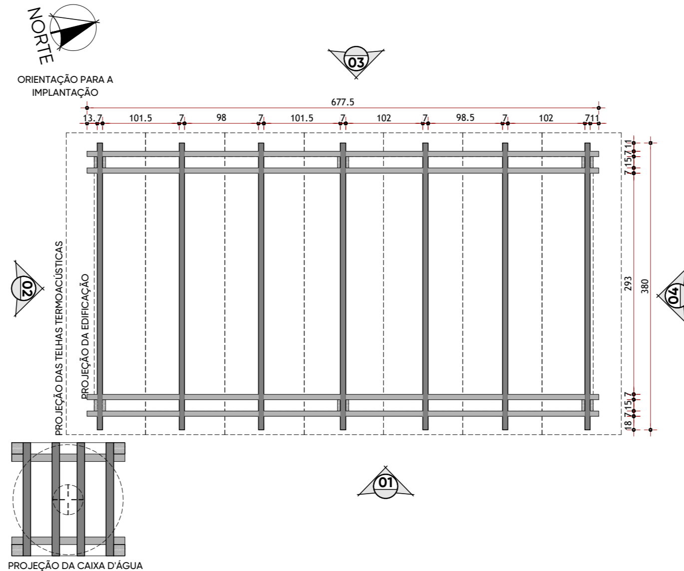
PLANTA DA ESTRUTURA DA COBERTURA - MÓDULO MENOR (2 PESSOAS) ESC 1:50
