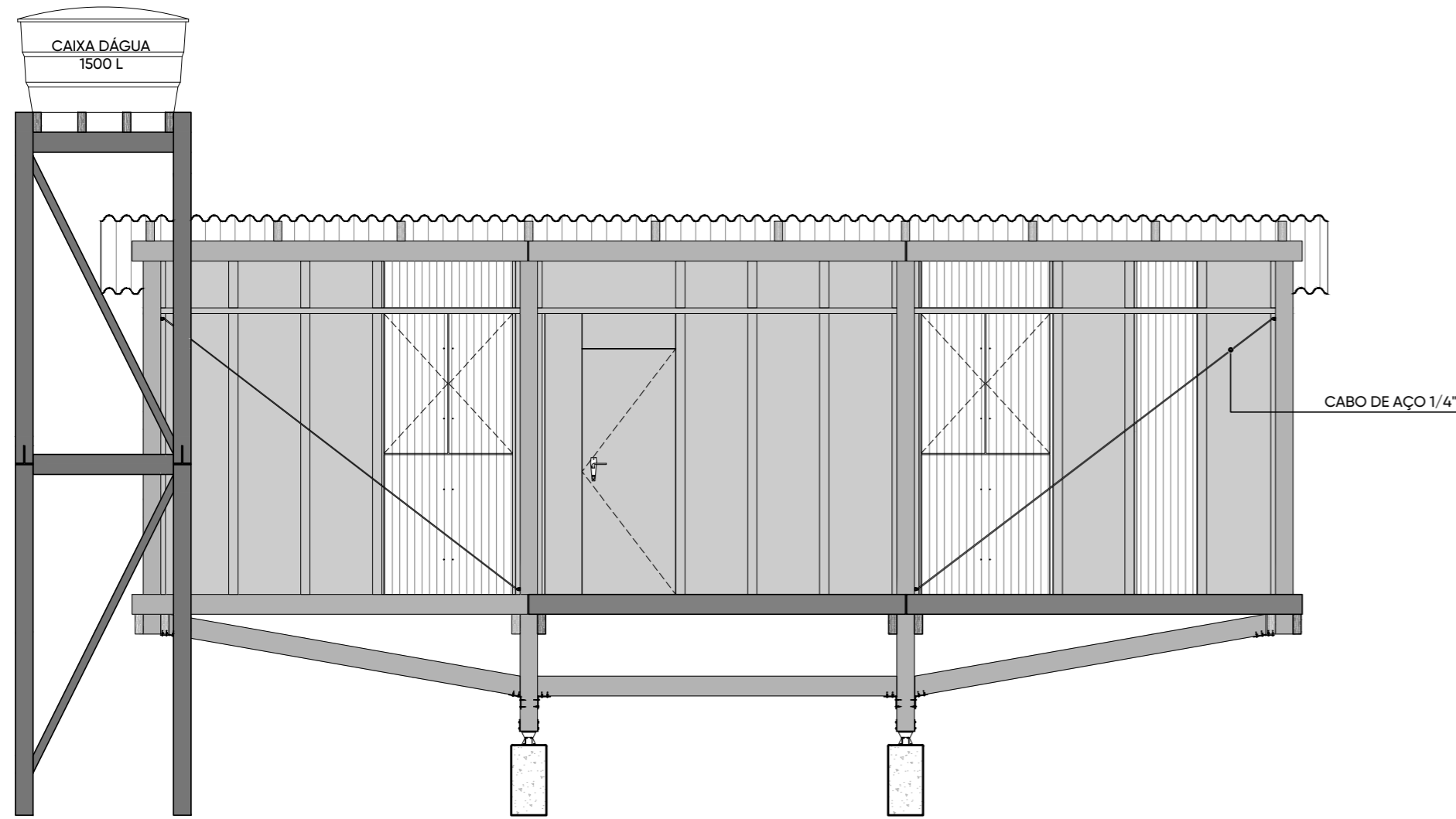
FACHADA 01 - MÓDULO MAIOR (4 A 6 PESSOAS) ESC 1:50
