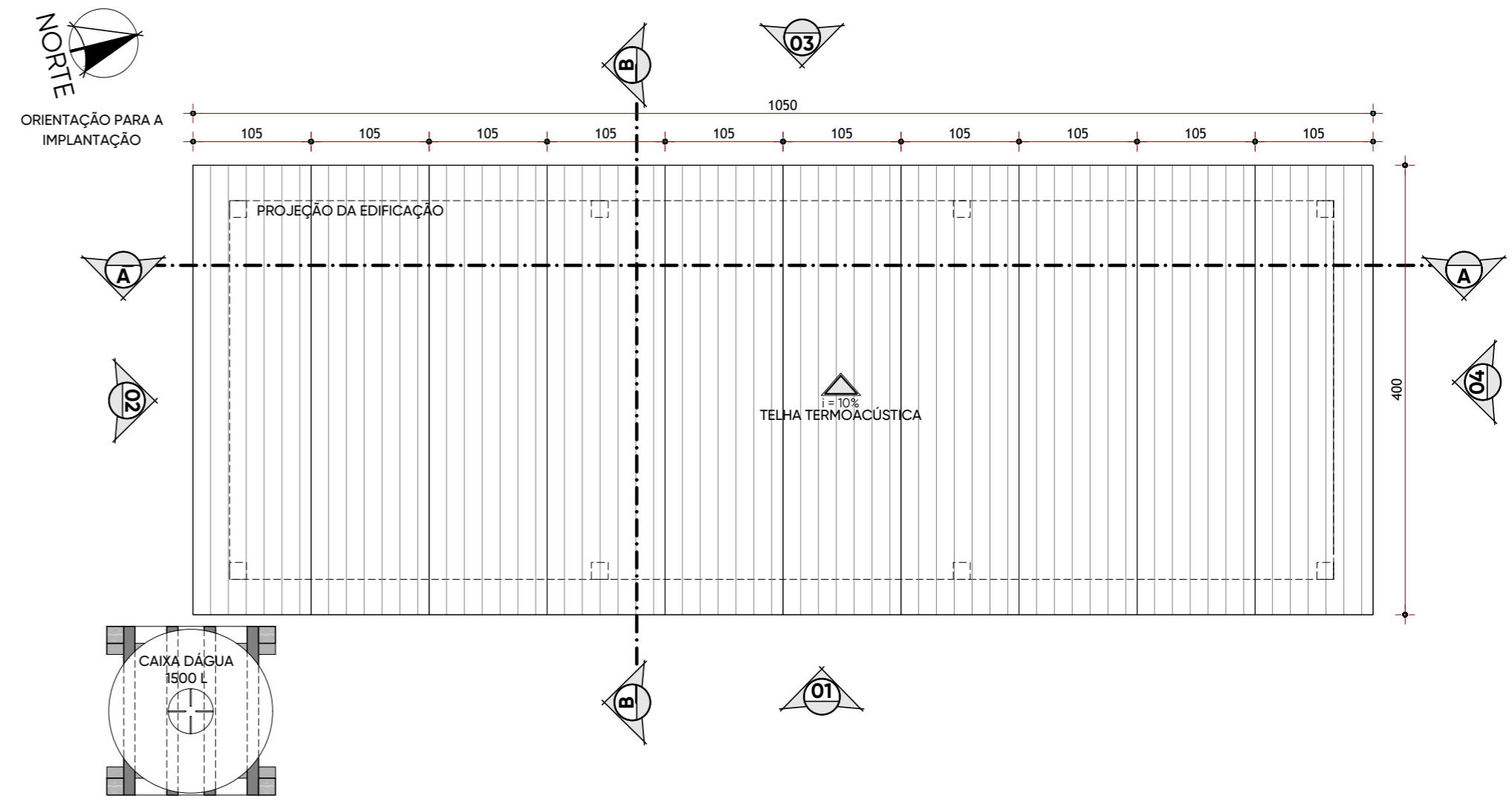
PLANTA DE COBERTURA - MÓDULO MAIOR (5 A 6 PESSOAS) ESC 1:50
