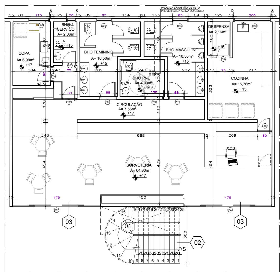
PLANTA LAYOUT TIPO (SORVETERIA) ESC. 1:100
