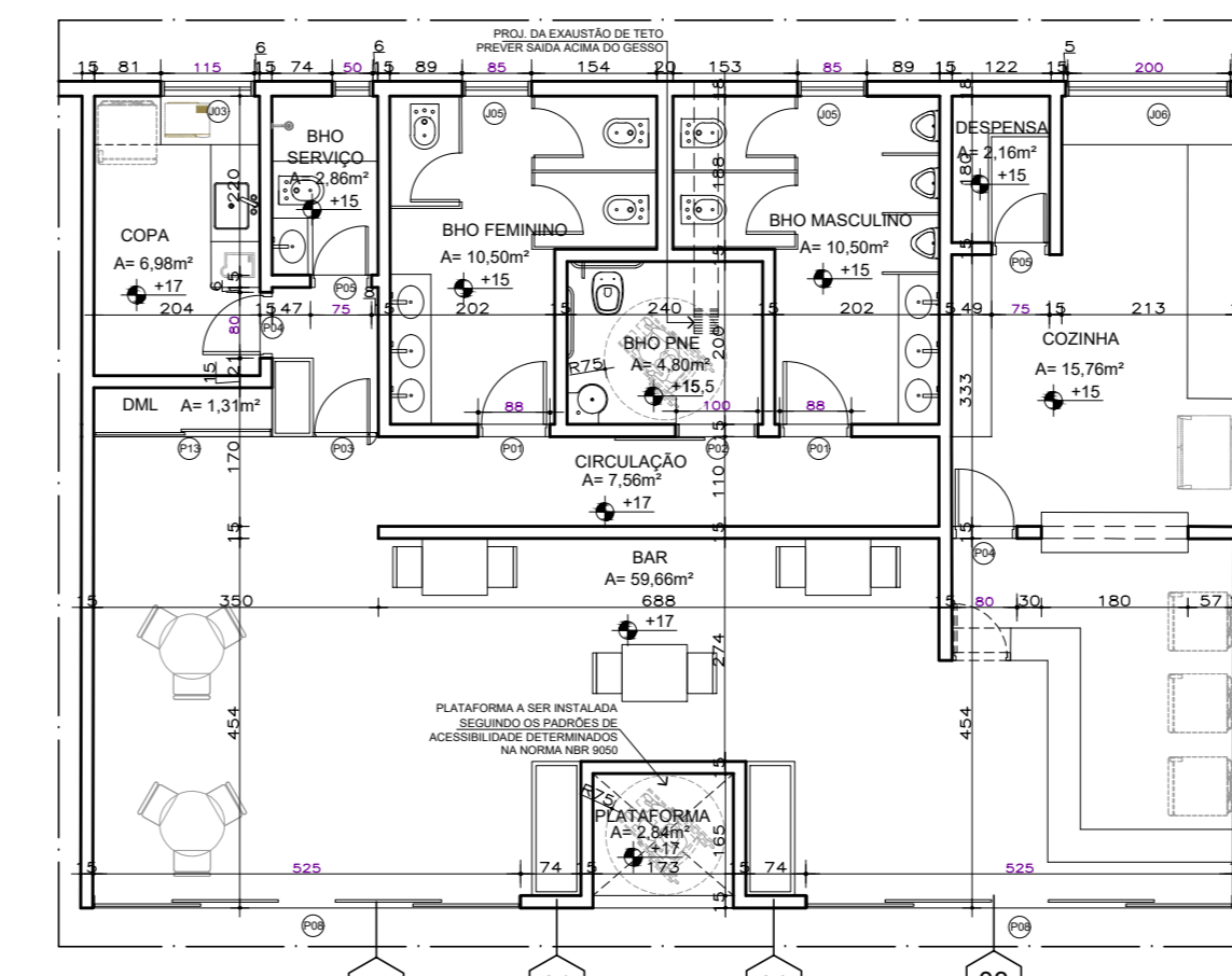
PLANTA LAYOUT TIPO (BAR) ESC. 1:100
