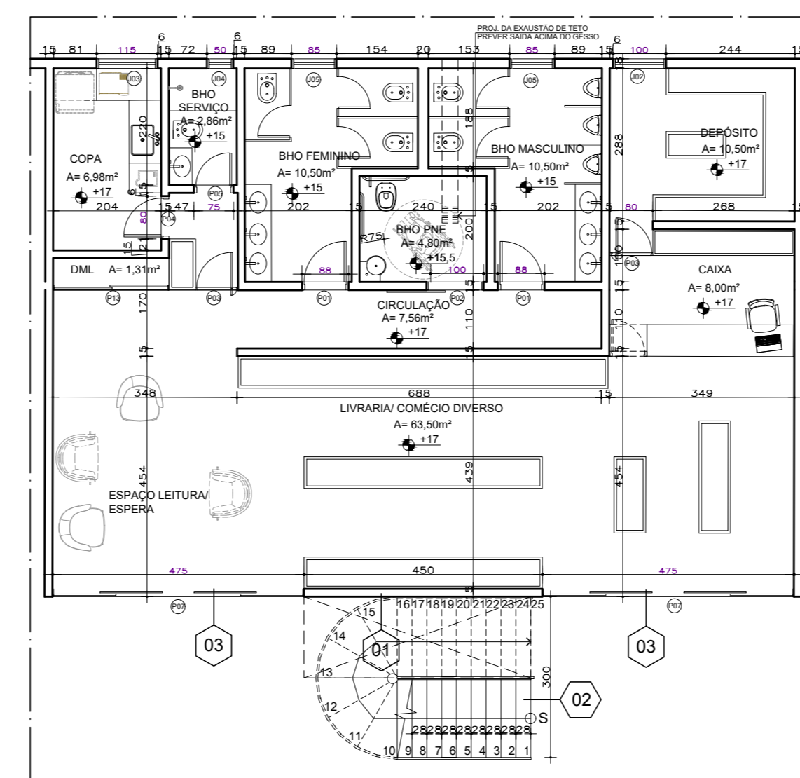
PLANTA LAYOUT TIPO (COMÉRCIO DIVERSO) ESC. 1:100
