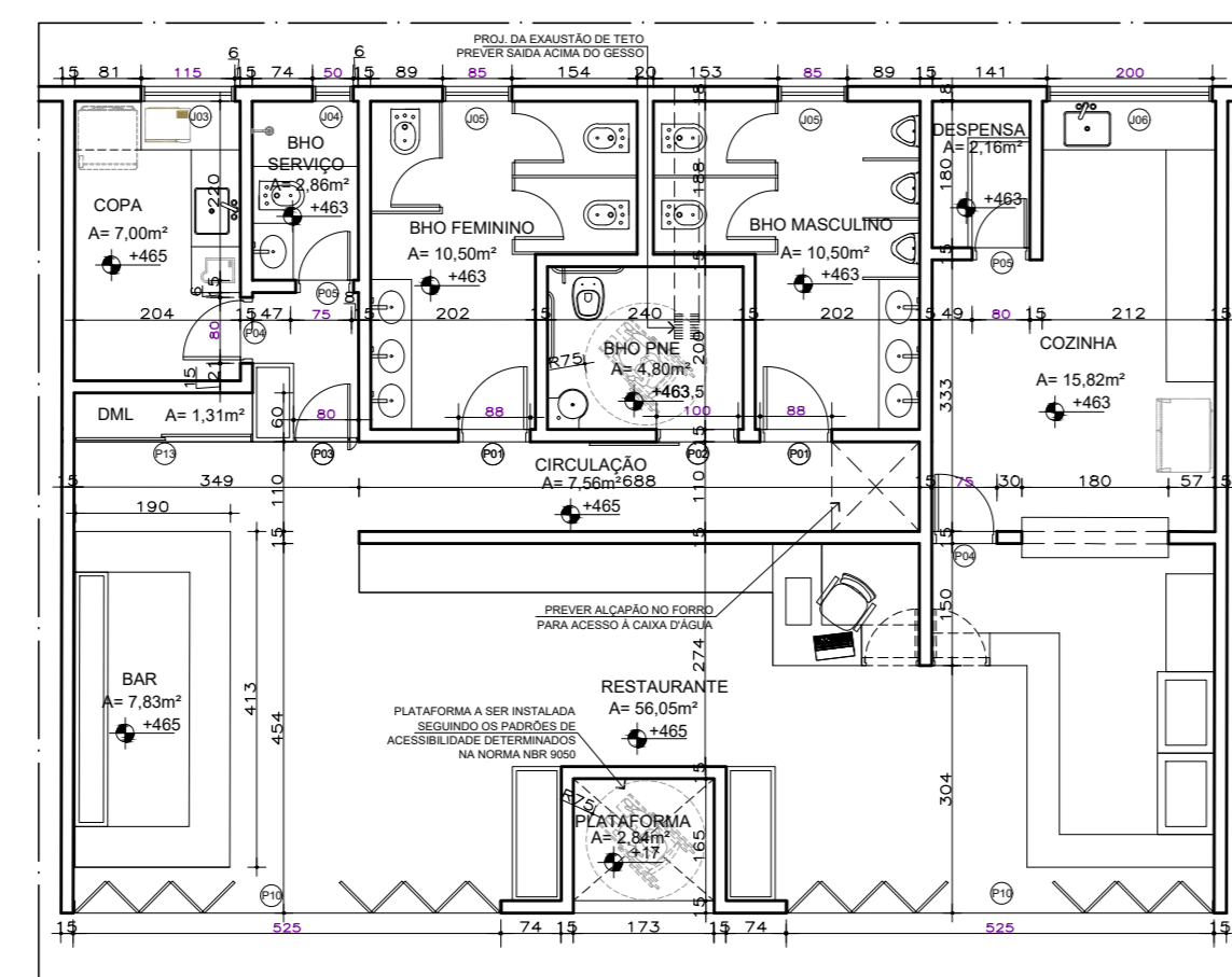
PLANTA LAYOUT TIPO (RESTAURANTES) ESC. 1:100
