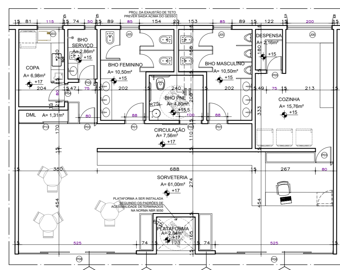
PLANTA LAYOUT TIPO (SORVETERIA) ESC. 1:100
