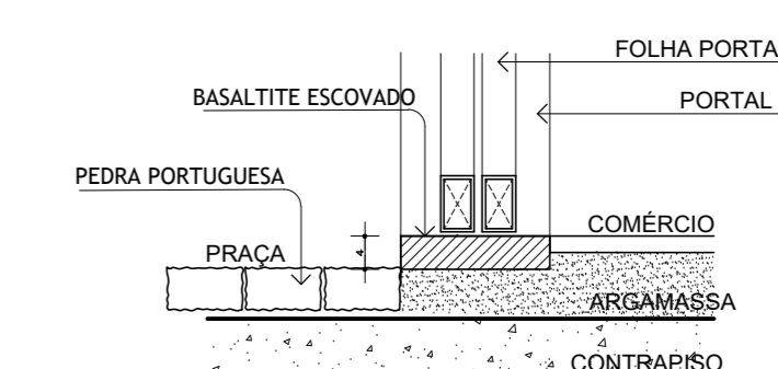
03 DET. DESNÍVEL PISO
