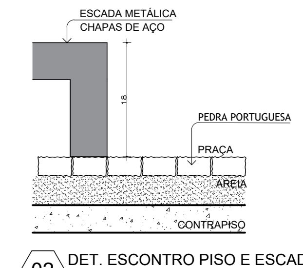
02 DET. ENCONTRO PISO E ESCADA
