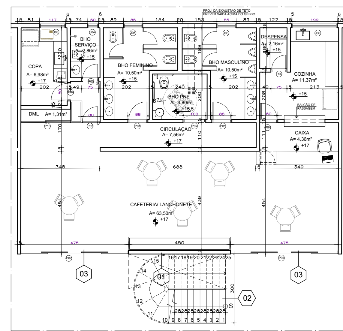
PLANTA LAYOUT TIPO (CAFETERIA/LANCHONETE) ESC. 1:100
