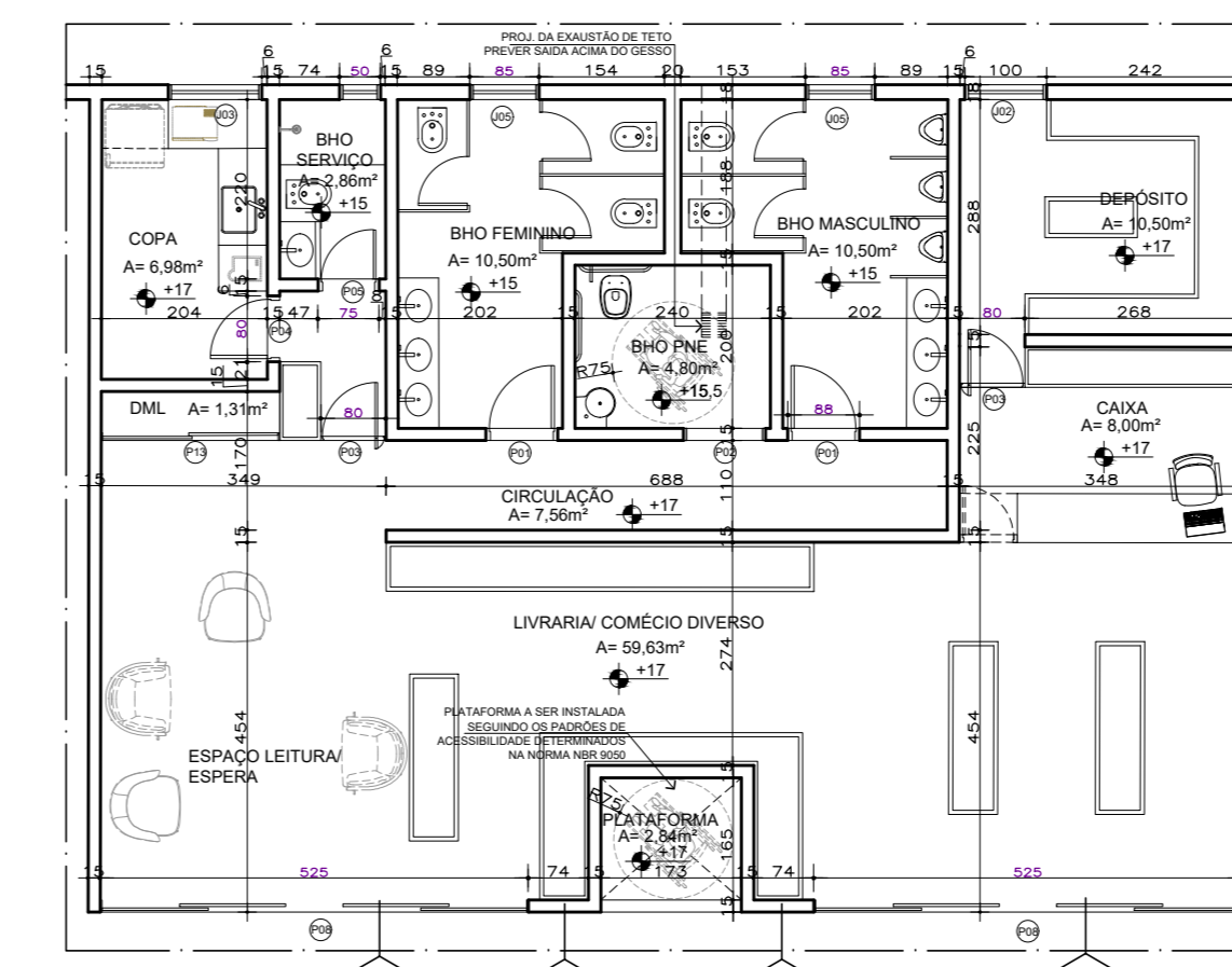
PLANTA LAYOUT TIPO (COMÉRCIO DIVERSO) ESC. 1:100
