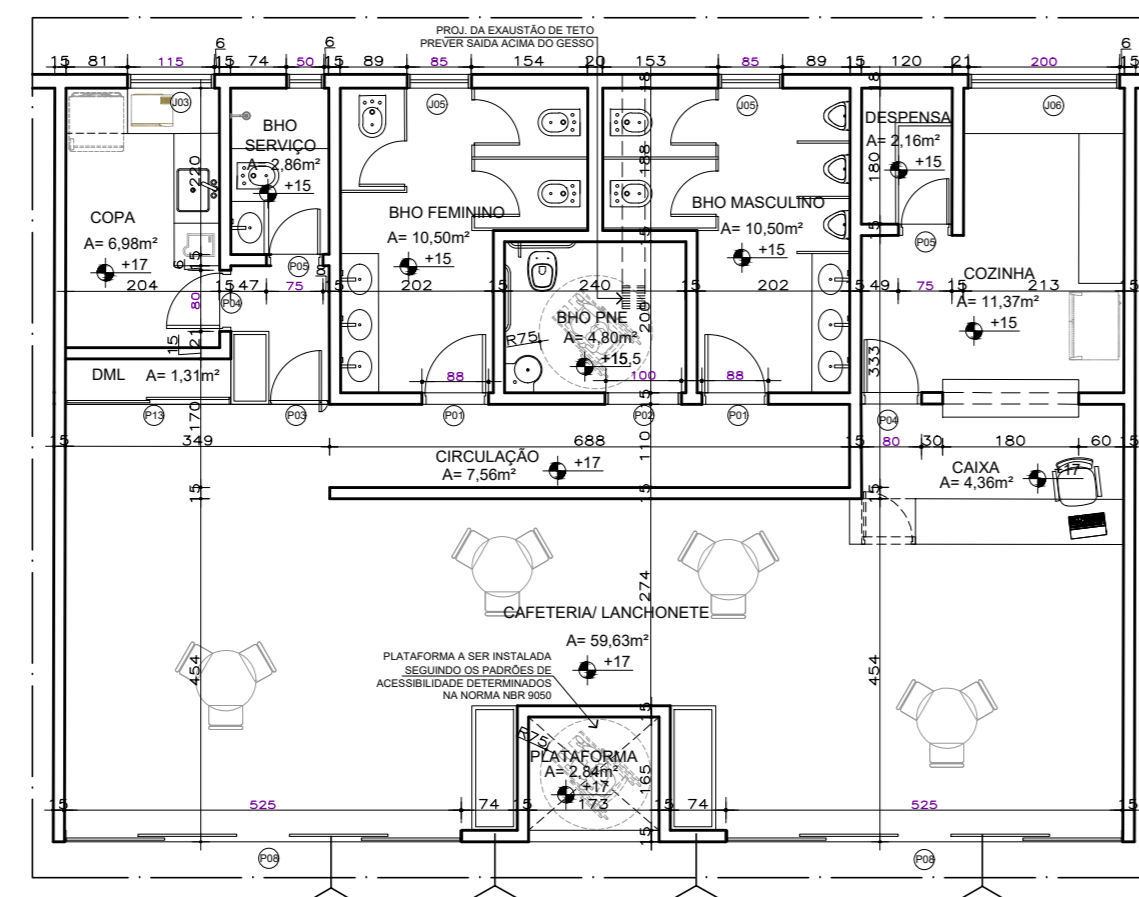
PLANTA LAYOUT TIPO (CAFETERIA/LANCHONETE) ESC. 1:100
