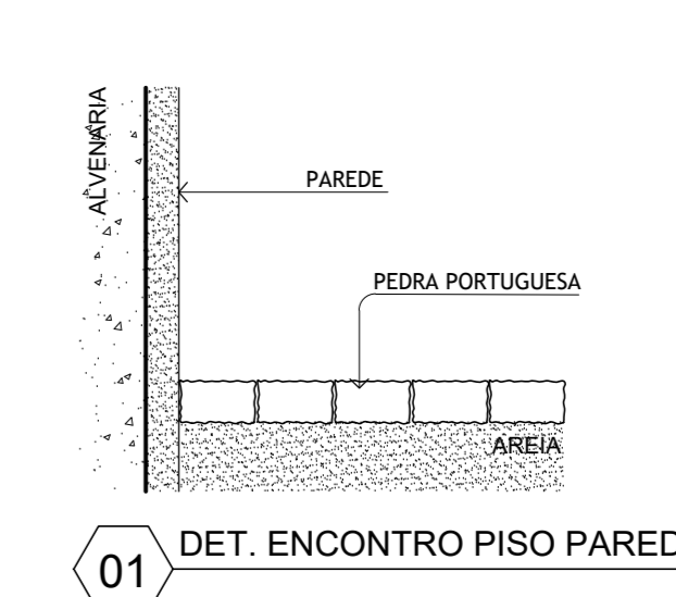
01 DET. ENCONTRO PISO PAREDE
