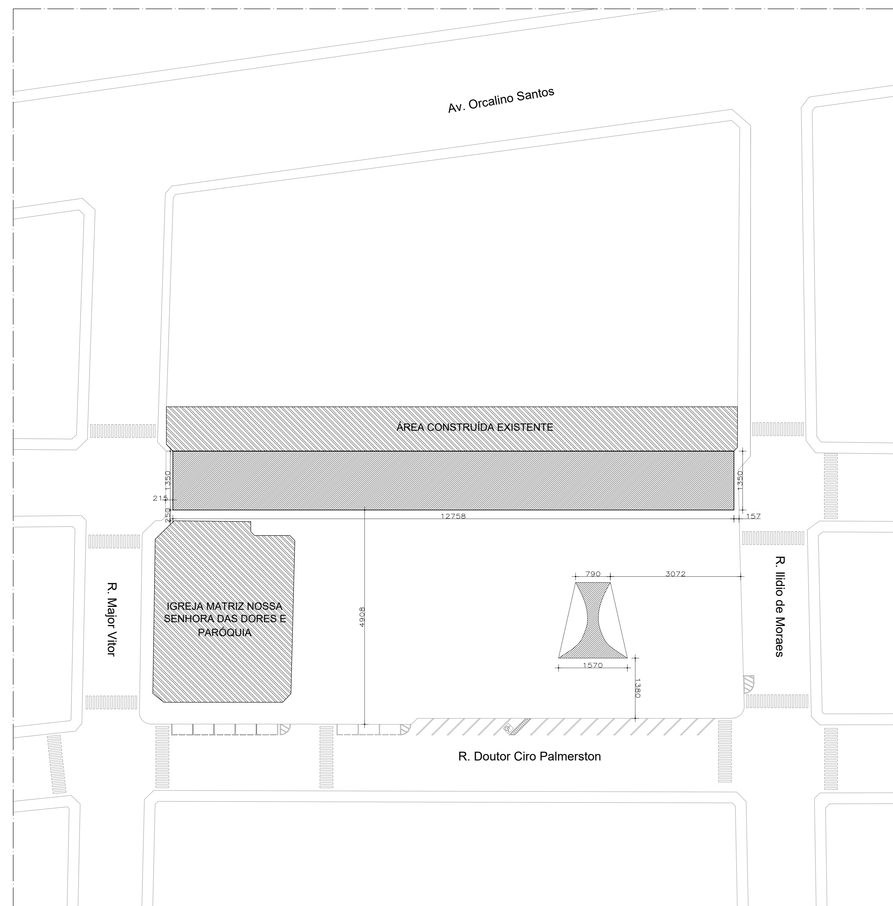
PLANTA DE LOCAÇÃO: COBERTURA DOS RESTAURANTES E ESPELHO D'ÁGUA ESC. 1:500
