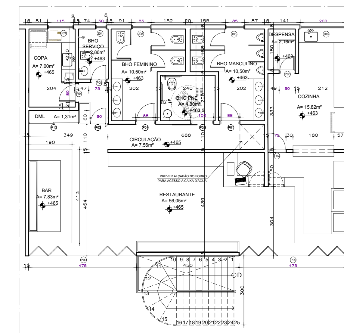
PLANTA LAYOUT TIPO (RESTAURANTES) ESC. 1:100
