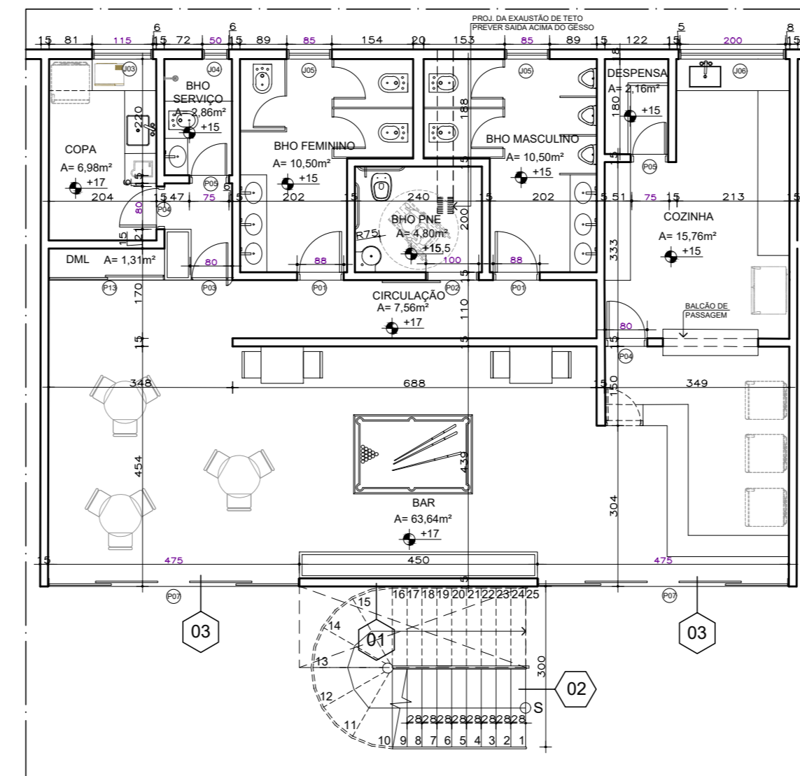
PLANTA LAYOUT TIPO (BAR) ESC. 1:100
