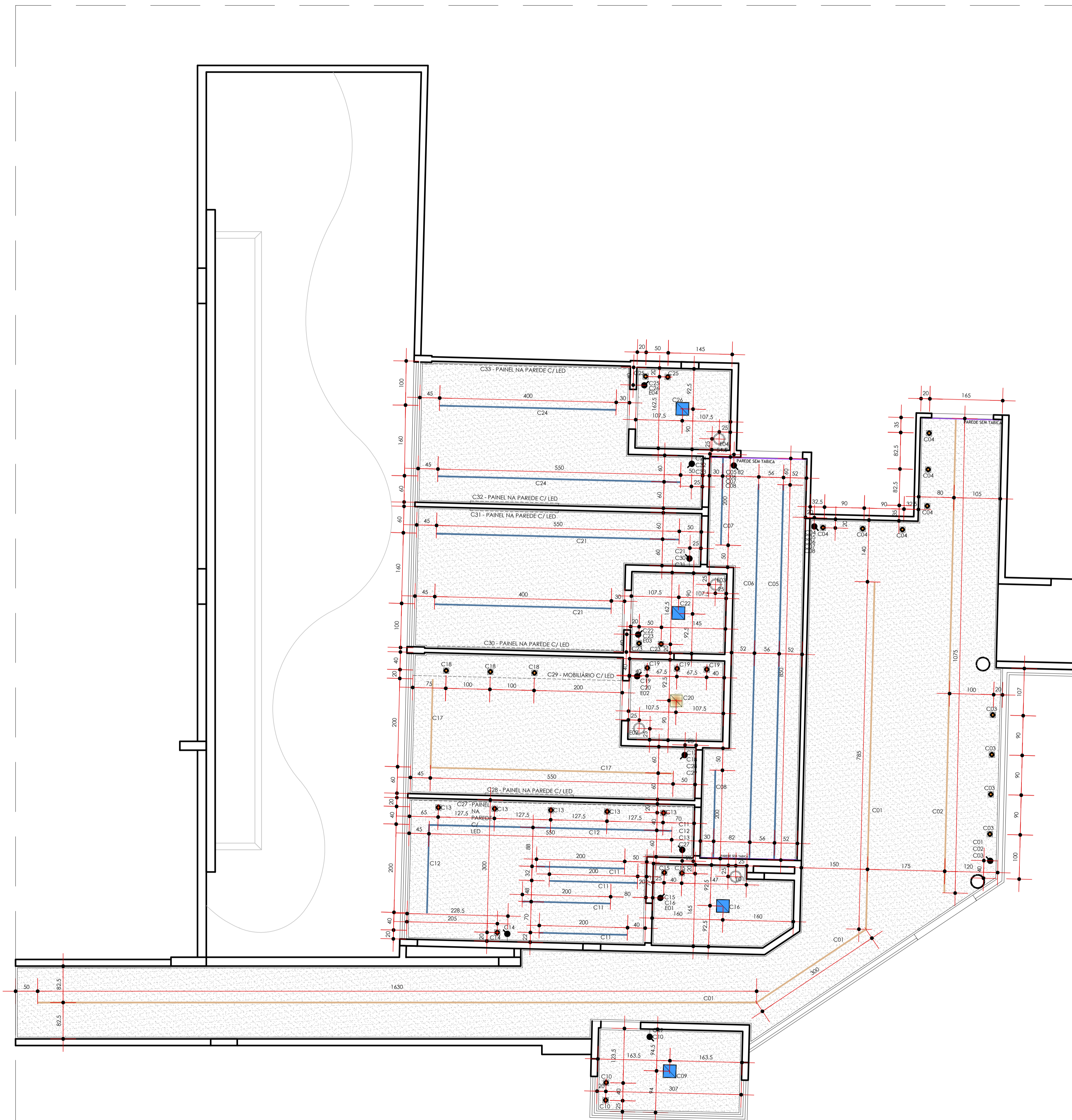
PLANTA LUMINOTÉCNICO - ALA PEDIATRIA ESCALA: 1:50
