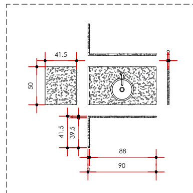
DET. BANCADA ESCALA 1:50
