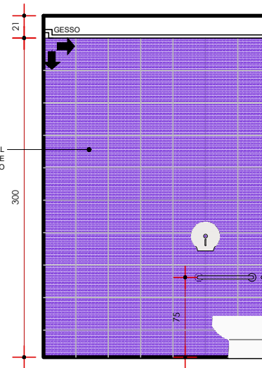
VISTA 03 ESCALA 1:50
