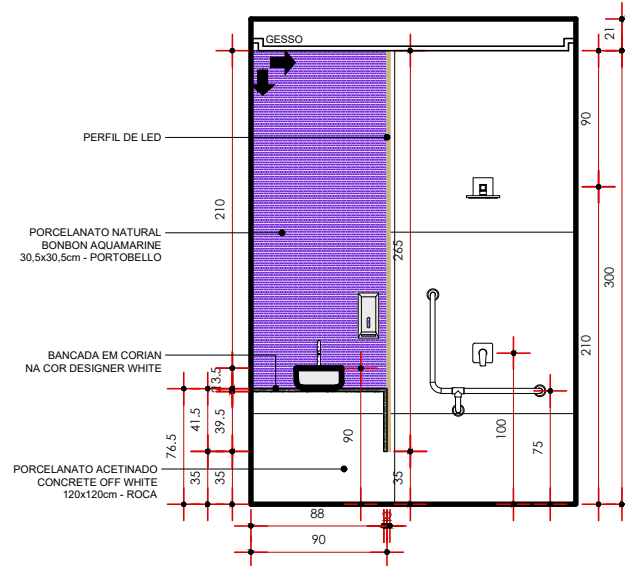
VISTA 01 ESCALA 1:50
