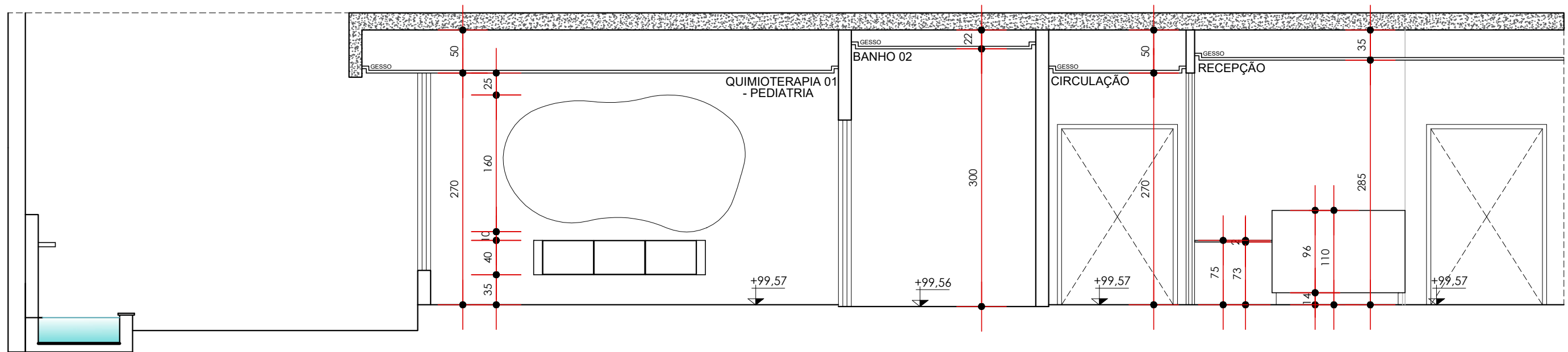
CORTE BB ESCALA 1:50
