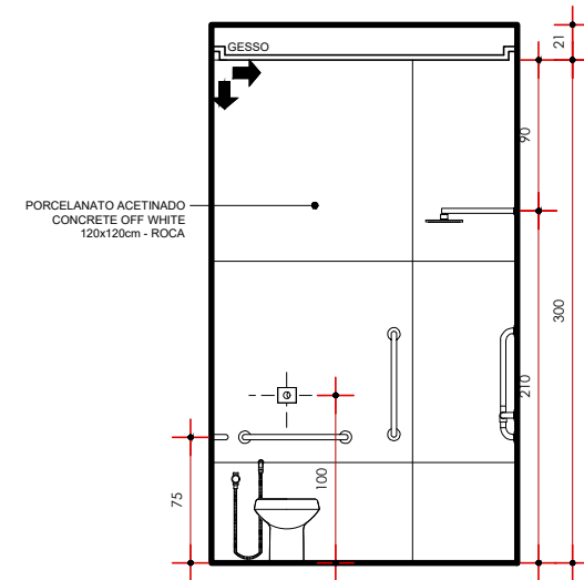
VISTA 04 ESCALA 1:50
