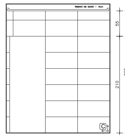
VISTA 12 - LAVANDERIA ESC. 1:50
