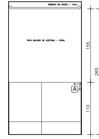
VISTA 5 - BANHEIRO I ESC. 1:50
