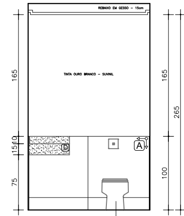
VISTA 7 - BANHEIRO II ESC. 1:50
