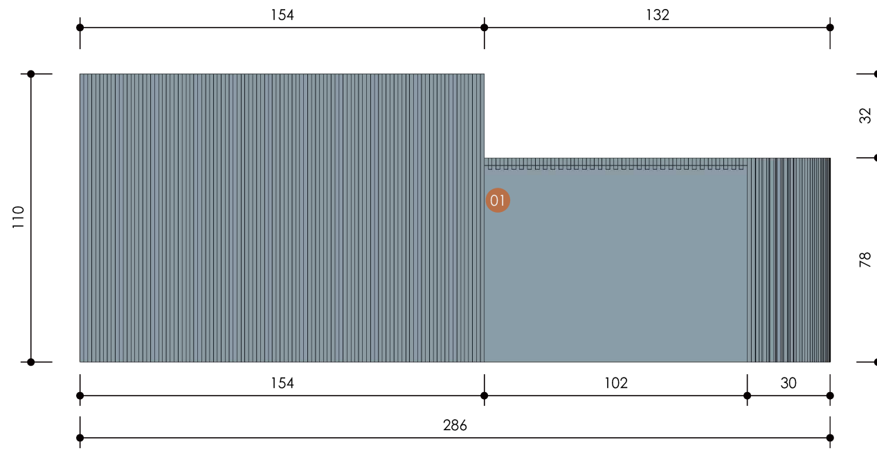
DETALHAMENTO - FRENTE ESC.: 1/20
