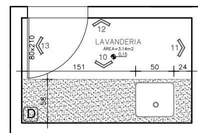
PLANTA - LAVANDERIA ESC. 1:50
