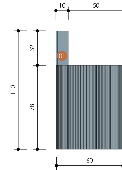
DETALHAMENTO - DIREITA ESC.: 1/25
