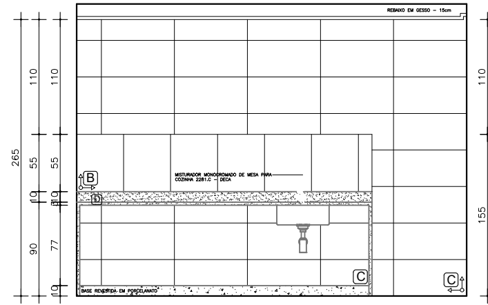
VISTA 1 - COZINHA ESC. 1:50
