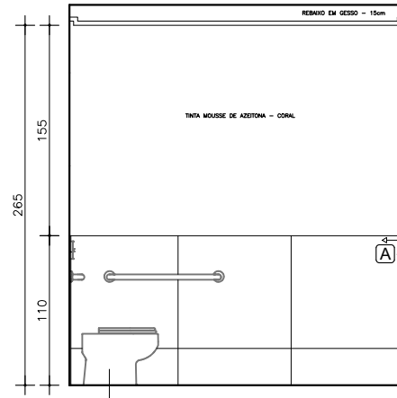
VISTA 2 - BANHEIRO I ESC. 1:50
