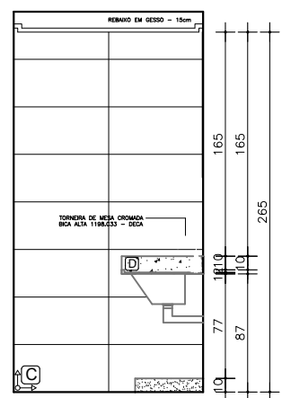
VISTA 11 - LAVANDERIA ESC. 1:50
