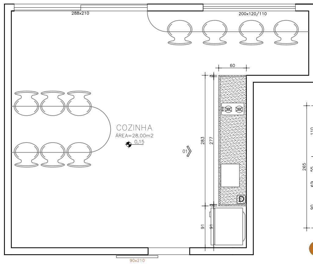
PLANTA - COZINHA ESC. 1:50
