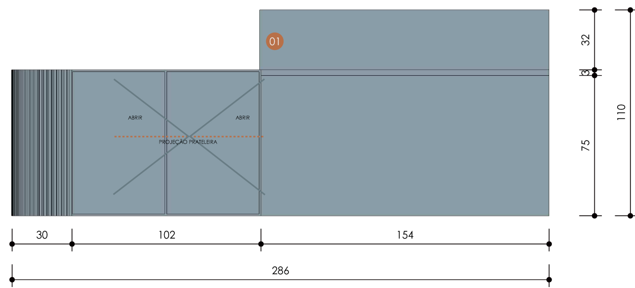
DETALHAMENTO - FUNDO ESC.: 1/20
