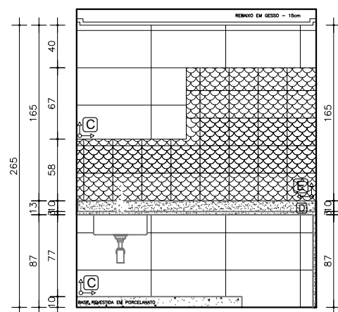
VISTA 10 - LAVANDERIA ESC. 1:50
