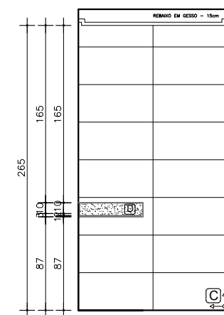
VISTA 13 - LAVANDERIA ESC. 1:50
