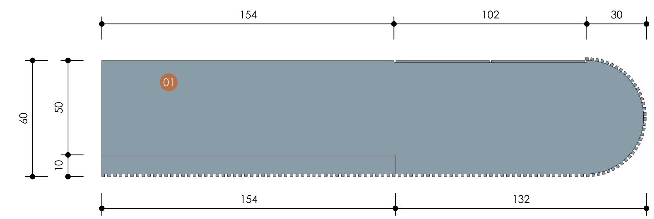
DETALHAMENTO - SUPERIOR ESC.: 1/20
