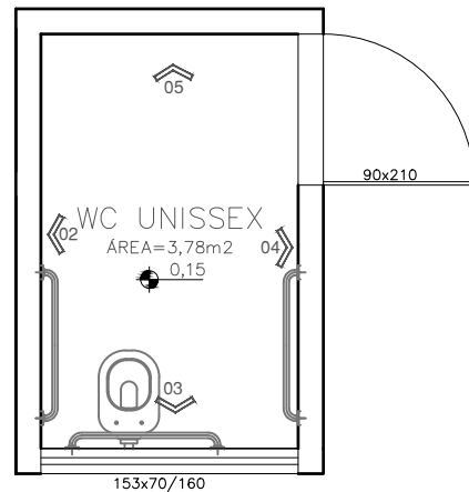
PLANTA - BANHEIRO I ESC. 1:50
