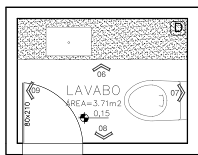
PLANTA - BANHEIRO II ESC. 1:50
