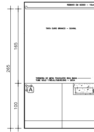
VISTA 9 - BANHEIRO II ESC. 1:50
