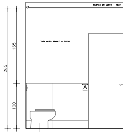
VISTA 8 - BANHEIRO II ESC. 1:50
