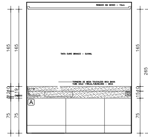
VISTA 6 - BANHEIRO II ESC. 1:50
