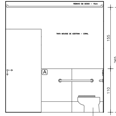
VISTA 4 - BANHEIRO I ESC. 1:50
