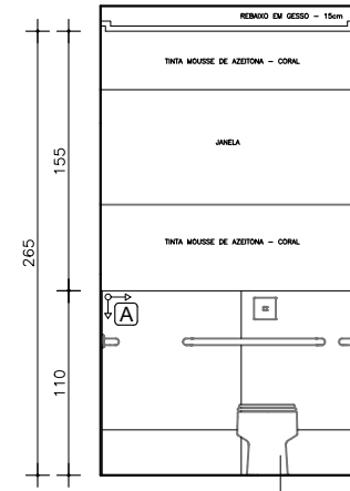
VISTA 3 - BANHEIRO I ESC. 1:50
