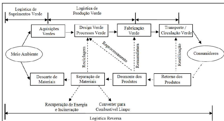
Figura 1: Diagrama do Sistema de Green Logistic
