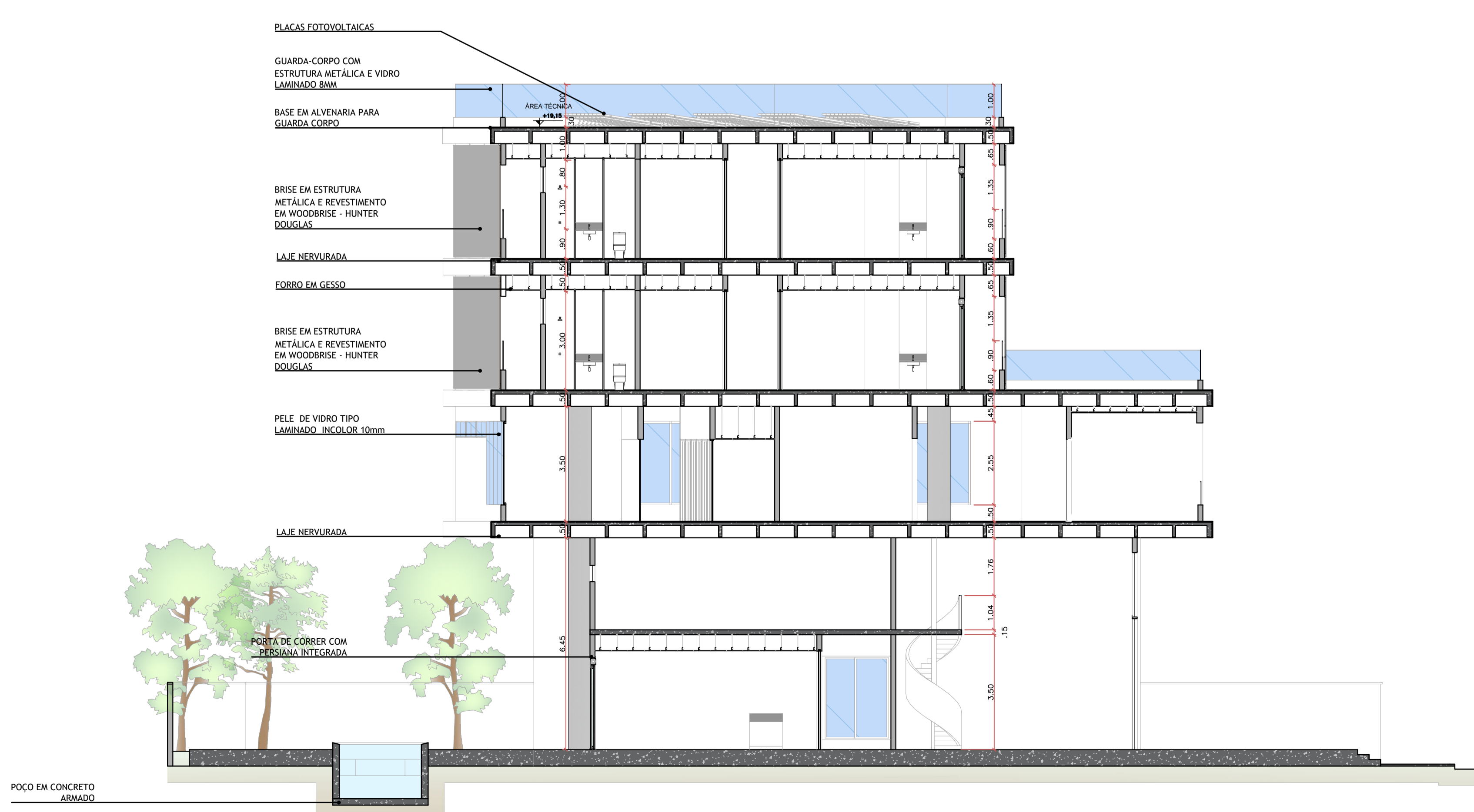
CORTE CC ESC 1:100
