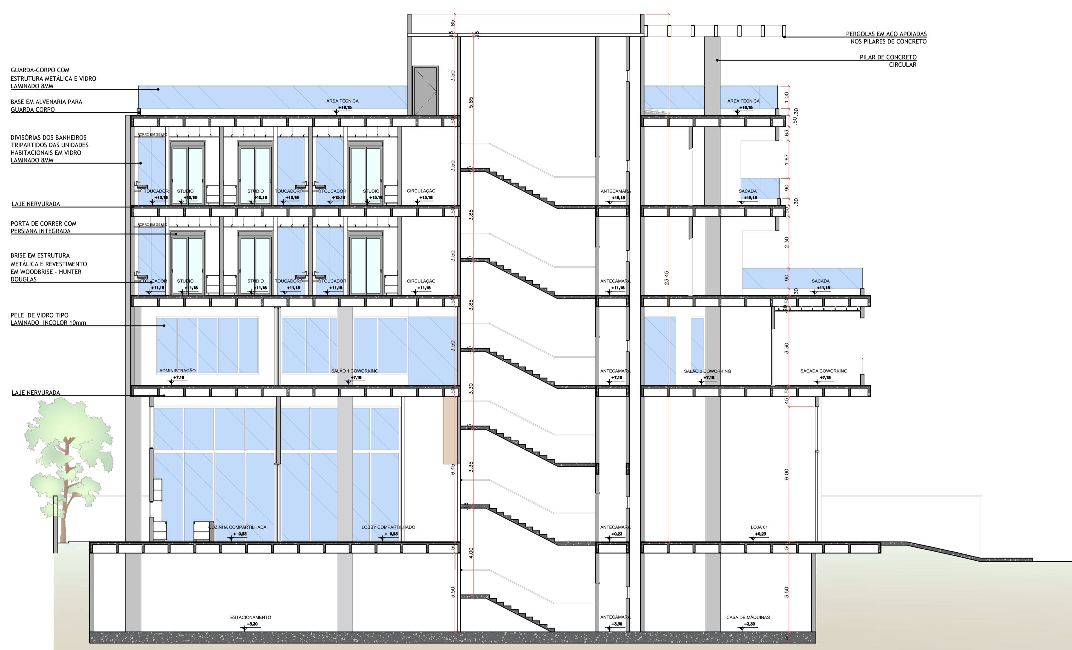
CORTE BB ESC 1:100
