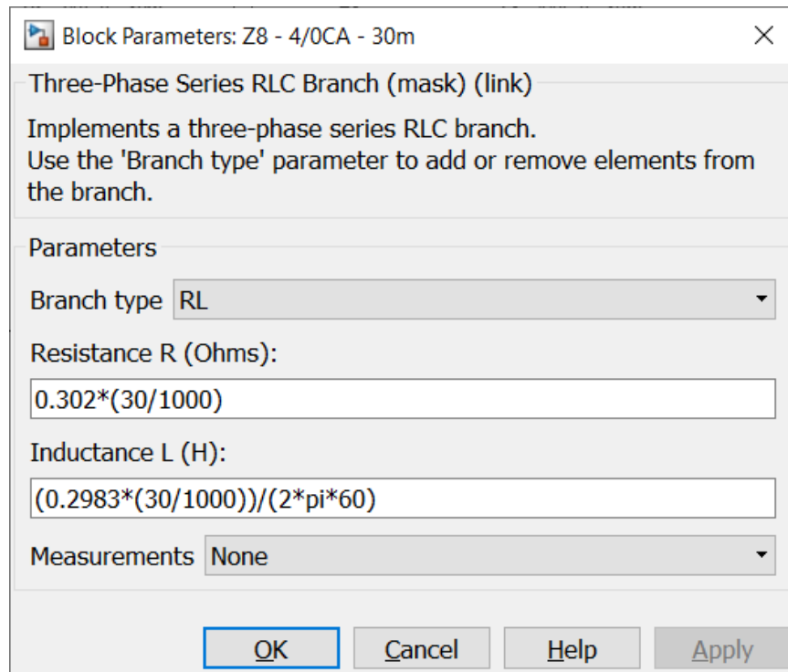
Figura 14 – Parâmetros do cabo 4/0CA.
